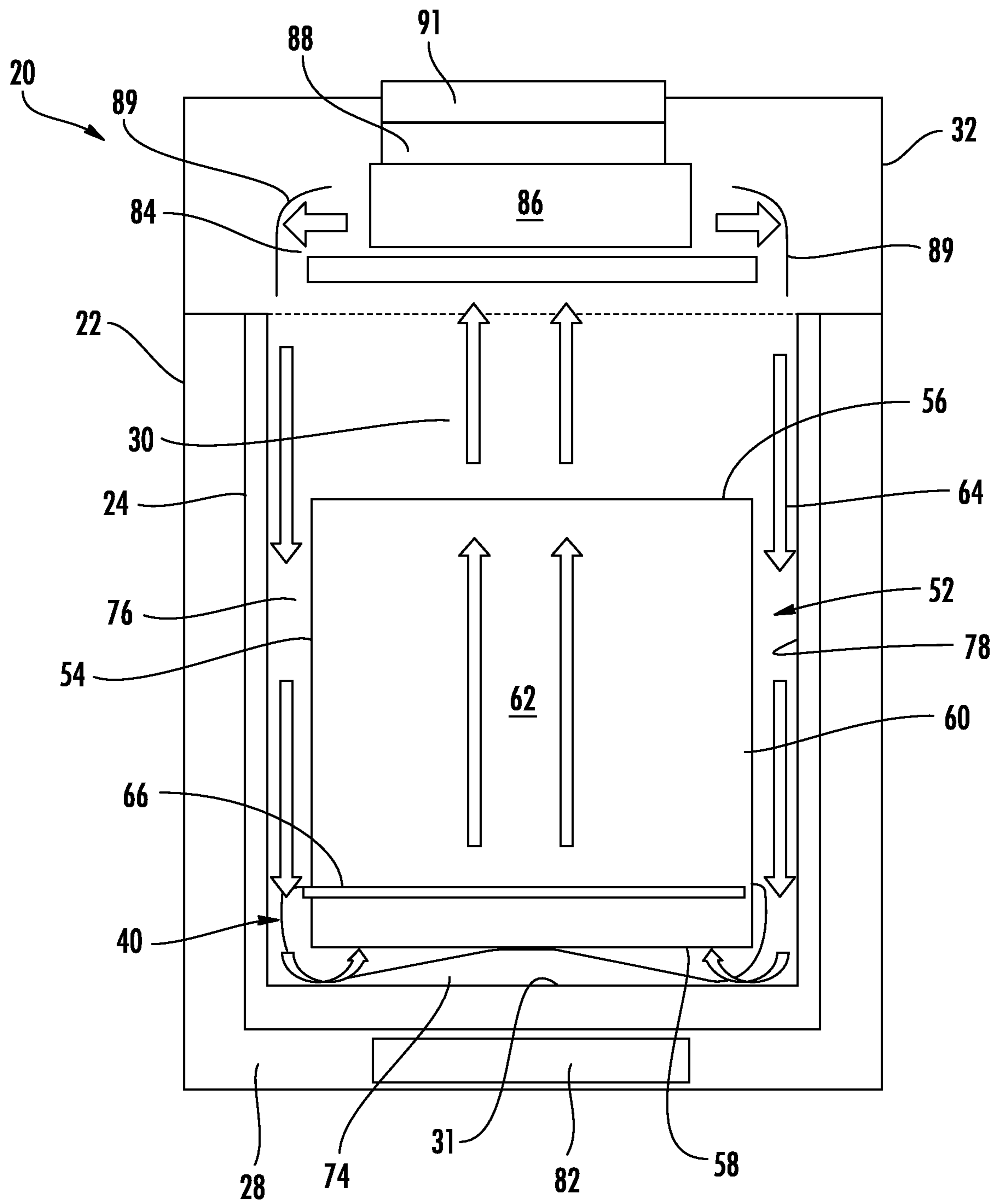
FIG. 7
