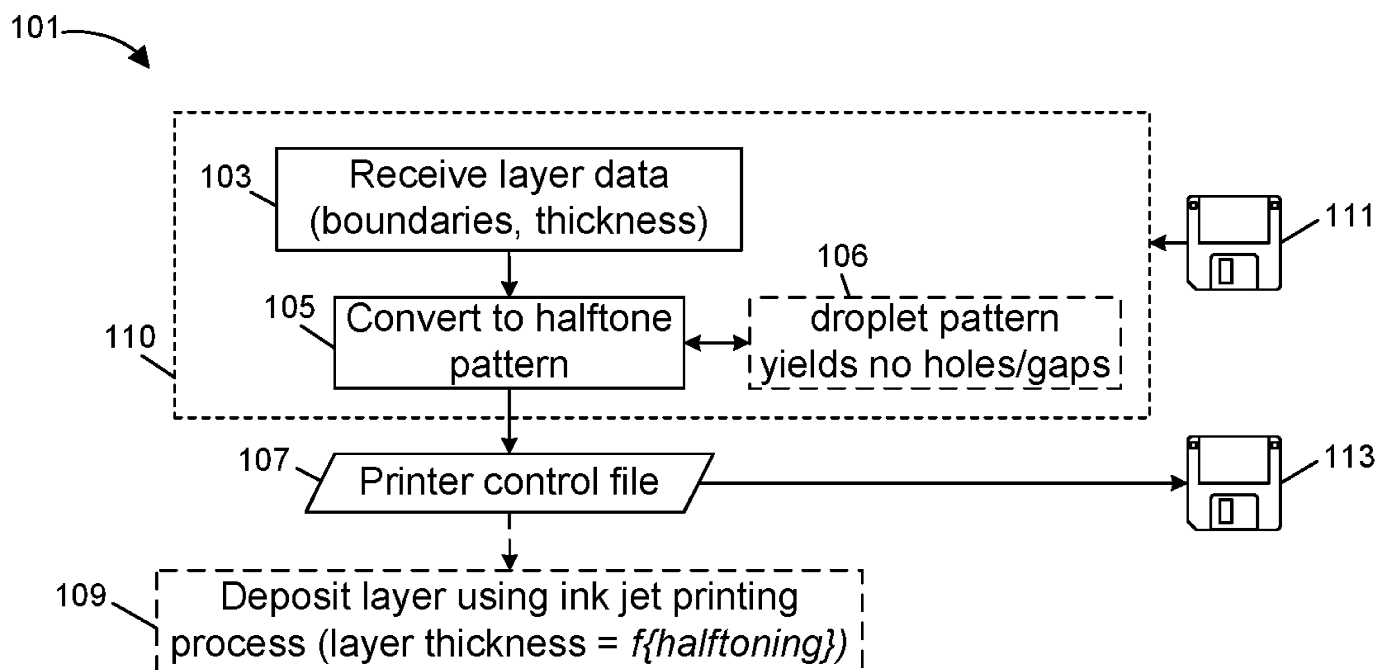
FIG. 1A
