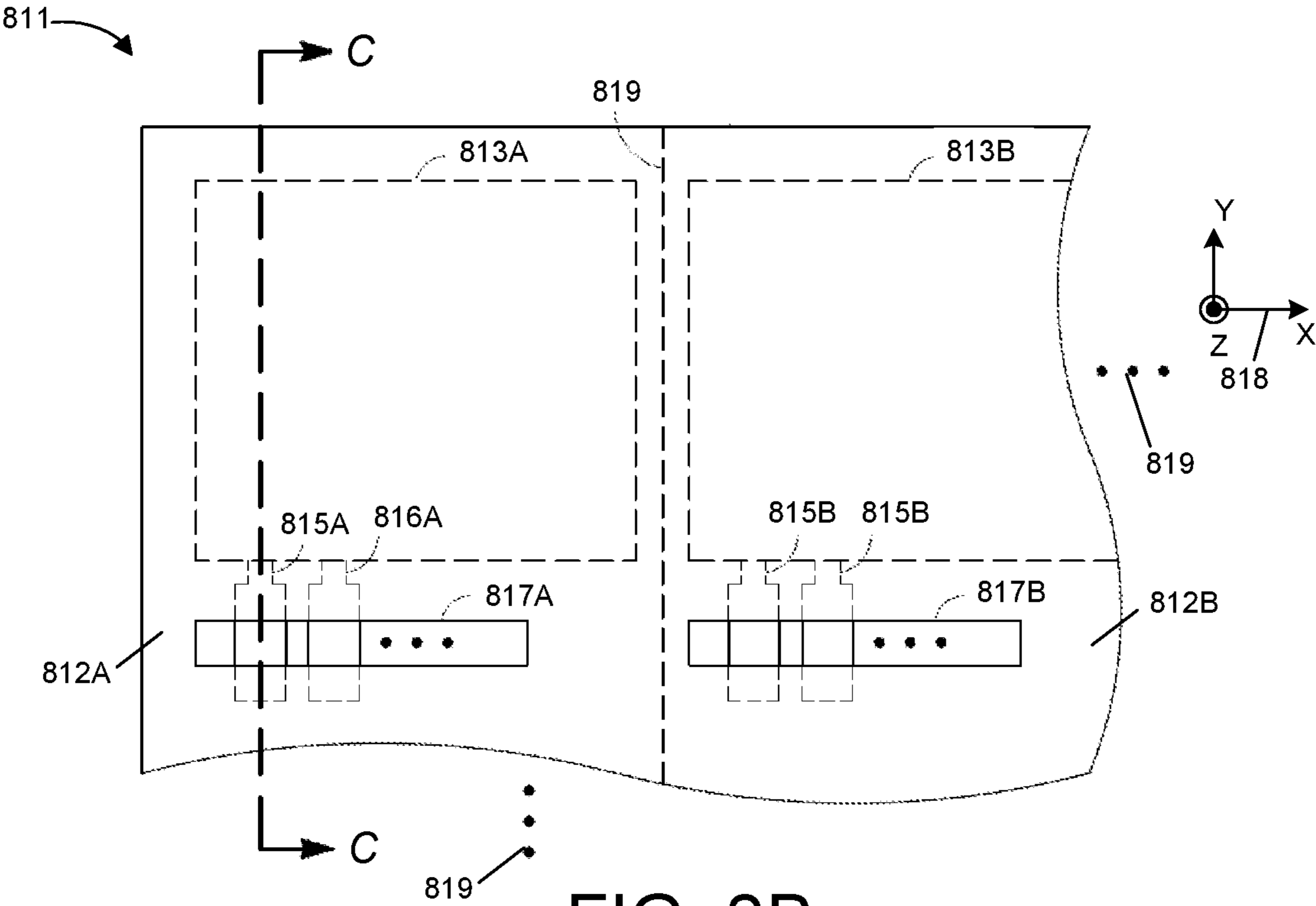
FIG. 8B
