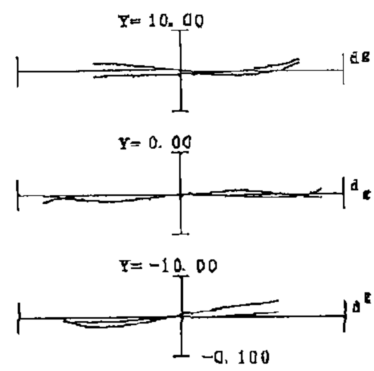
COMA ABERRATION
