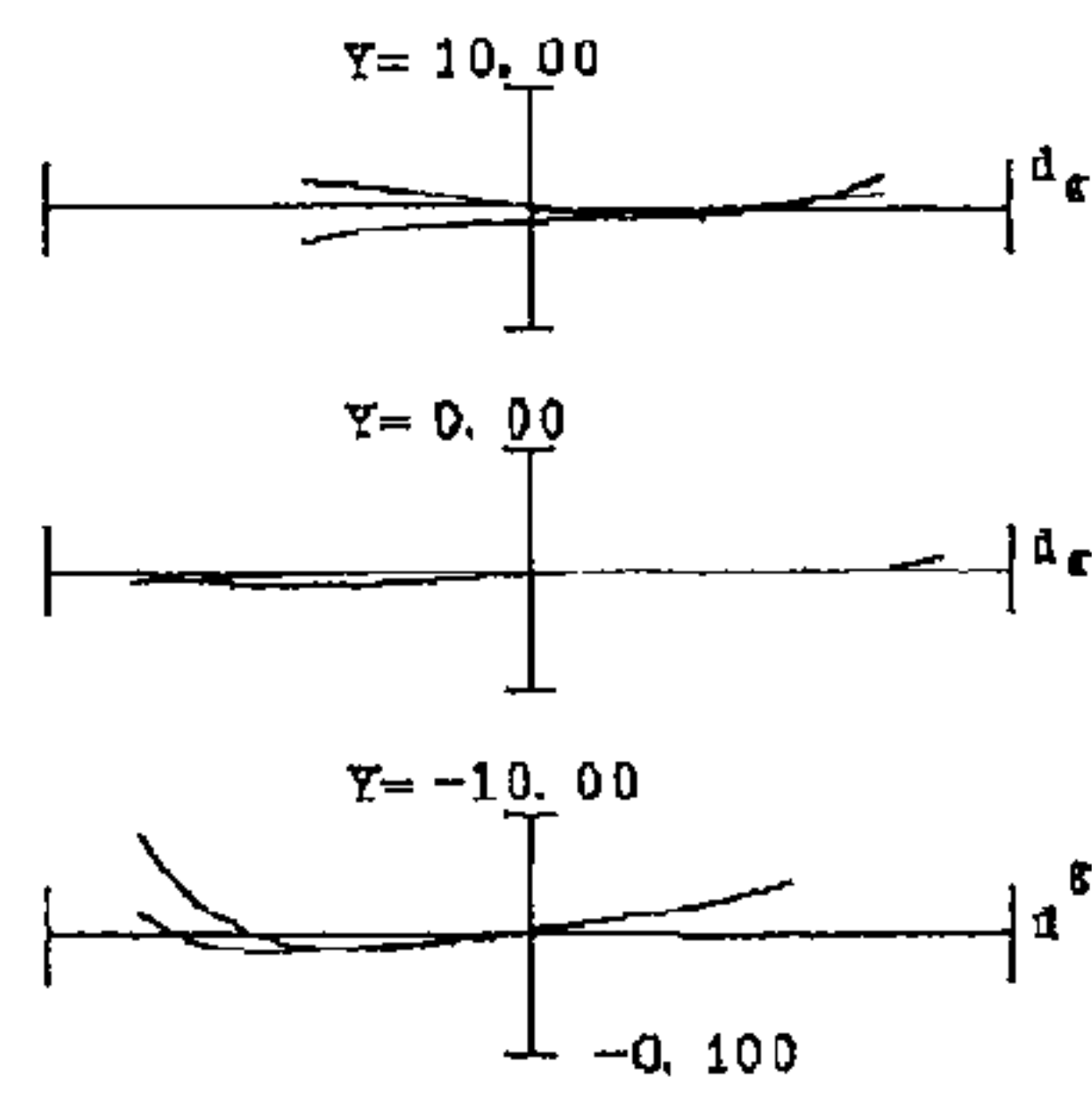
COMA ABERRATION
