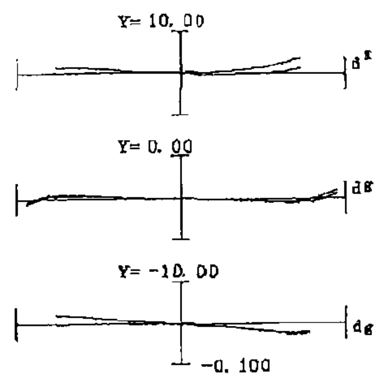
COMA ABERRATION
