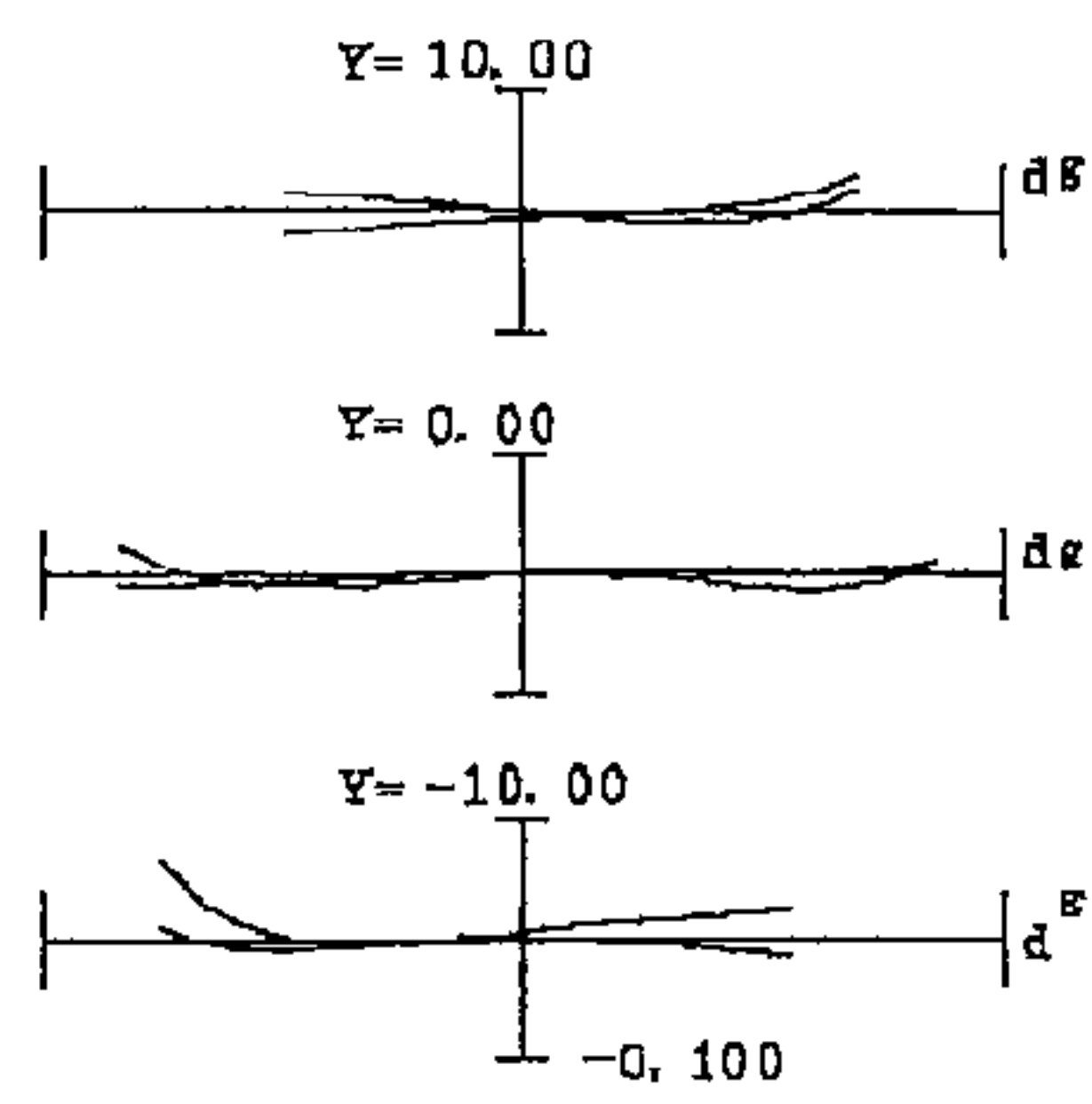
COMA ABERRATION
