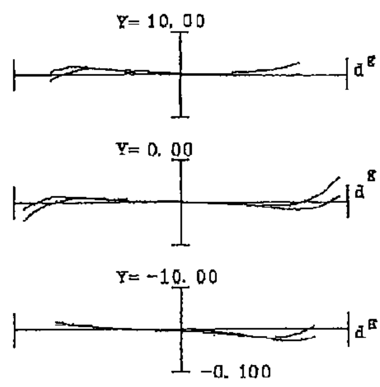
COMA ABERRATION
