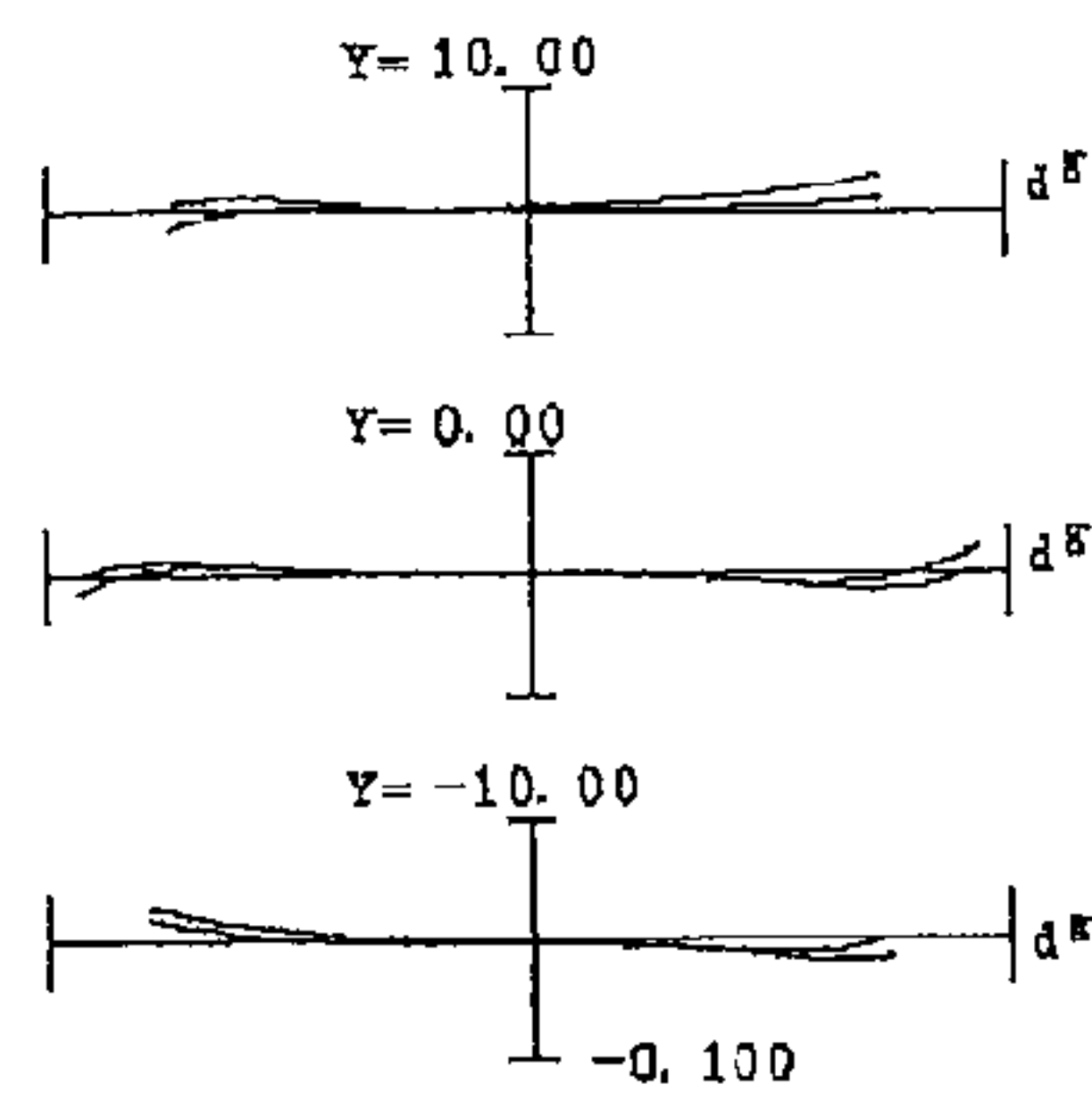
COMA ABERRATION
