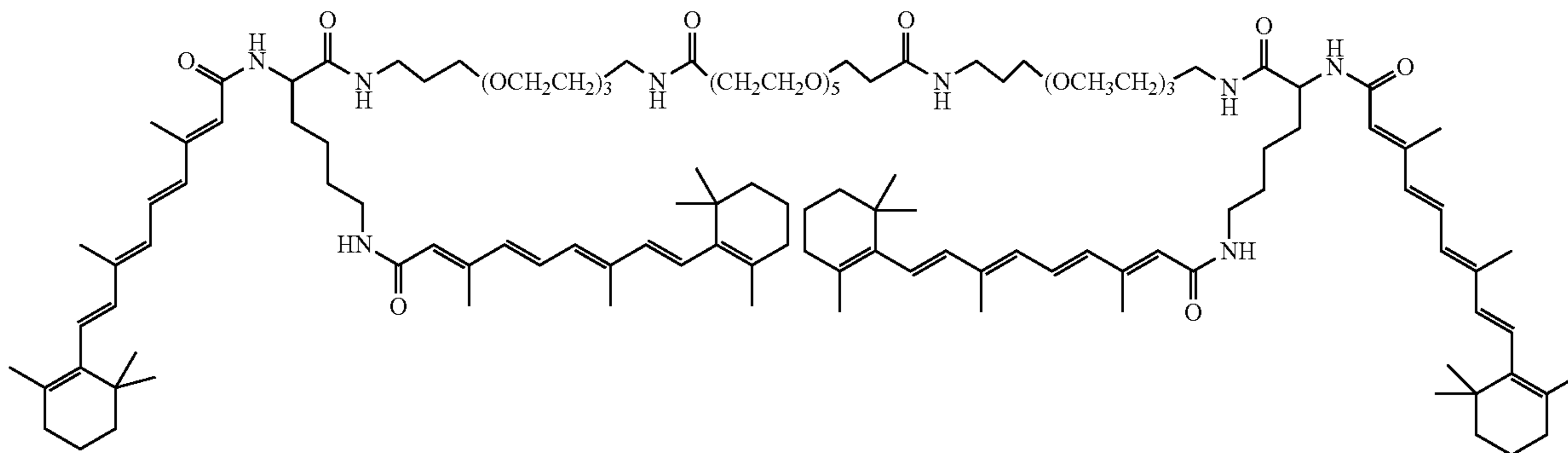
DiVA-PEG-DiVA
