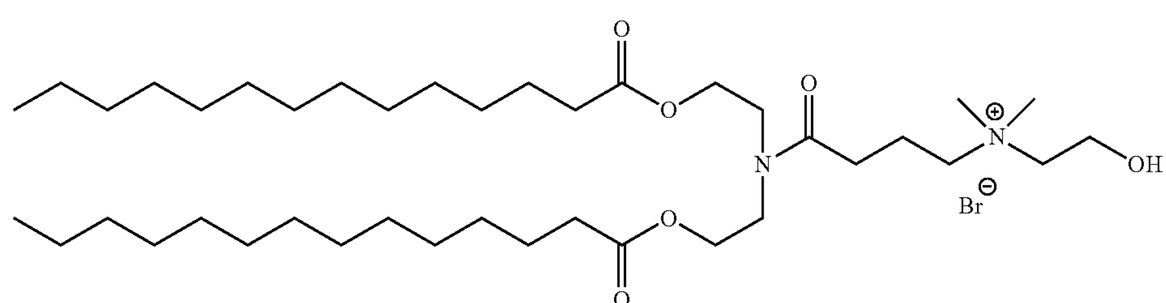
HE-Pr-DC
