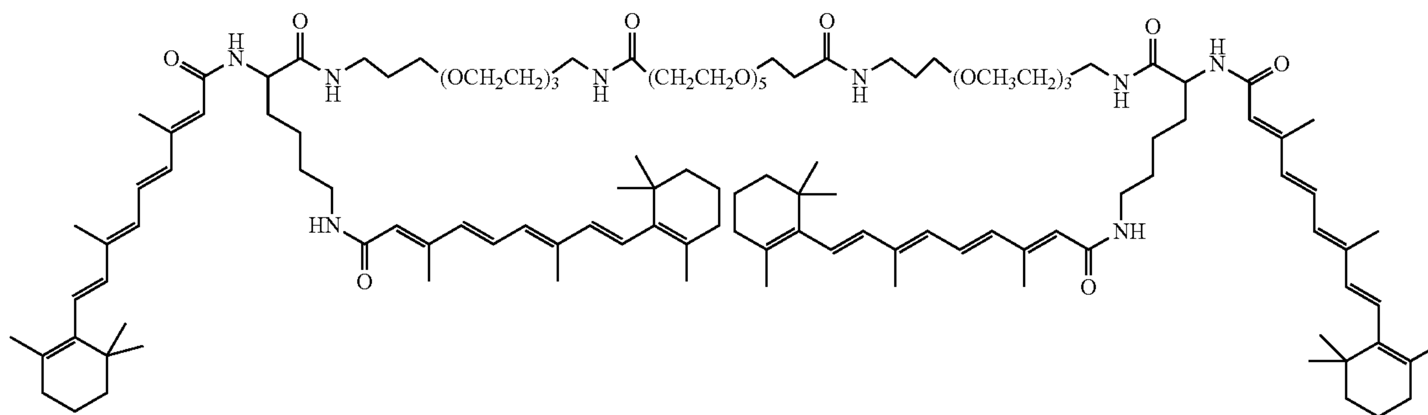
DiVA-PEG-DiVA
