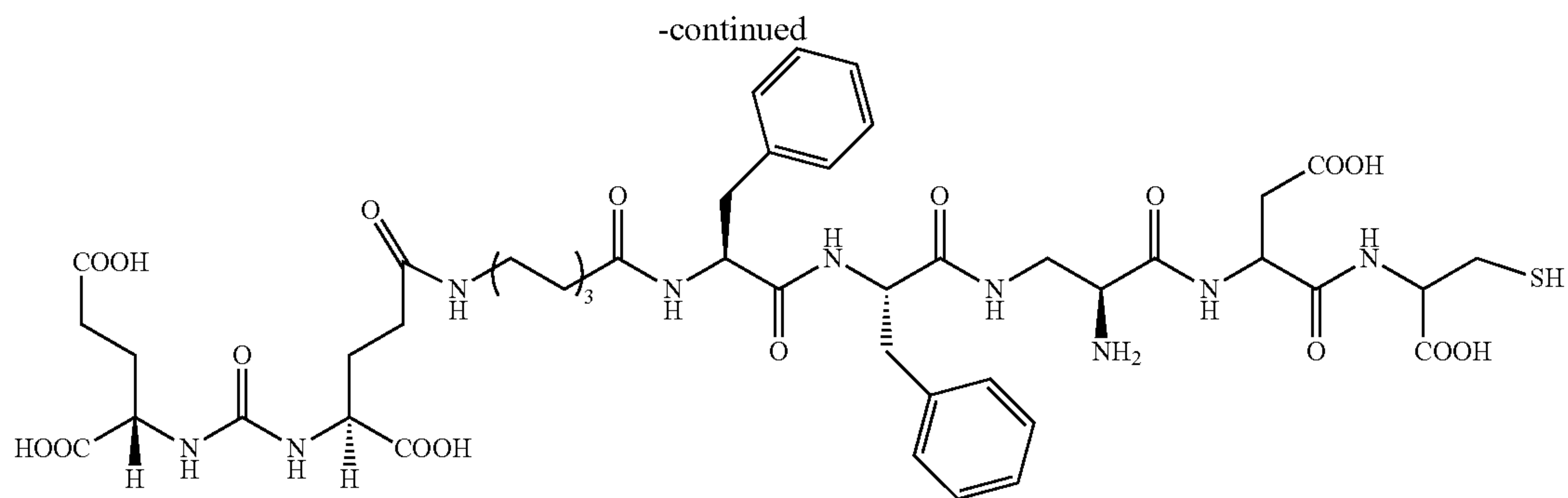
PC01SK28 C 47 H 65 N 9 O 17 S Mol. Wt.: 1060.13
