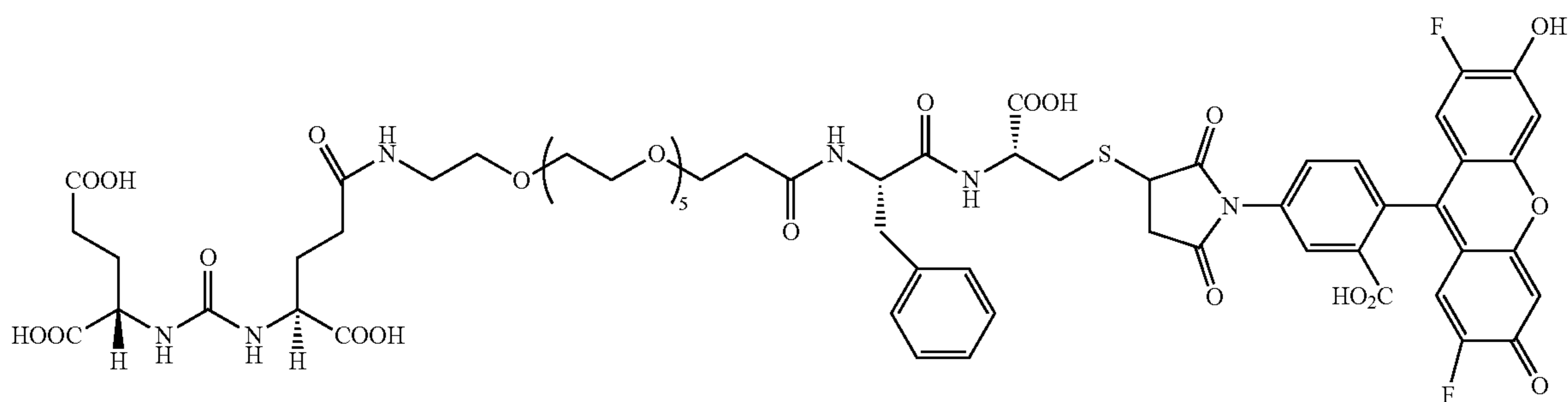
PC01SK56 C_{62}H_{70}F_2N_5O_{25}S Mol. Wt.: 1369.31
