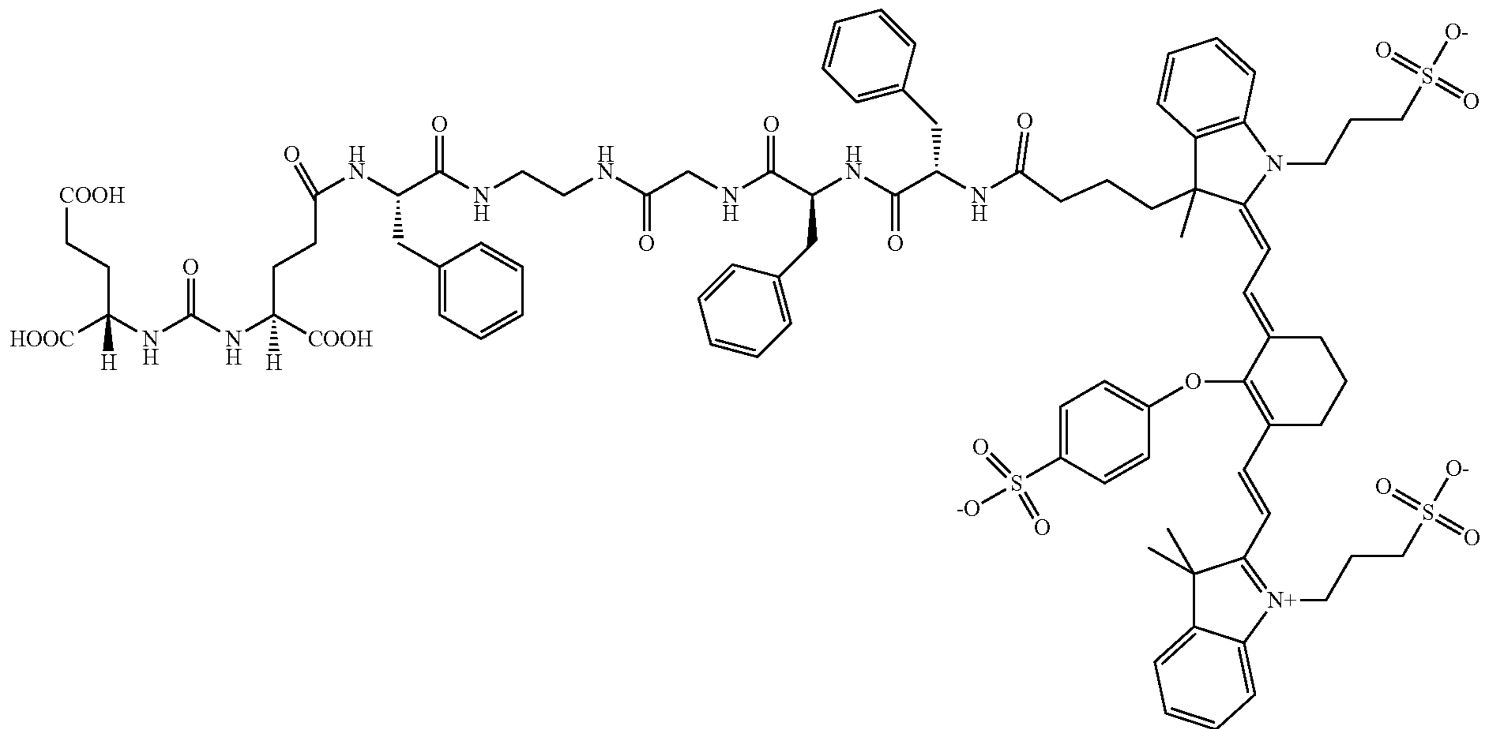
DyLight 800 conjugate
