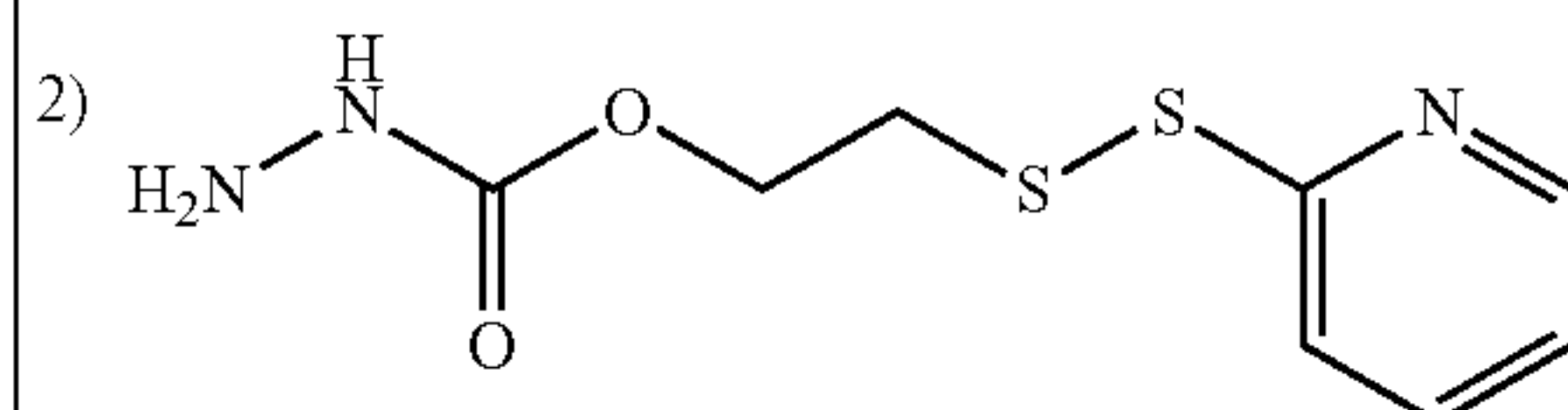
EC0311 C 8 H 11 N 3 O 2 S 2 Mol. Wt.: 245.32
