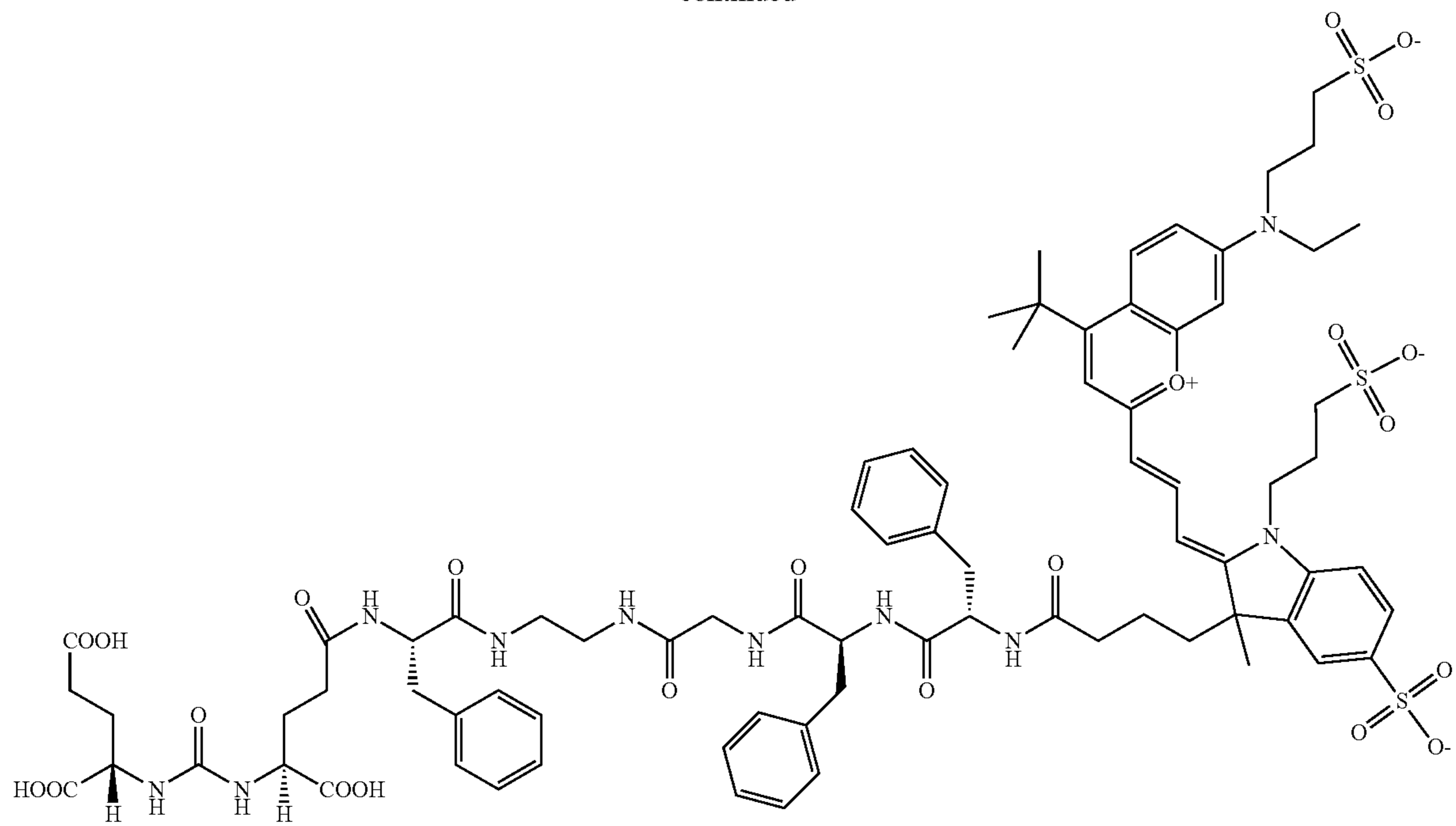
DyLight 680 conjugate
