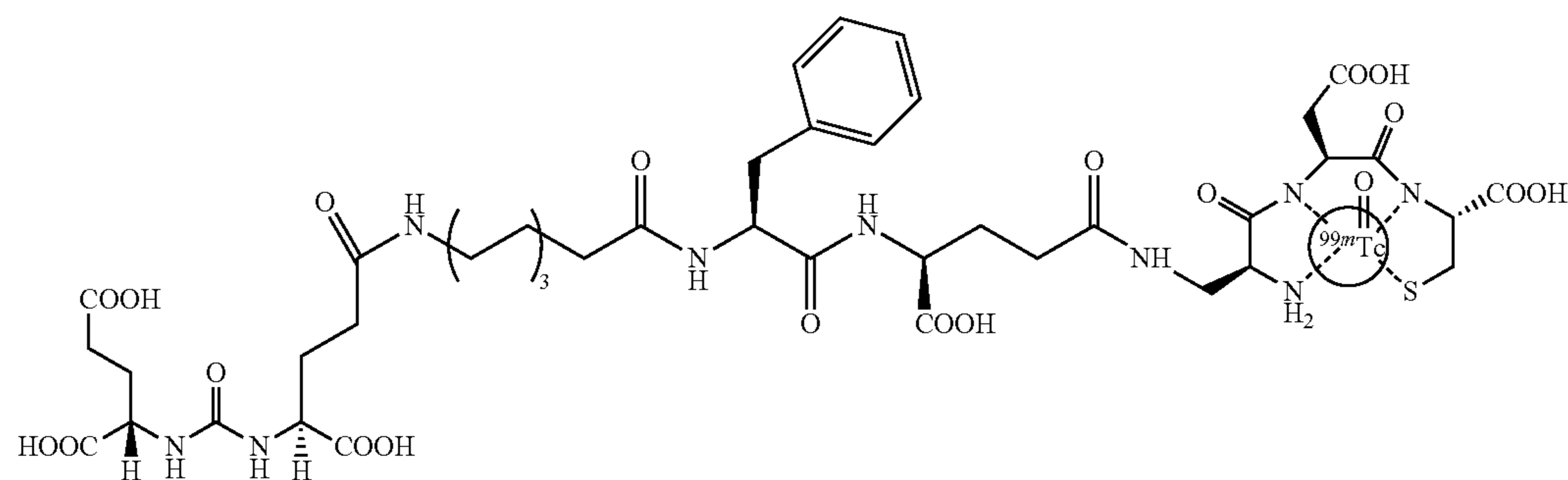
SK38- 99m Tc (16-atom linker, 1.4 mg)
