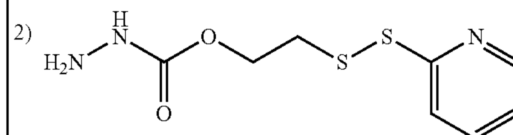
EC0311 C 9 H 11 N 3 O 2 S 2 Mol. Wt.: 245.32
