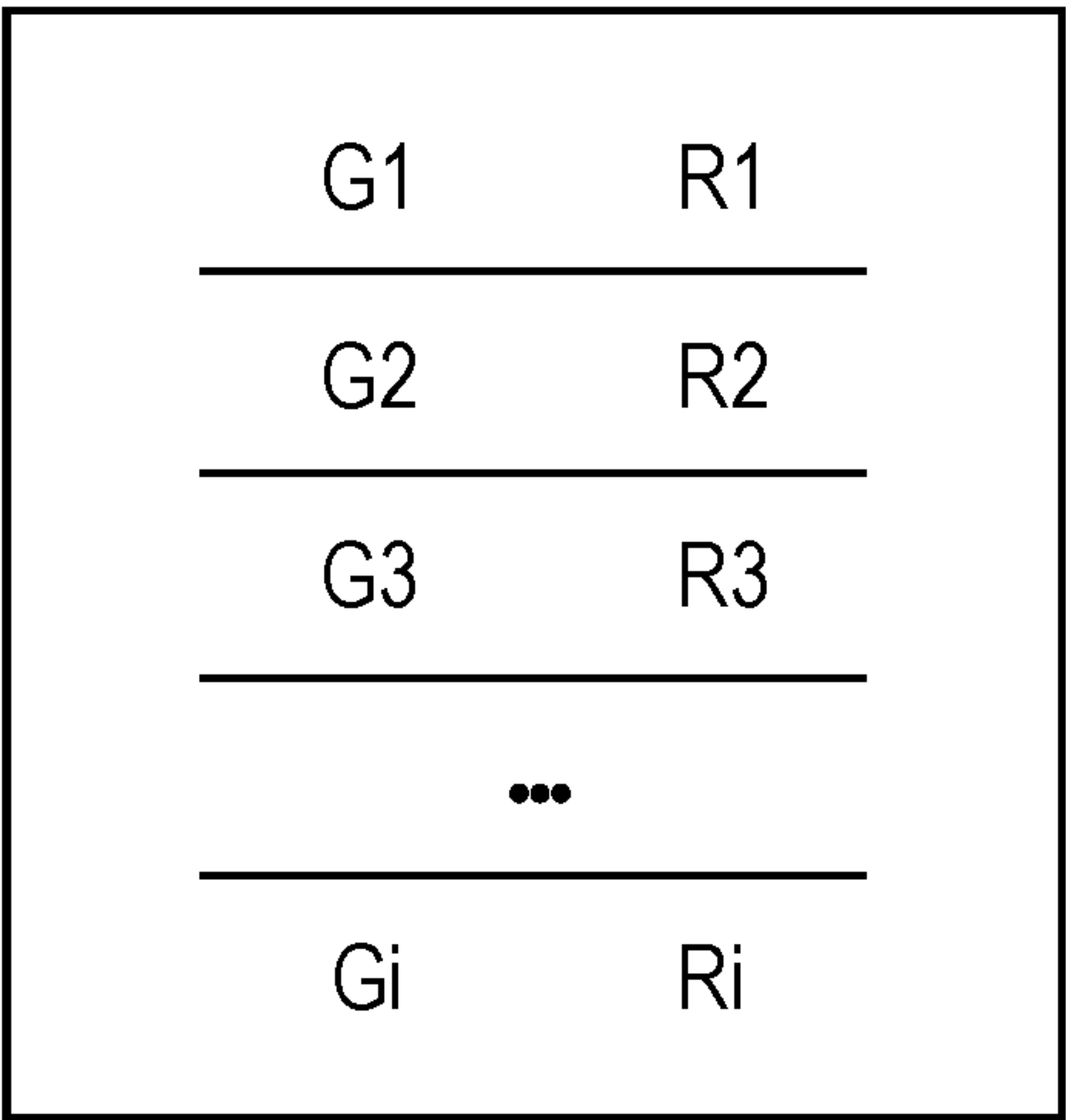
Resistor string
