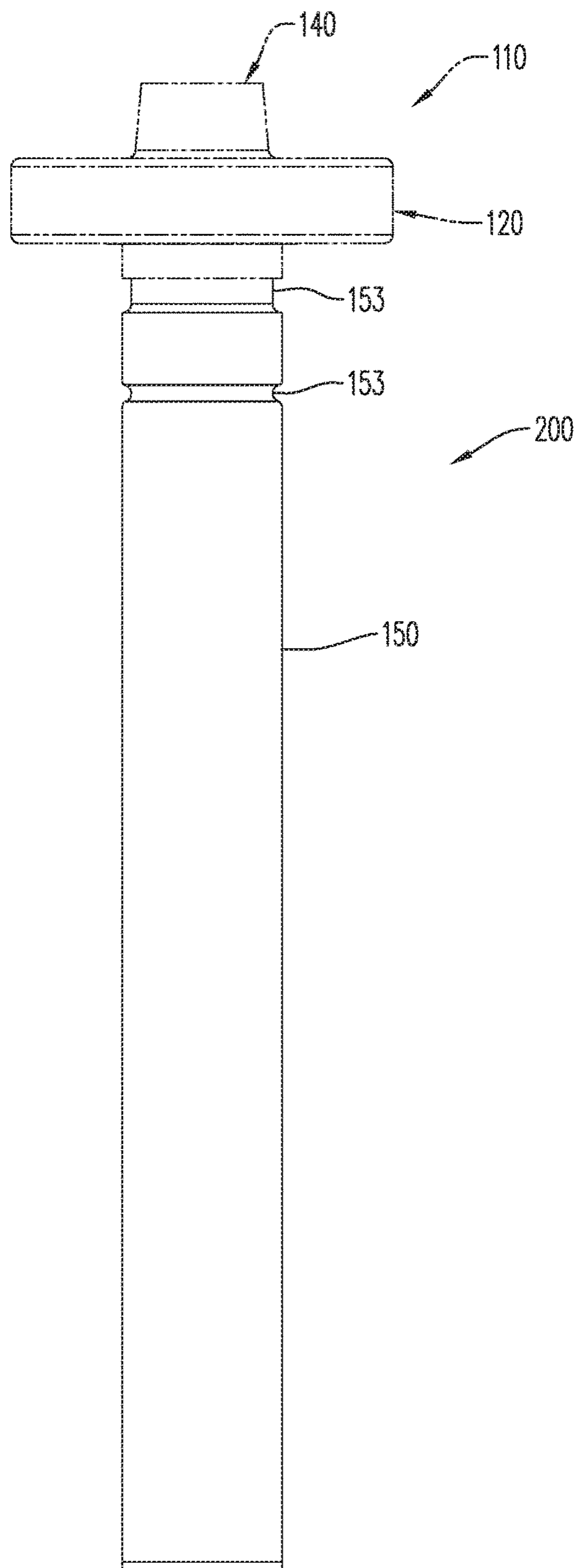
FIG. 11
