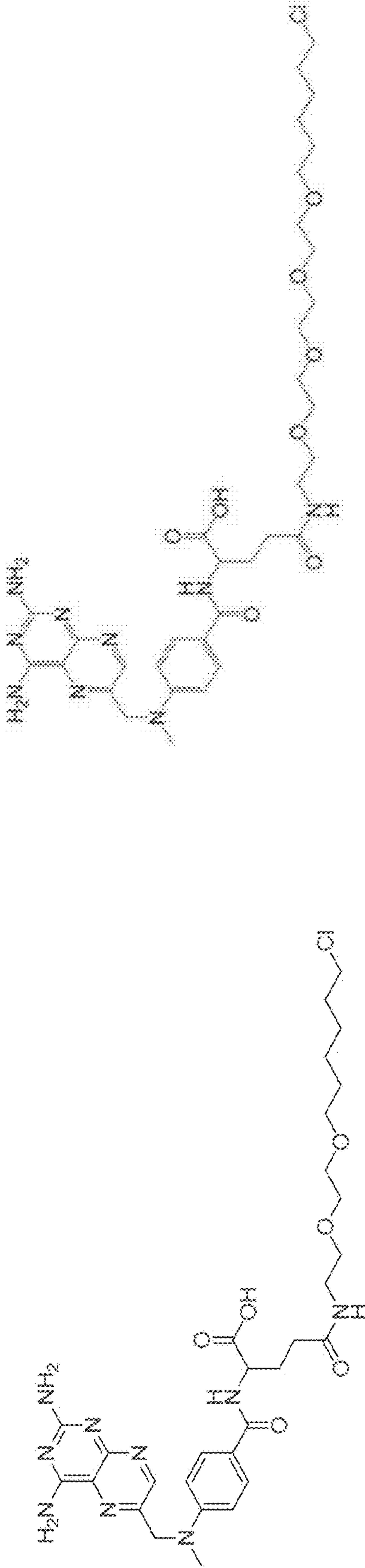
PBI-4848 (Methotrexate-O2 chloroalkane)
