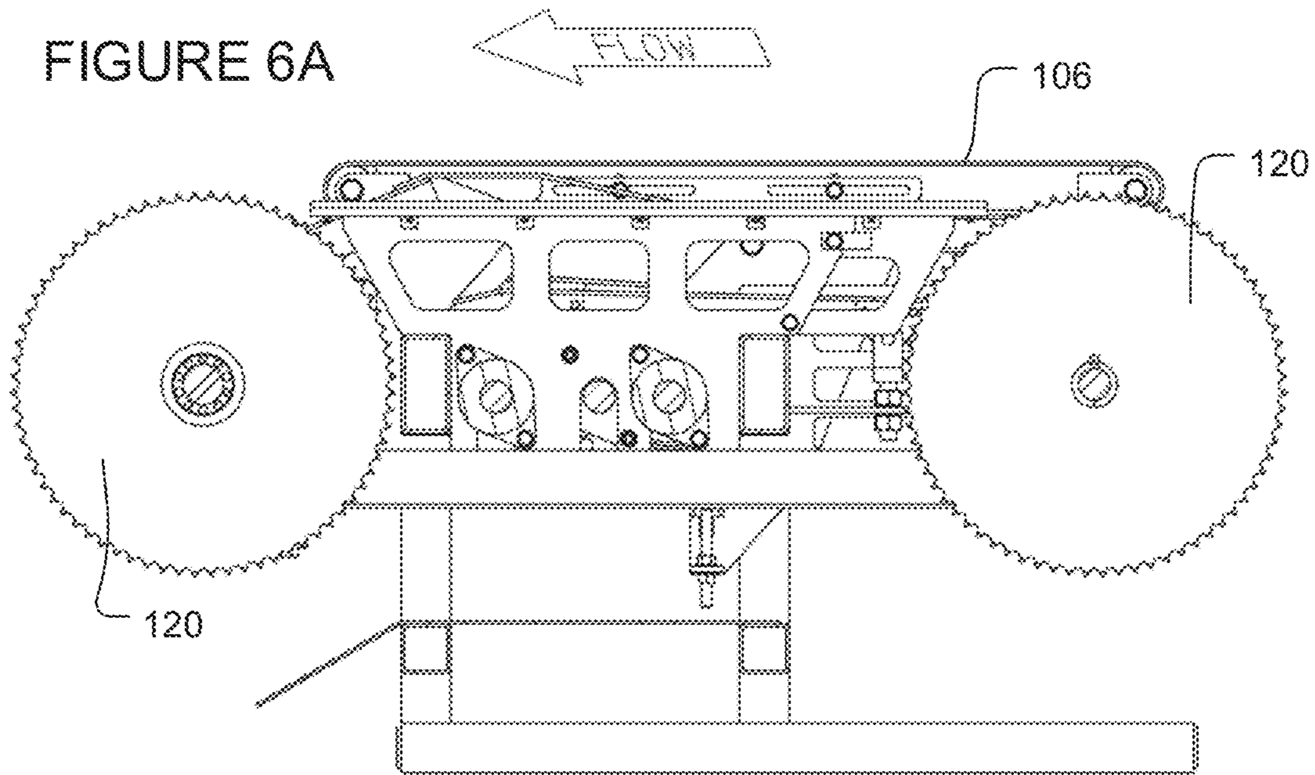
SECTION A-A
