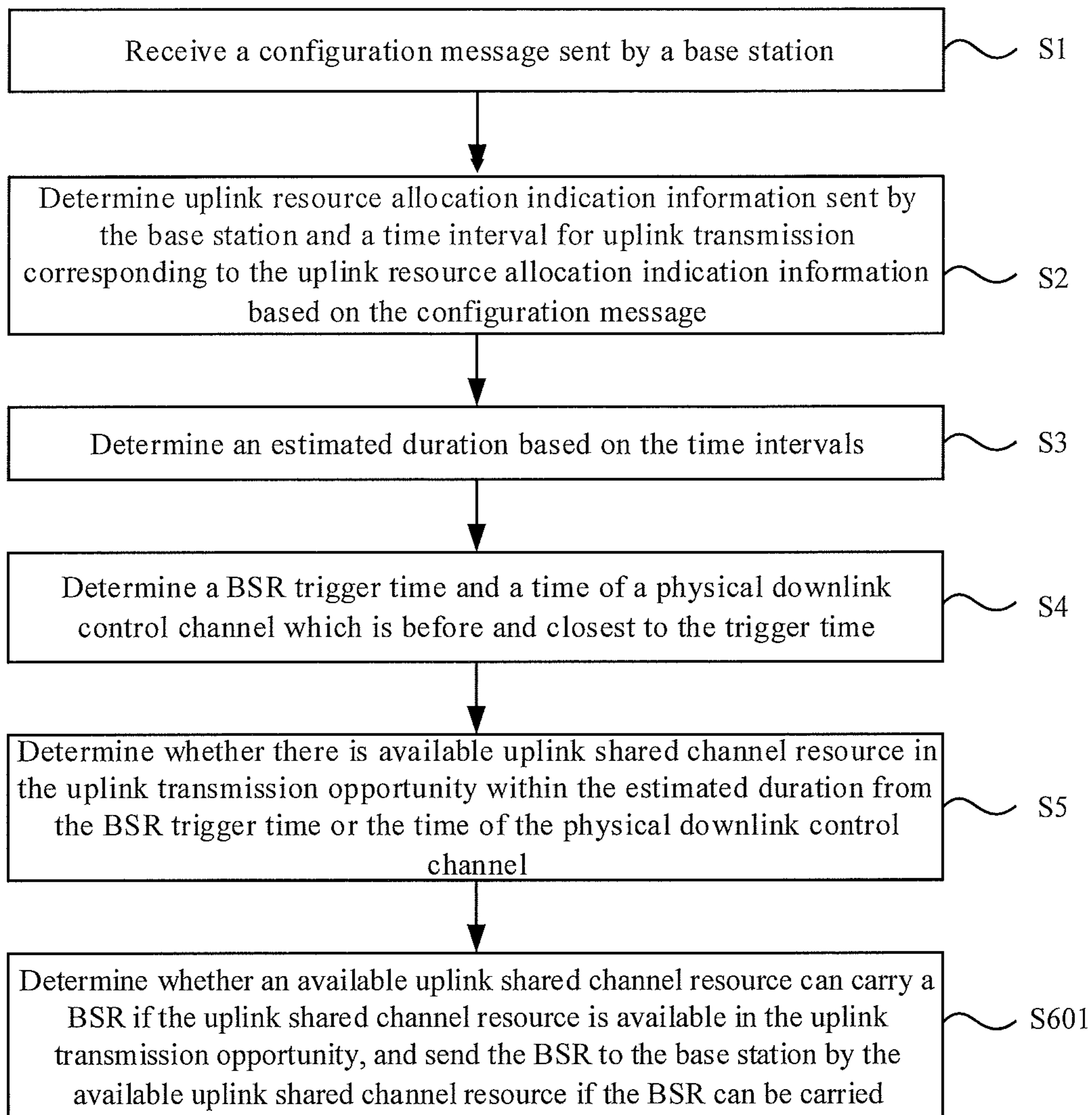
FIG. 11
