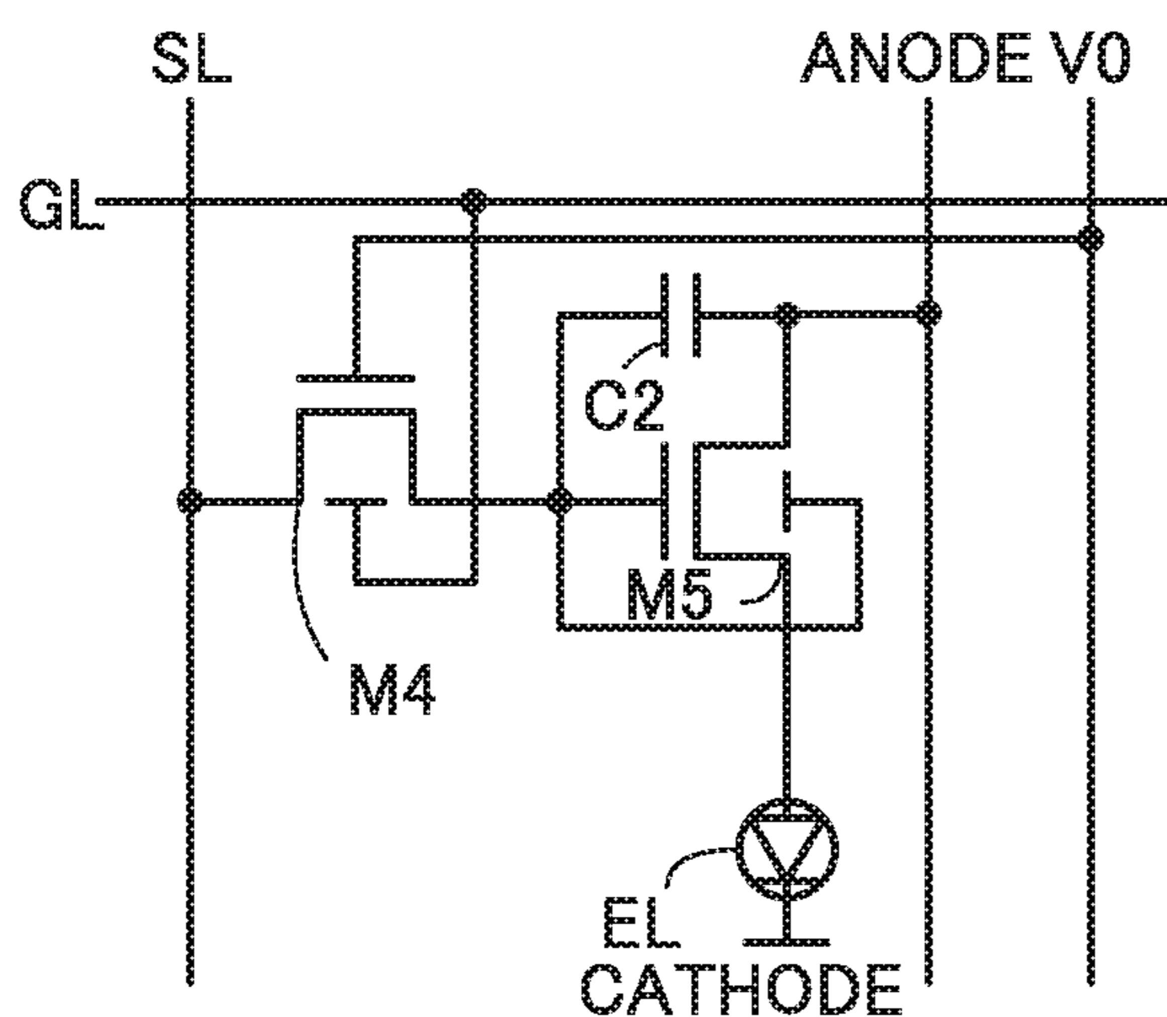
FIG. 26B
