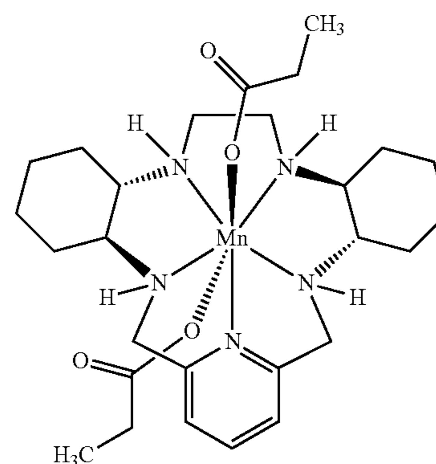
[Bis-Propionato(GC4419)] C_{27}H_{45}MnN_5O_4 MW 558.63
