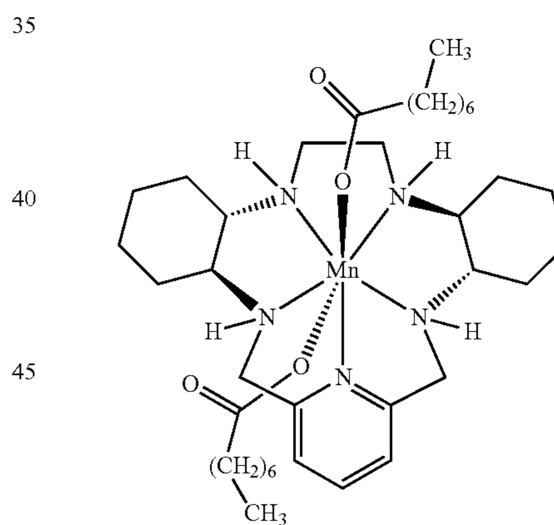
[Bis-Octanoato(GC4419)] C 37 H 65 MnN 5 O 4 MW 698.90
