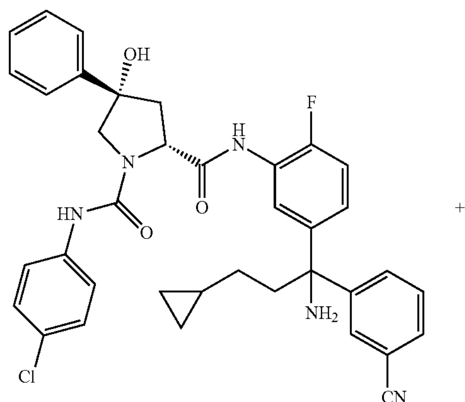
30a (+)-isomer
