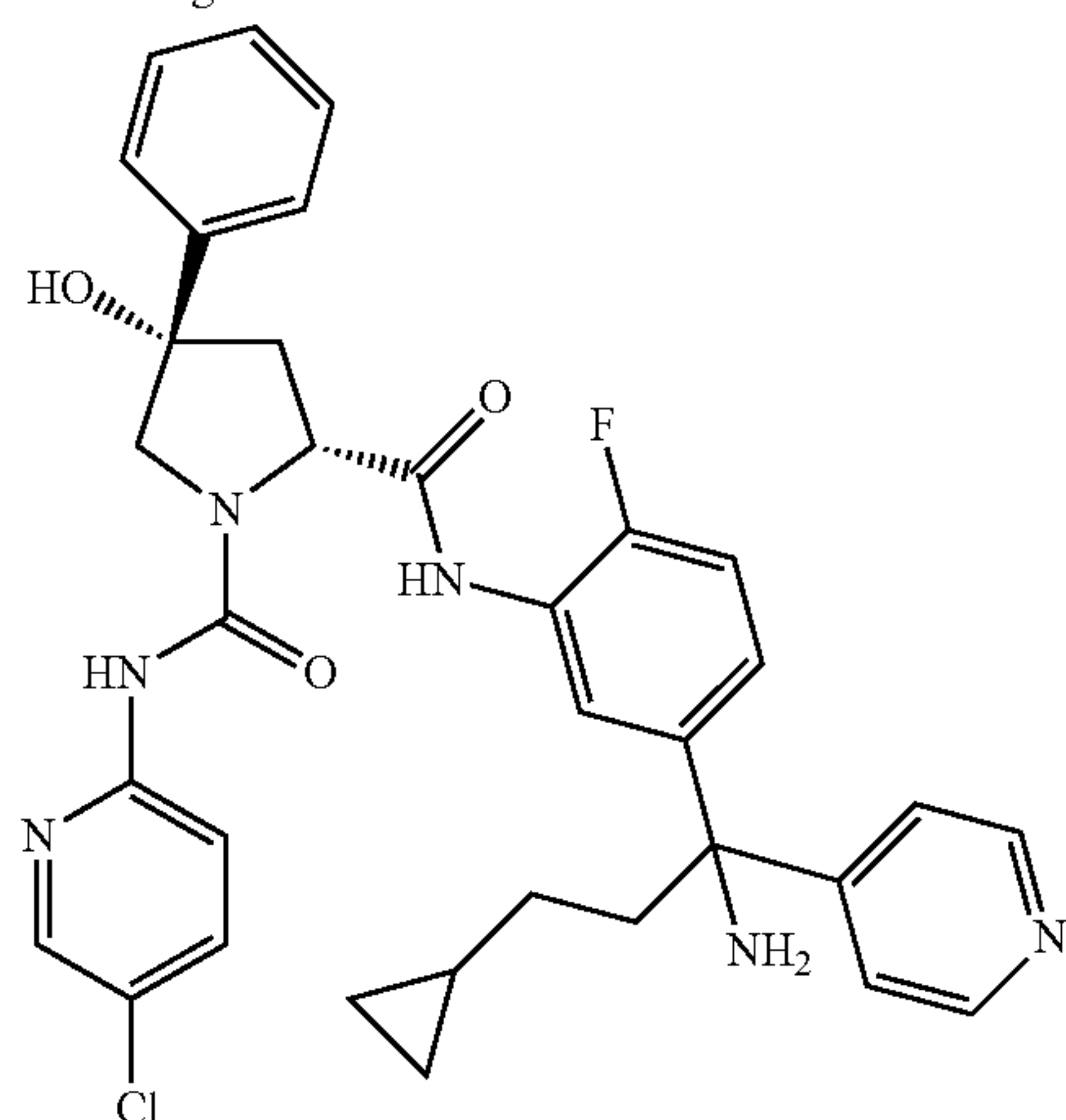
39h (+)-isomer
