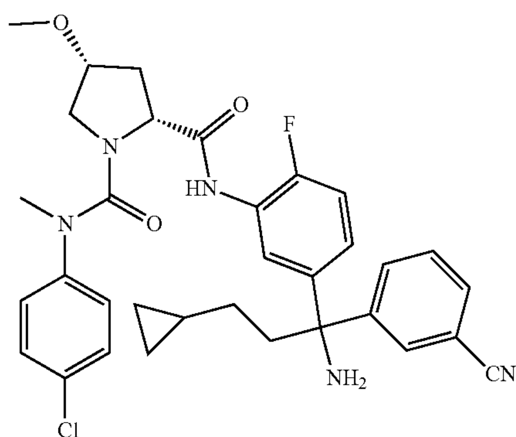
6e (-)-isomer
