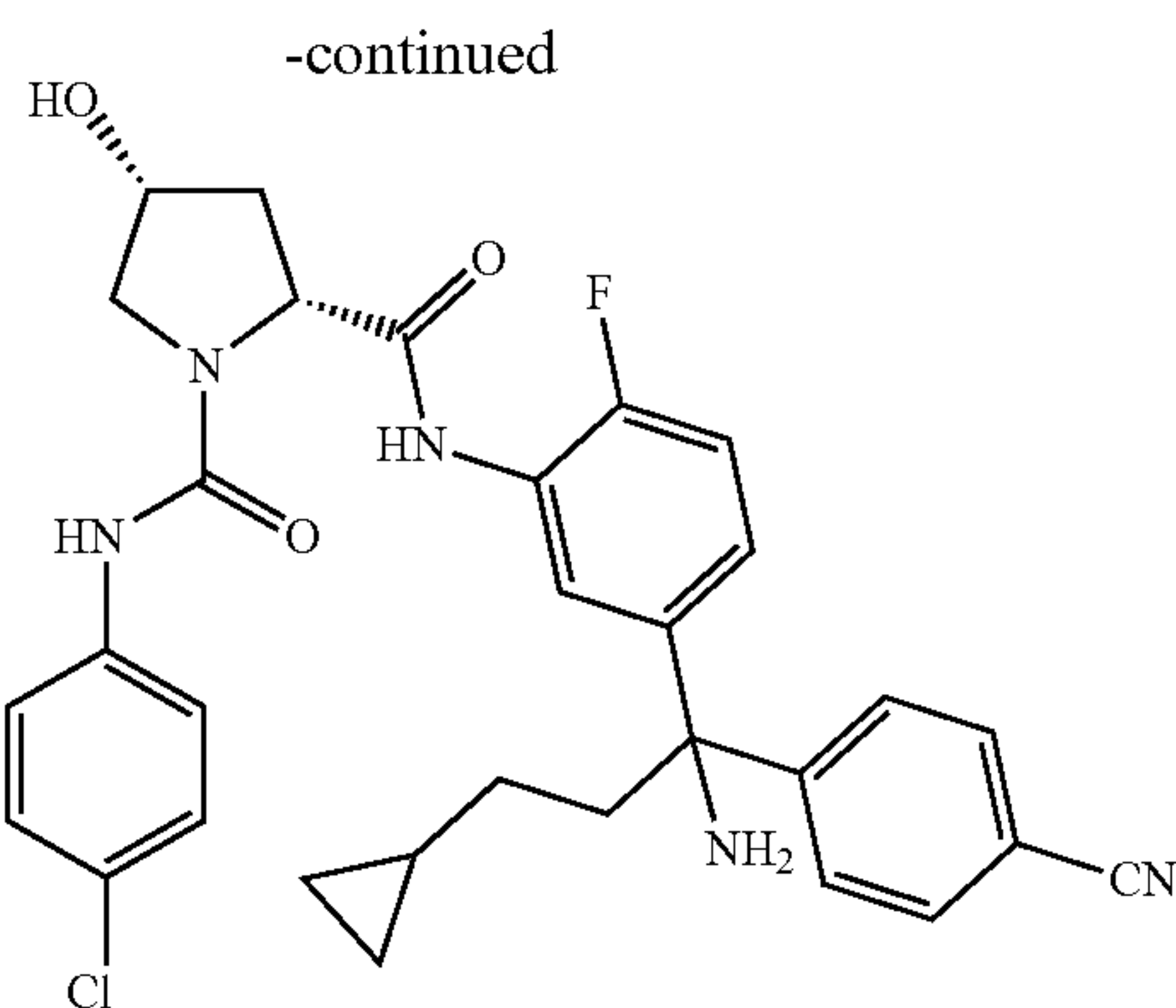
63g (+) isomer
