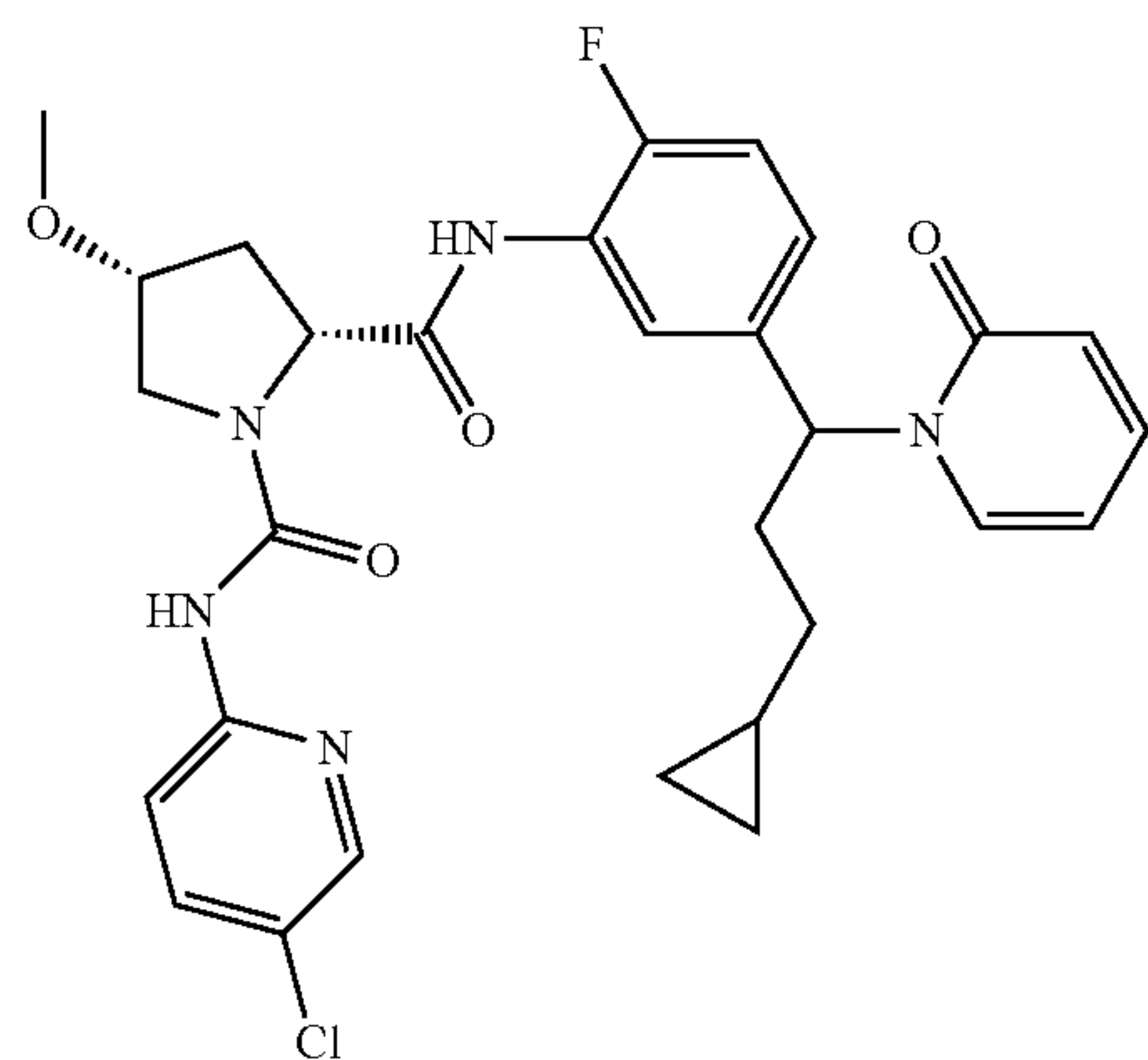
43m (+)-isomer
