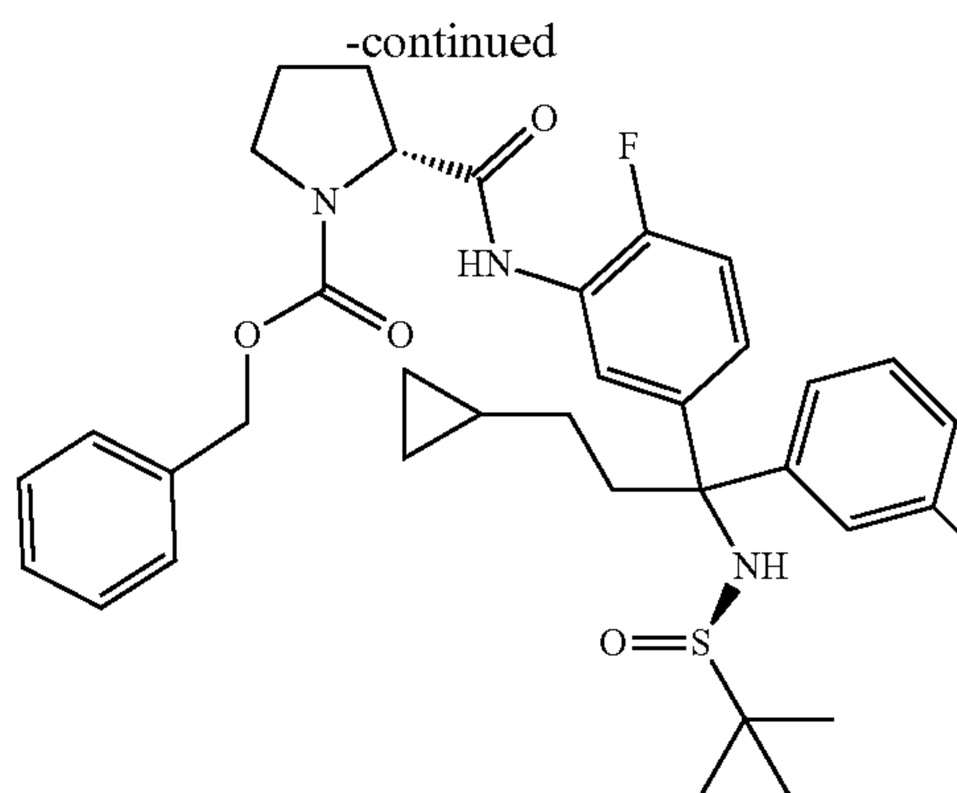
12b (-)-isomer
