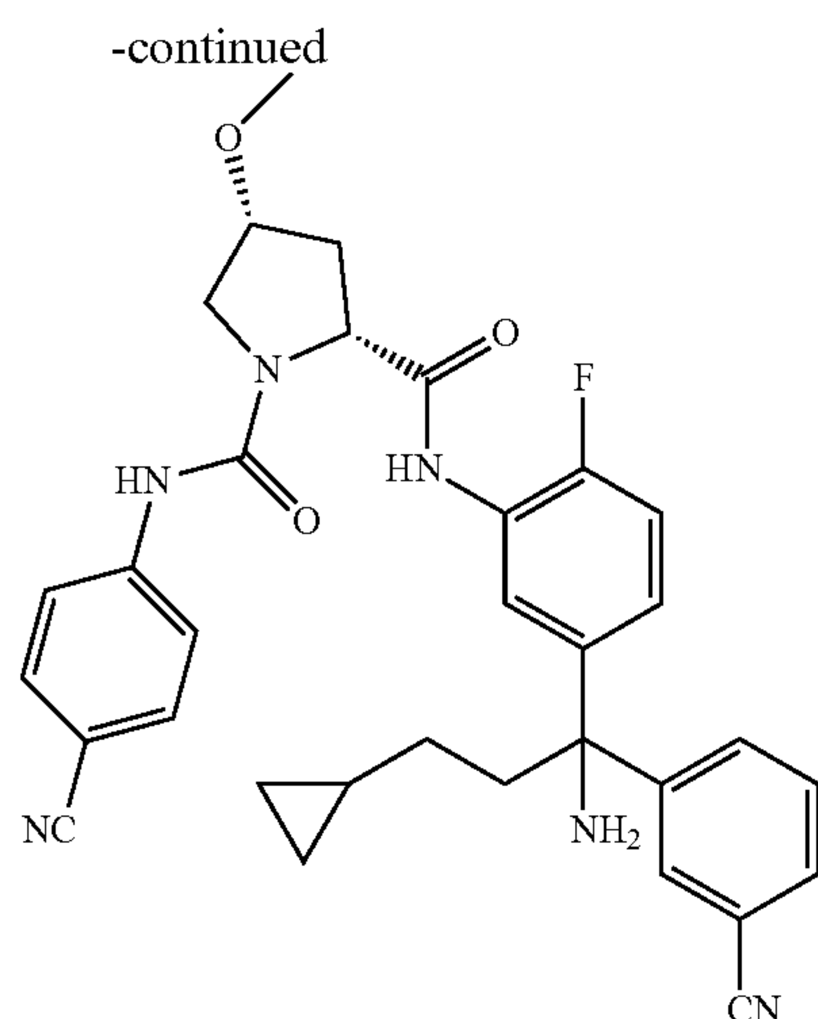
15f (+)-isomer
