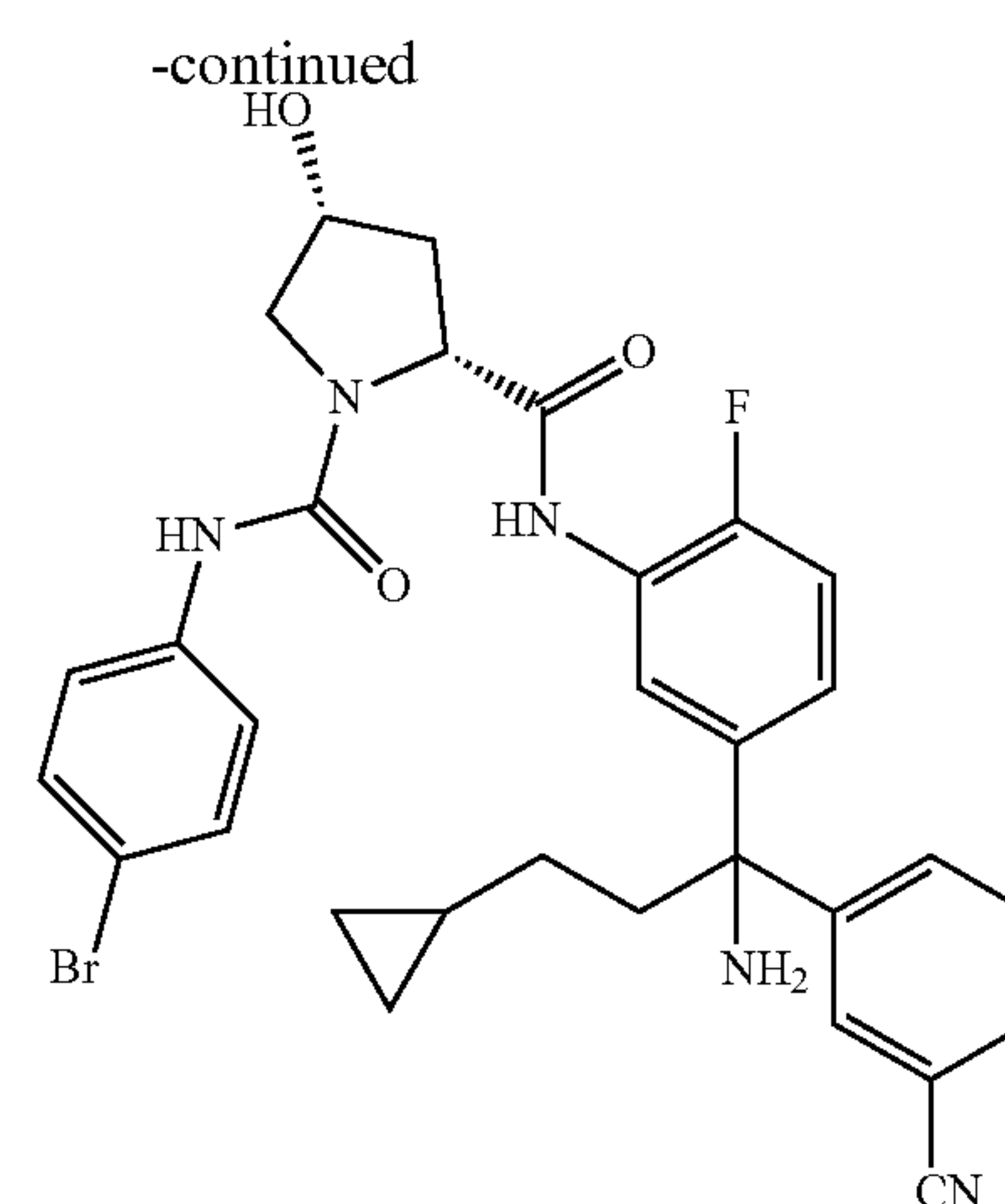
23b (+)-isomer
