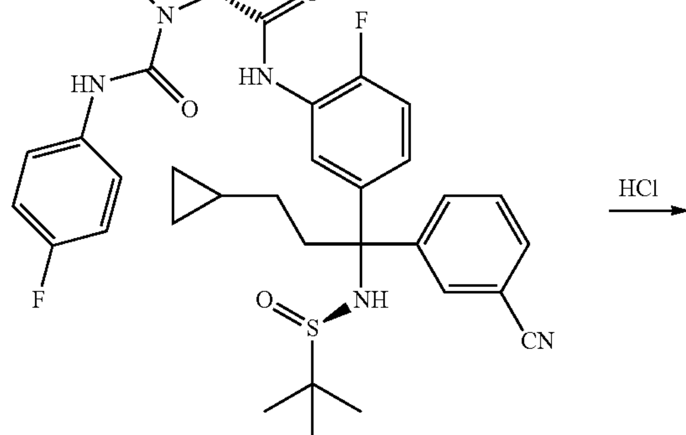
24a (-)-isomer
