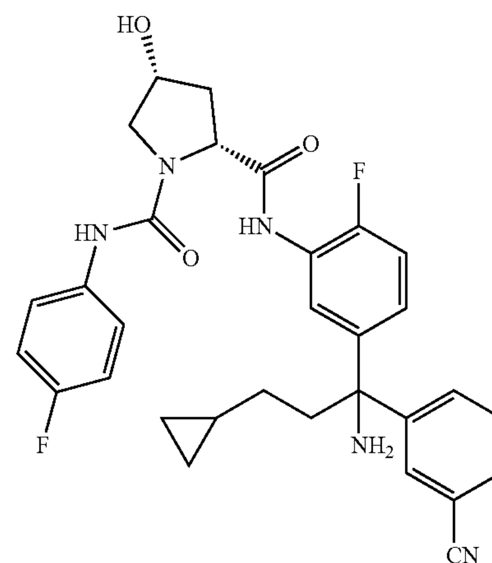
24b (+)-isomer
