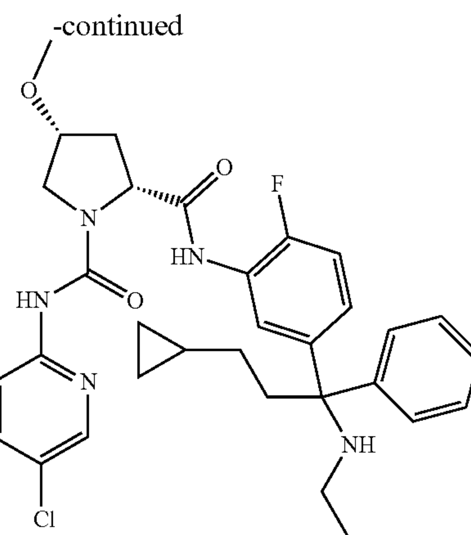
67b (+)-isomer
