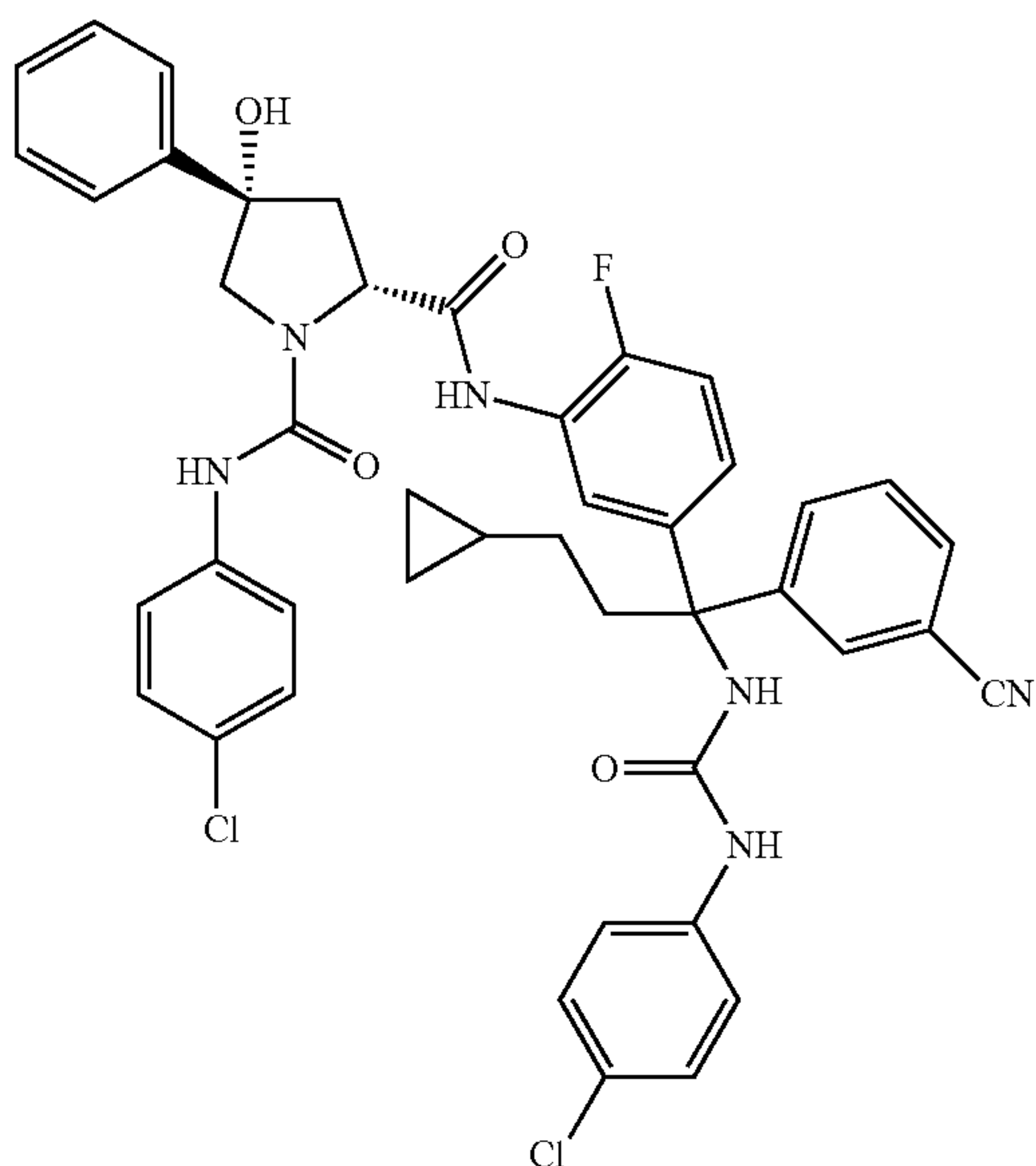
30b (+)-isomer
