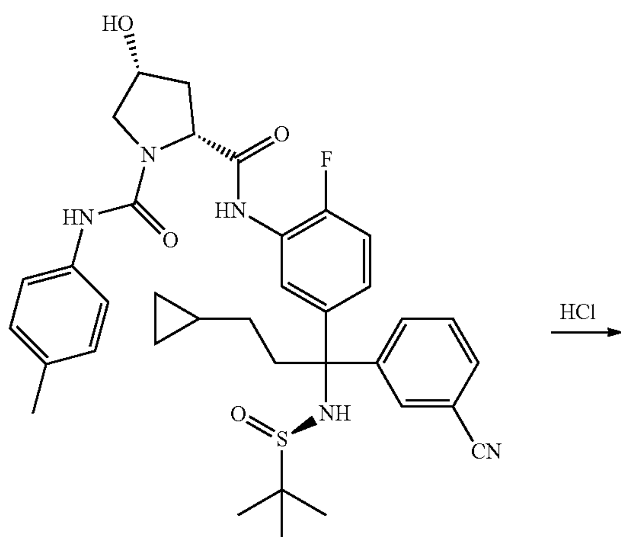
22a (-)-isomer
