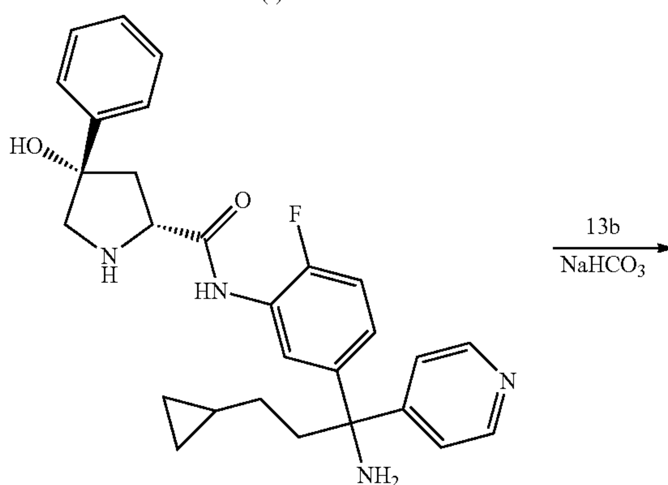
39g
