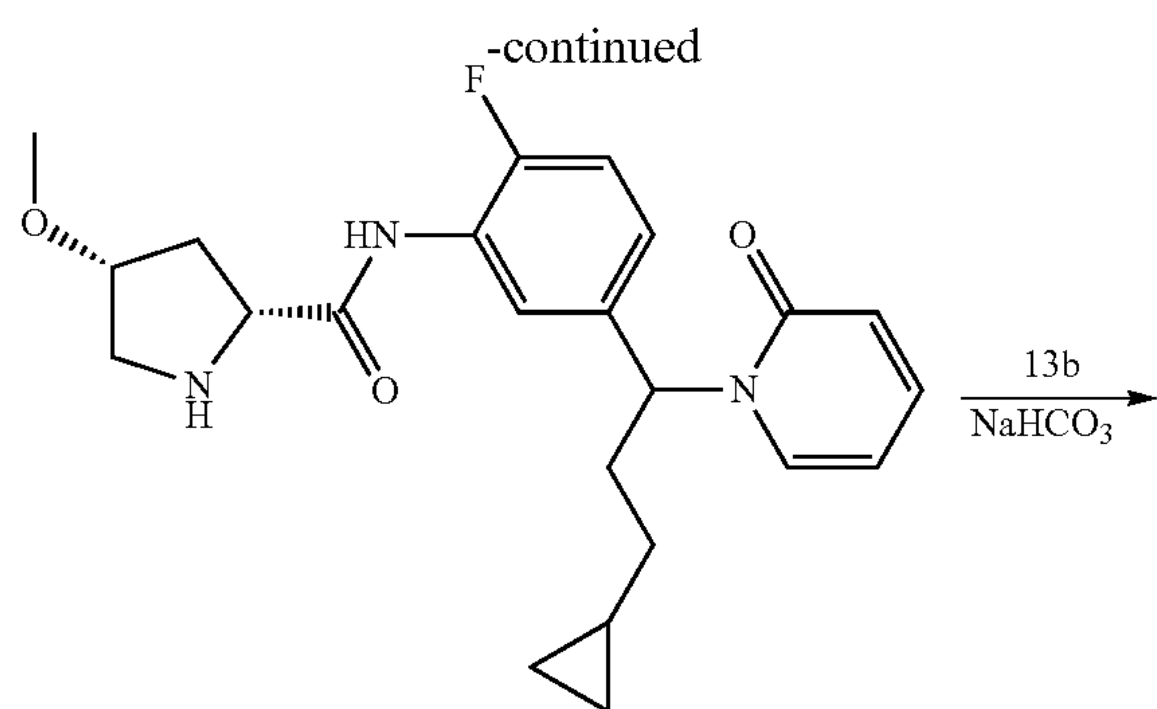
43l (+)-isomer
