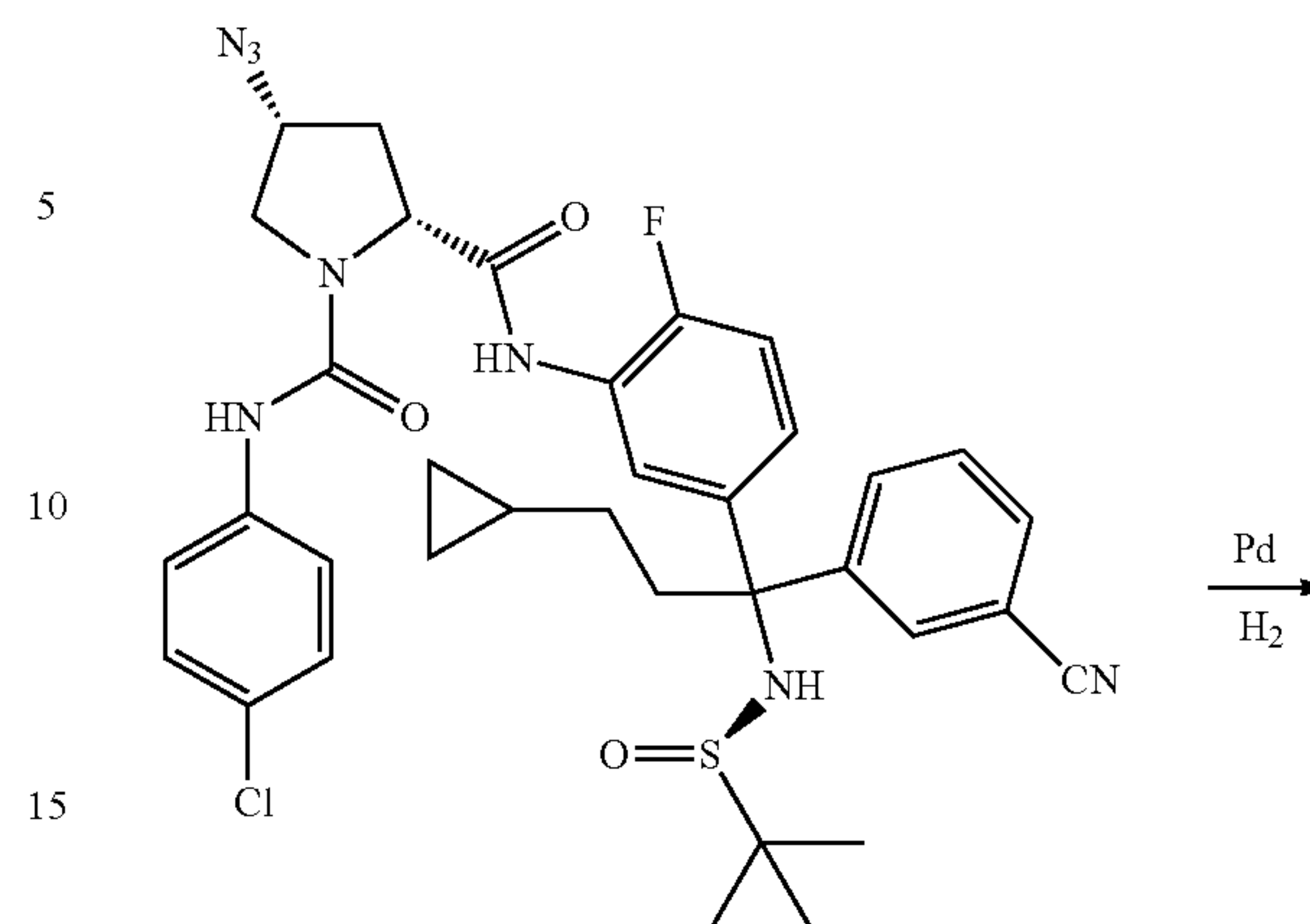
19a
