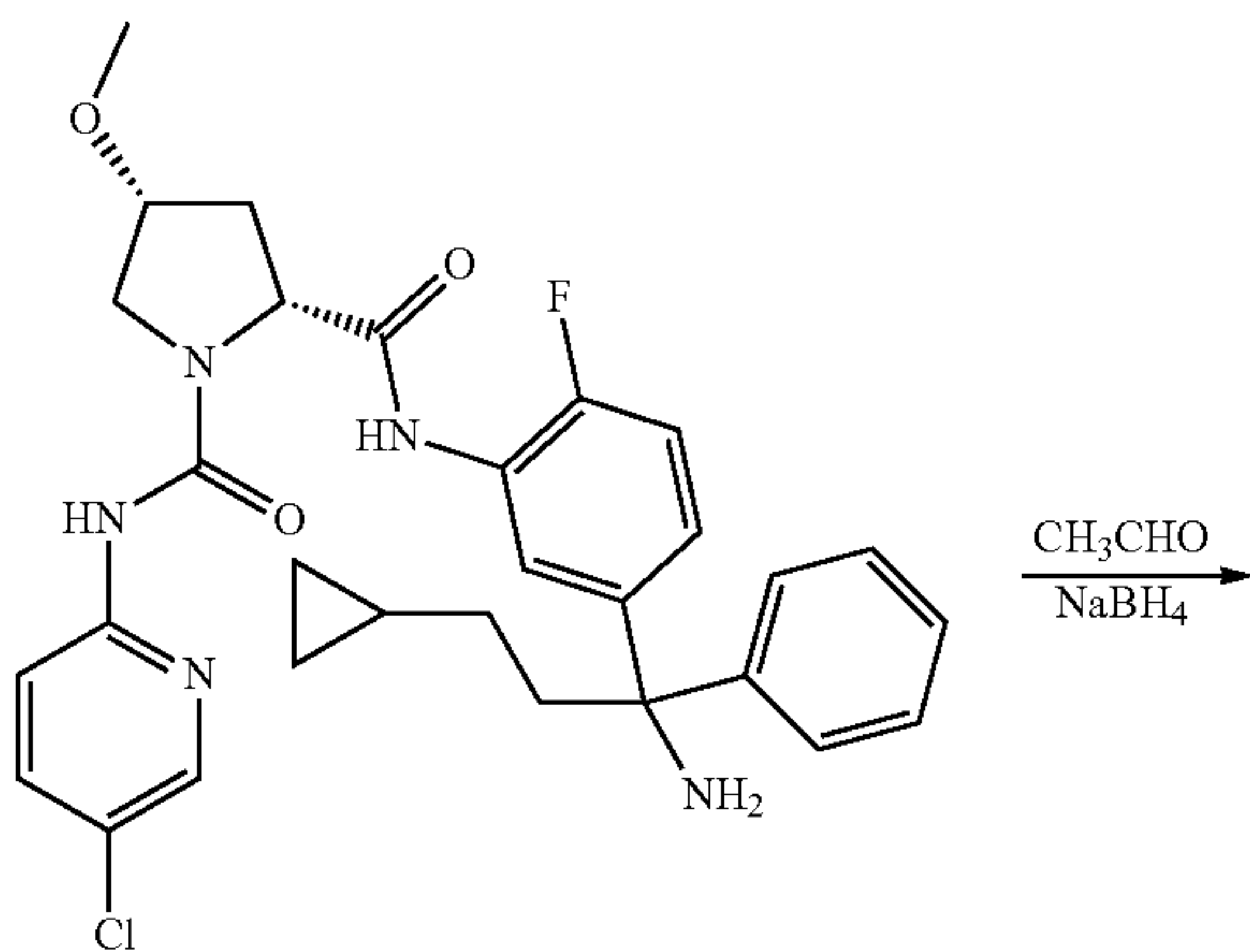
67a
