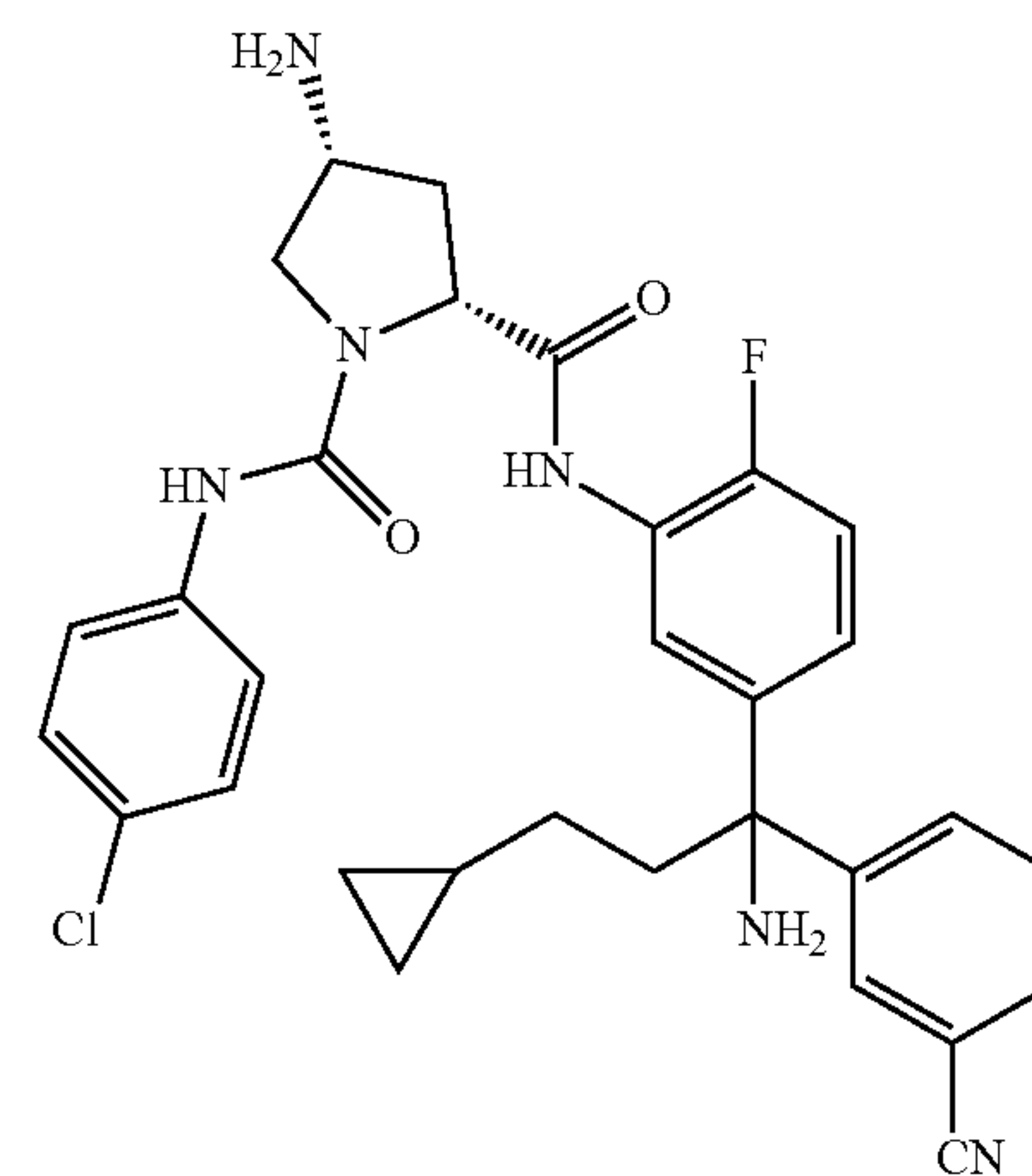
19c (+)-isomer
