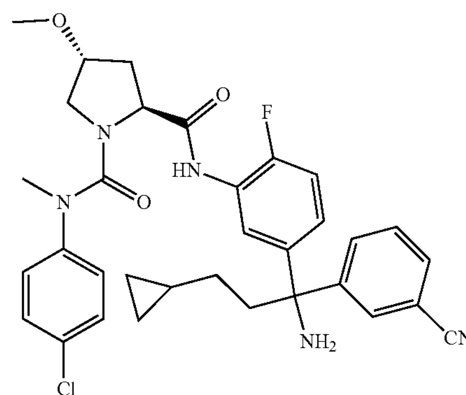
6f (+)-isomer
