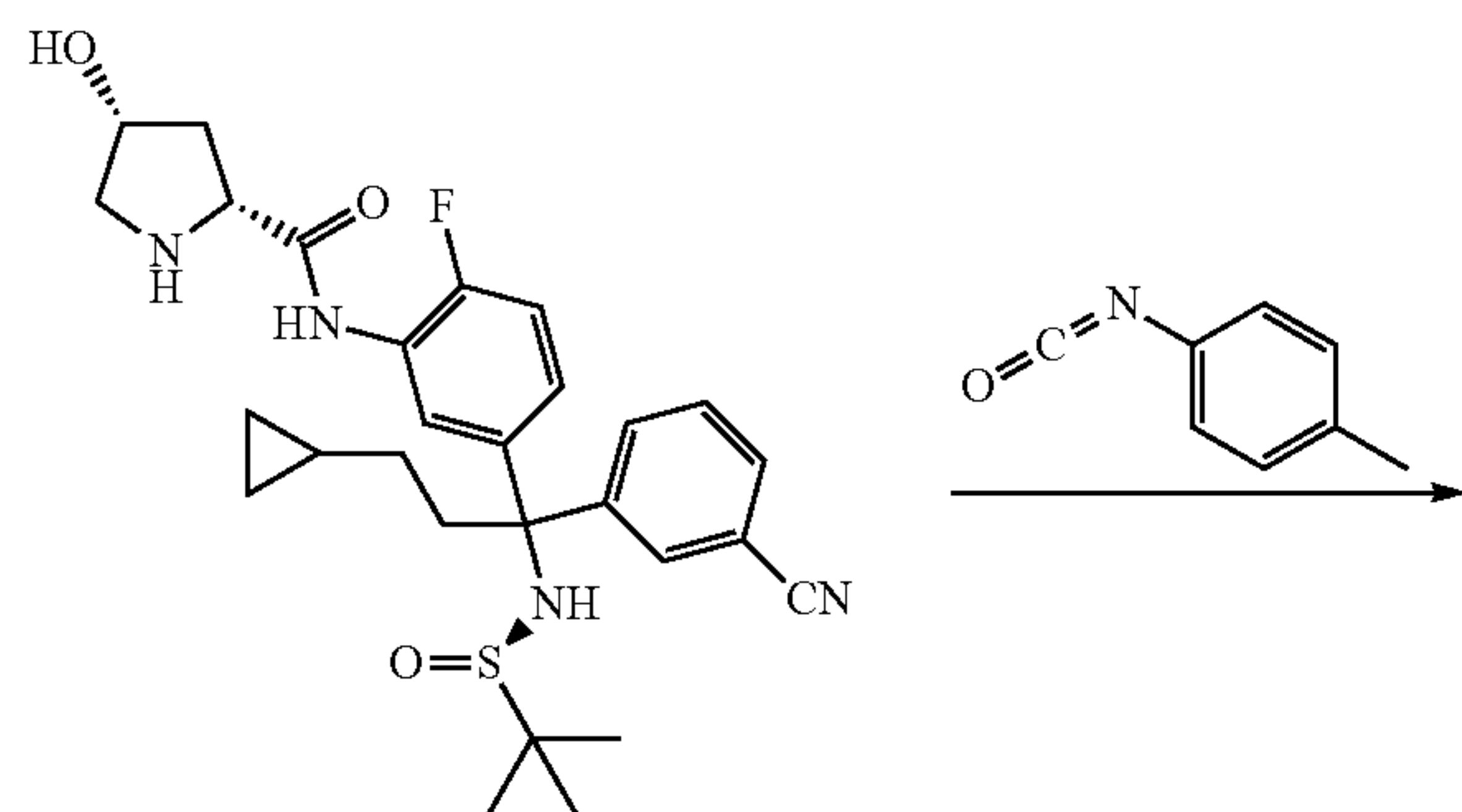
21b (-)-isomer
