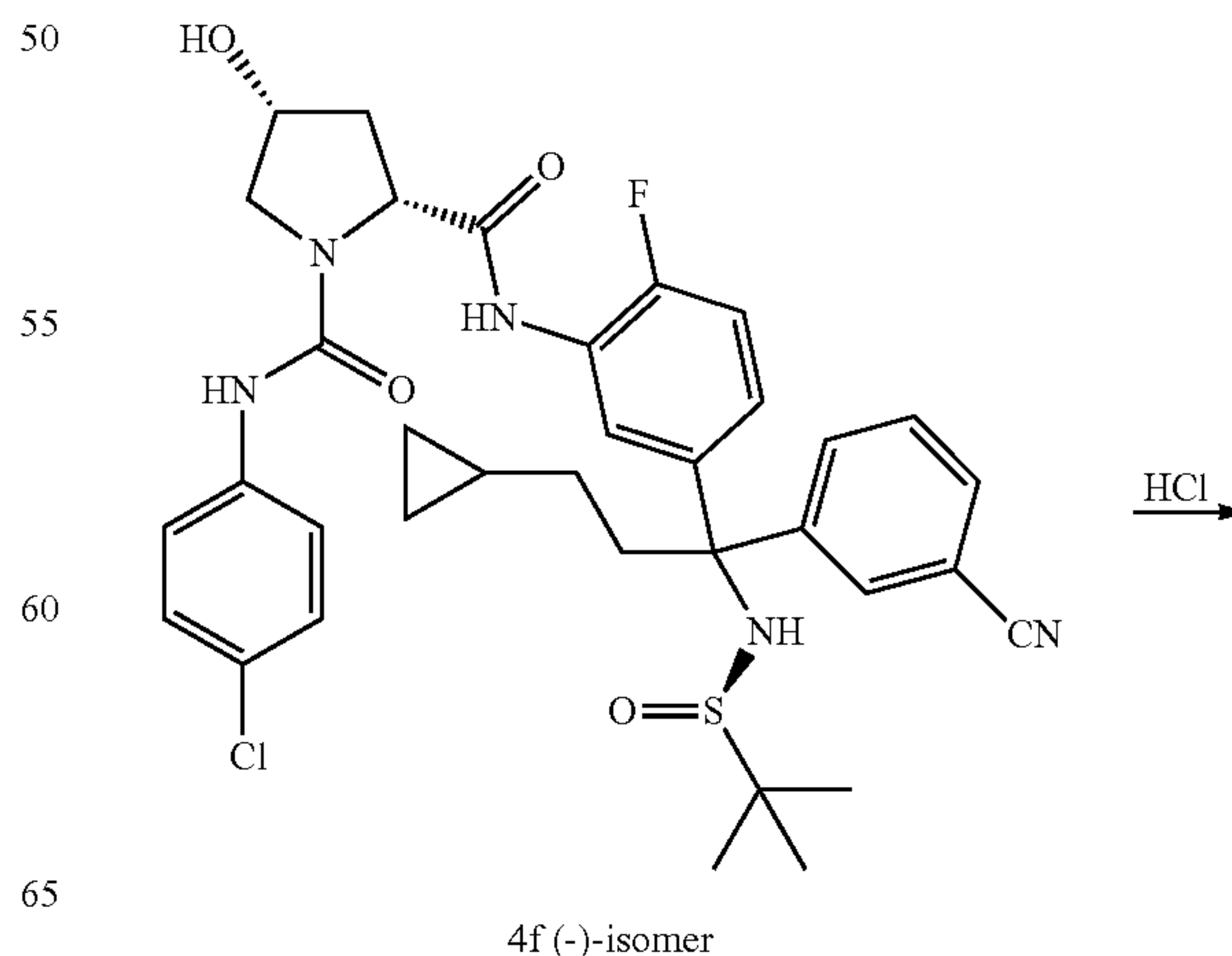
1o
