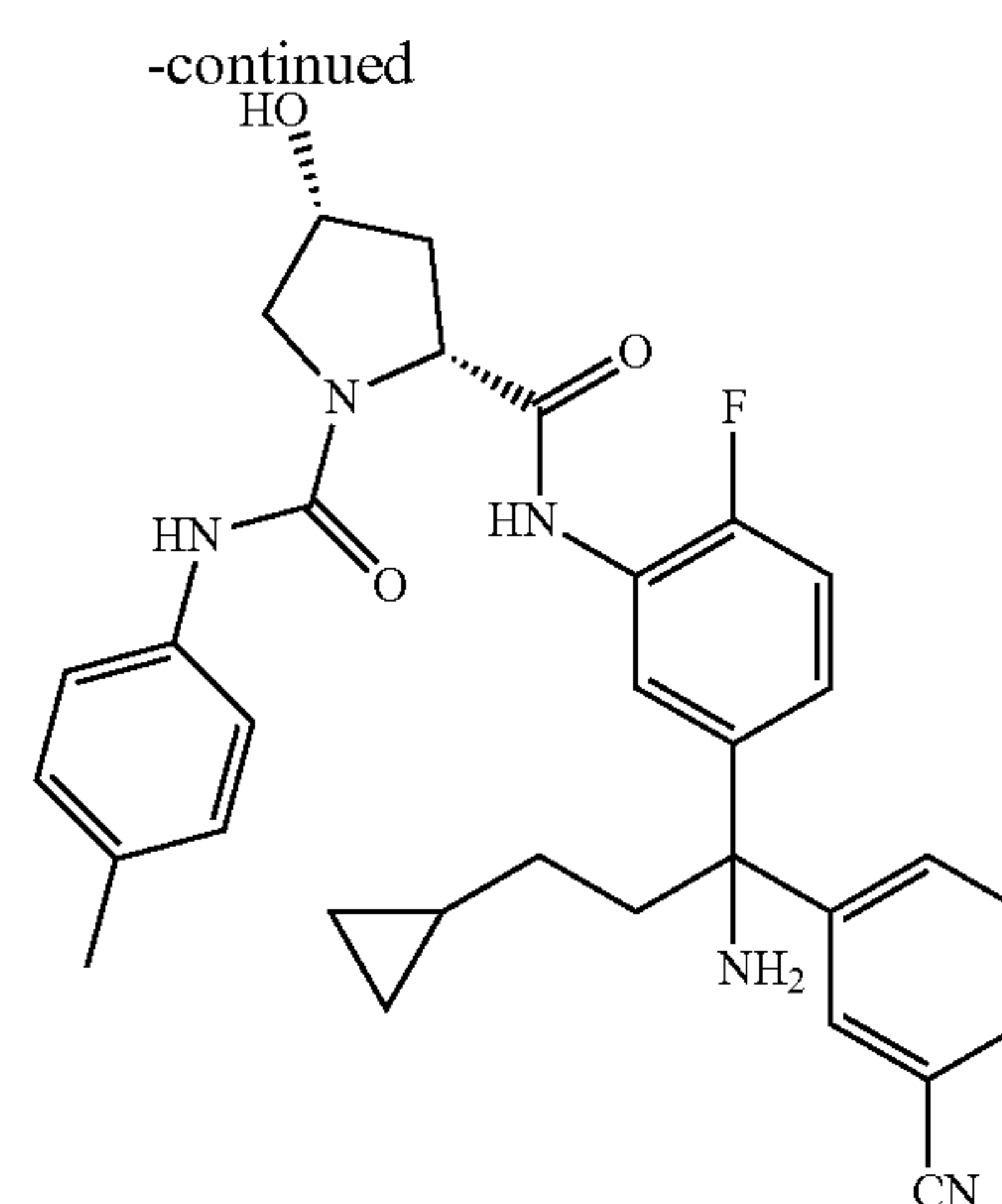
22b (+)-isomer
