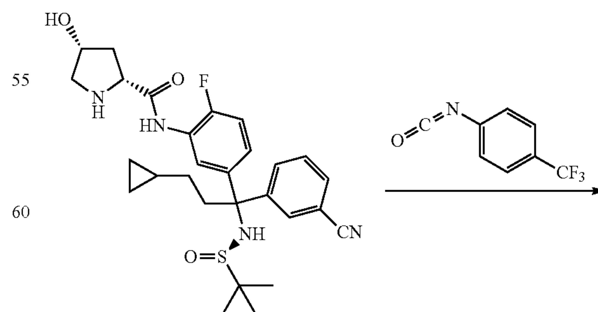
21b (-)-isomer
