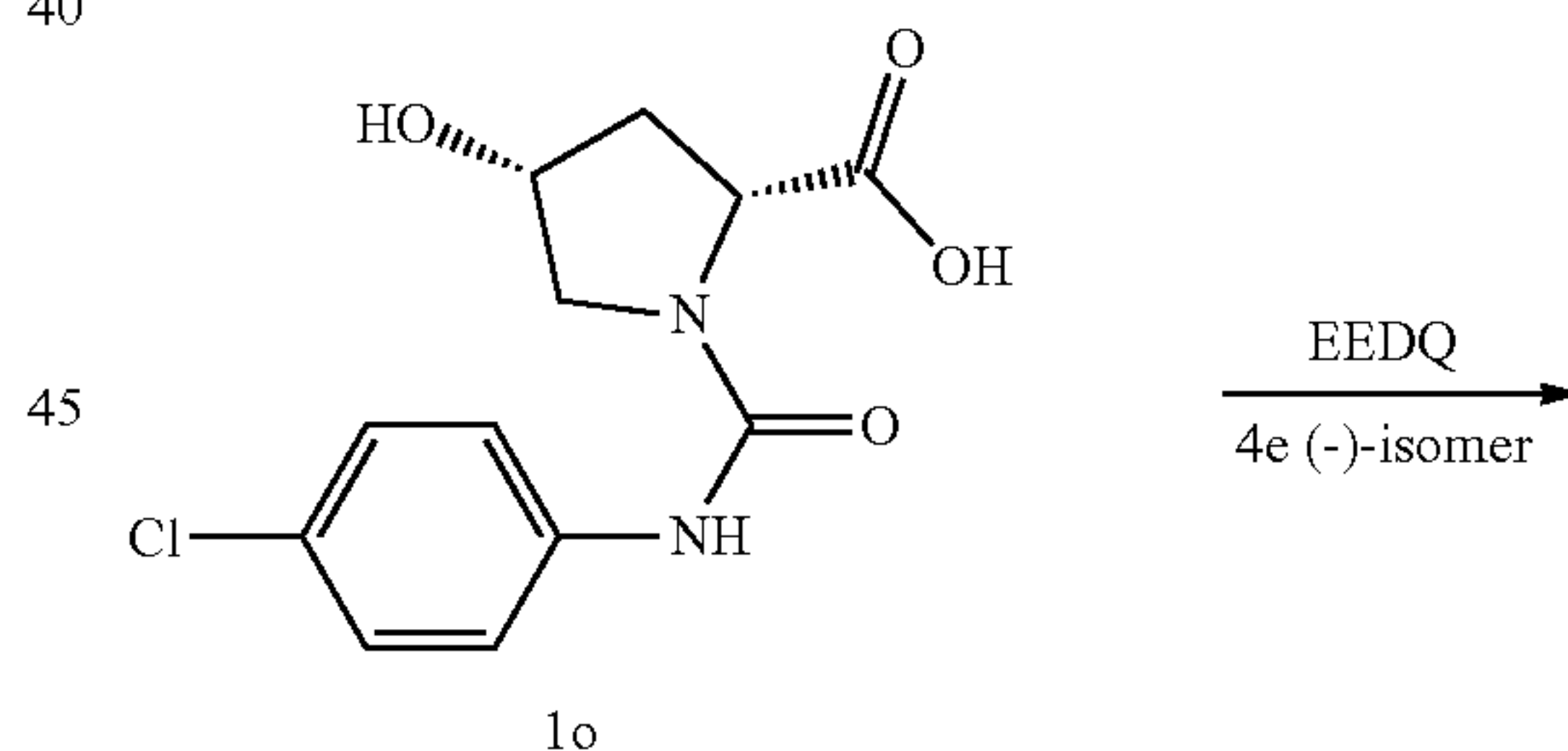
1o
