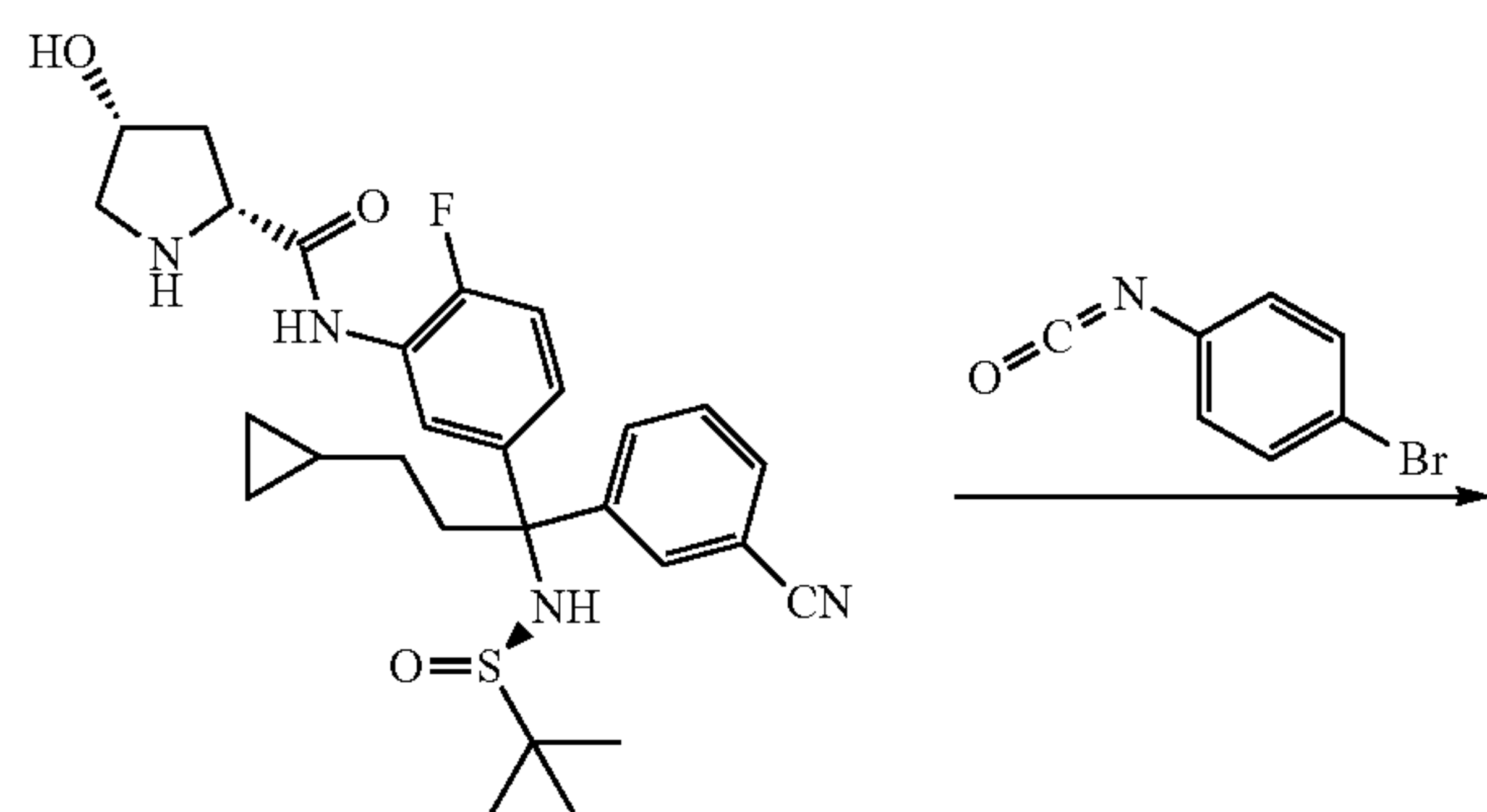
21b (-)-isomer
