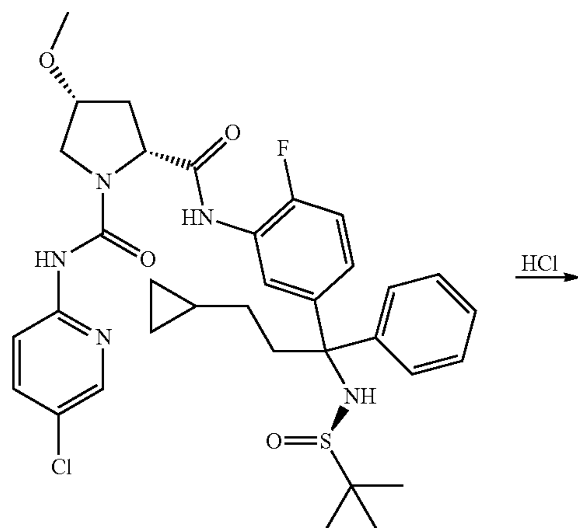
66c (+)-isomer
