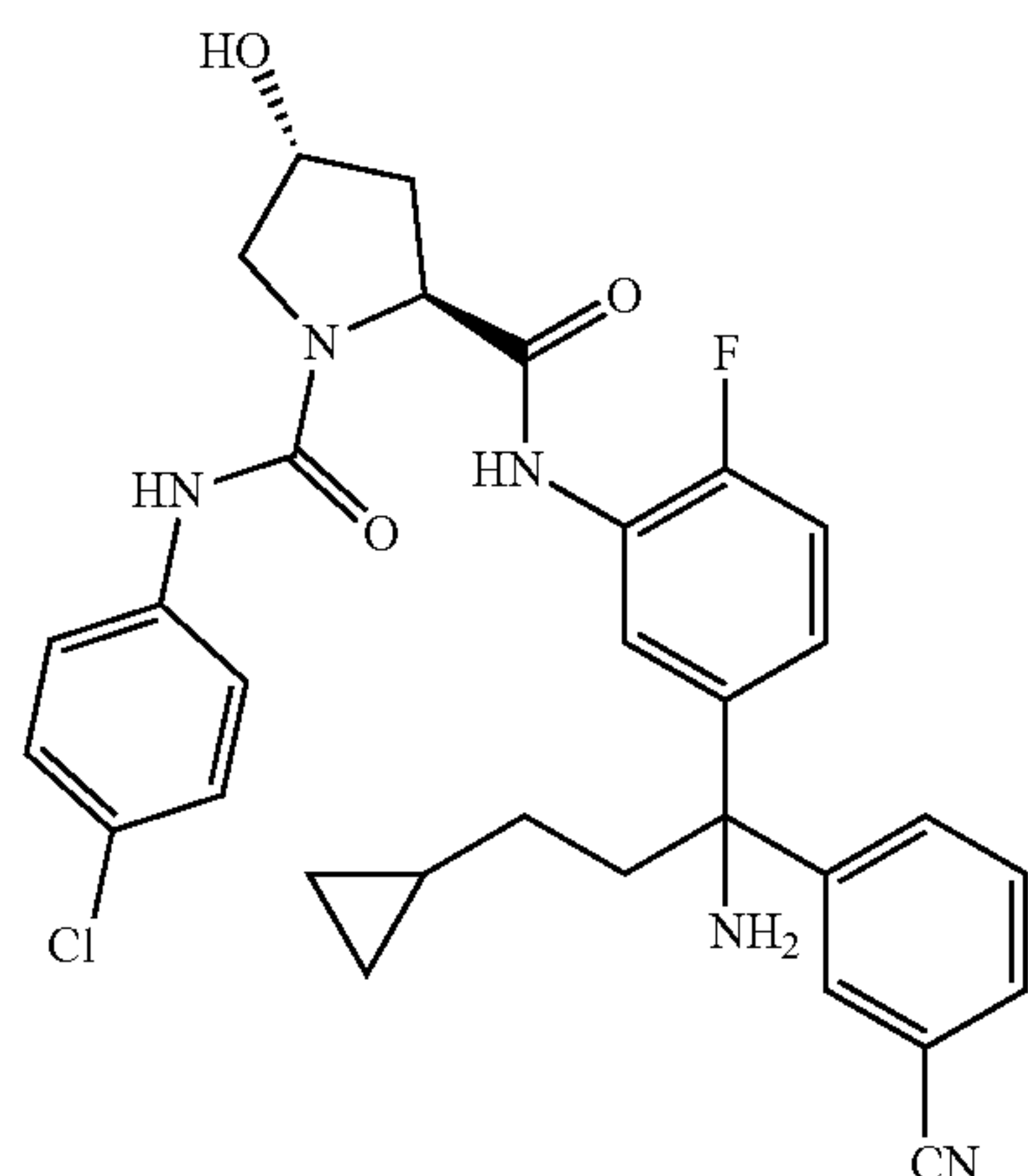
5e (-)-isomer
