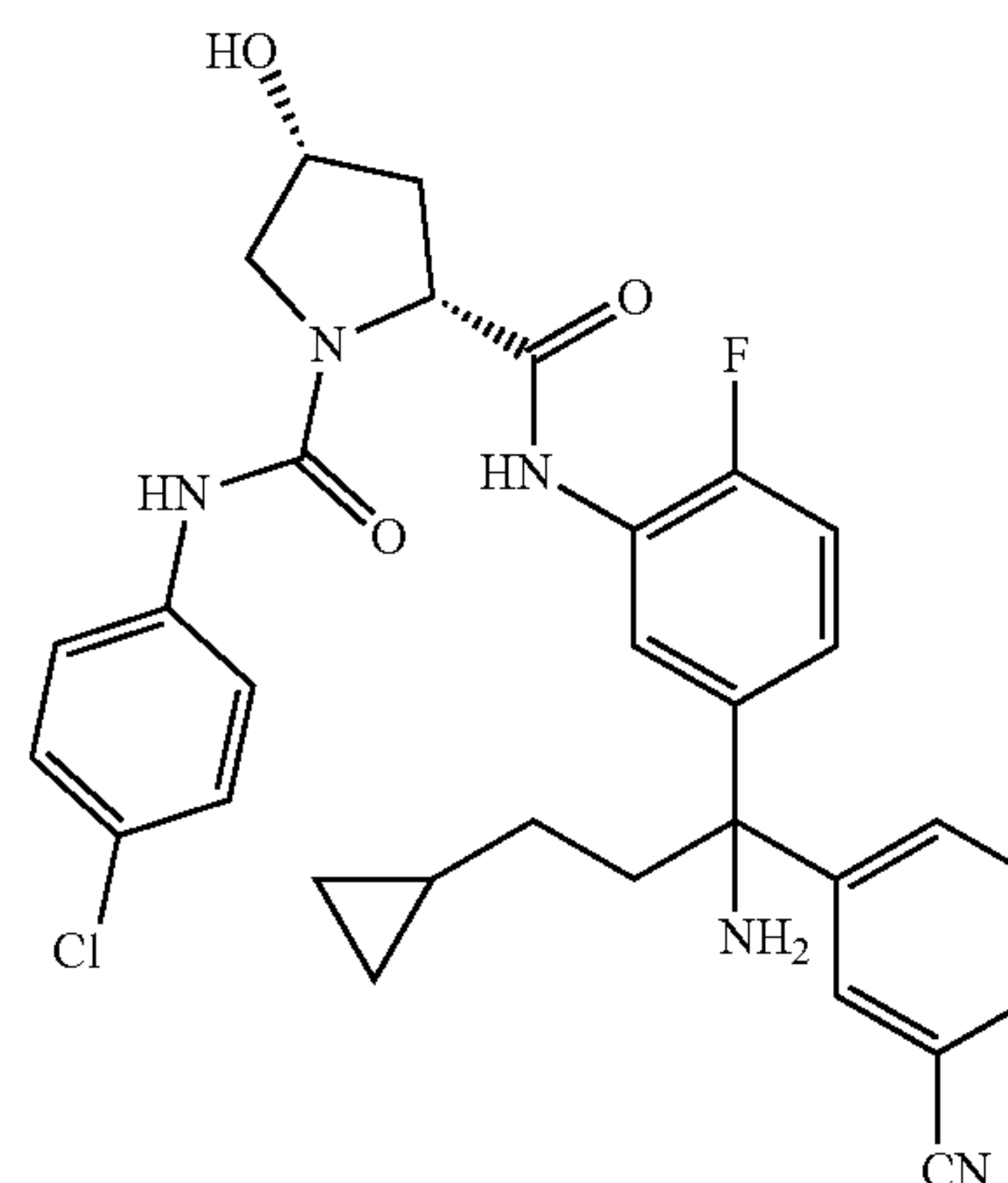
4g (+)-isomer
