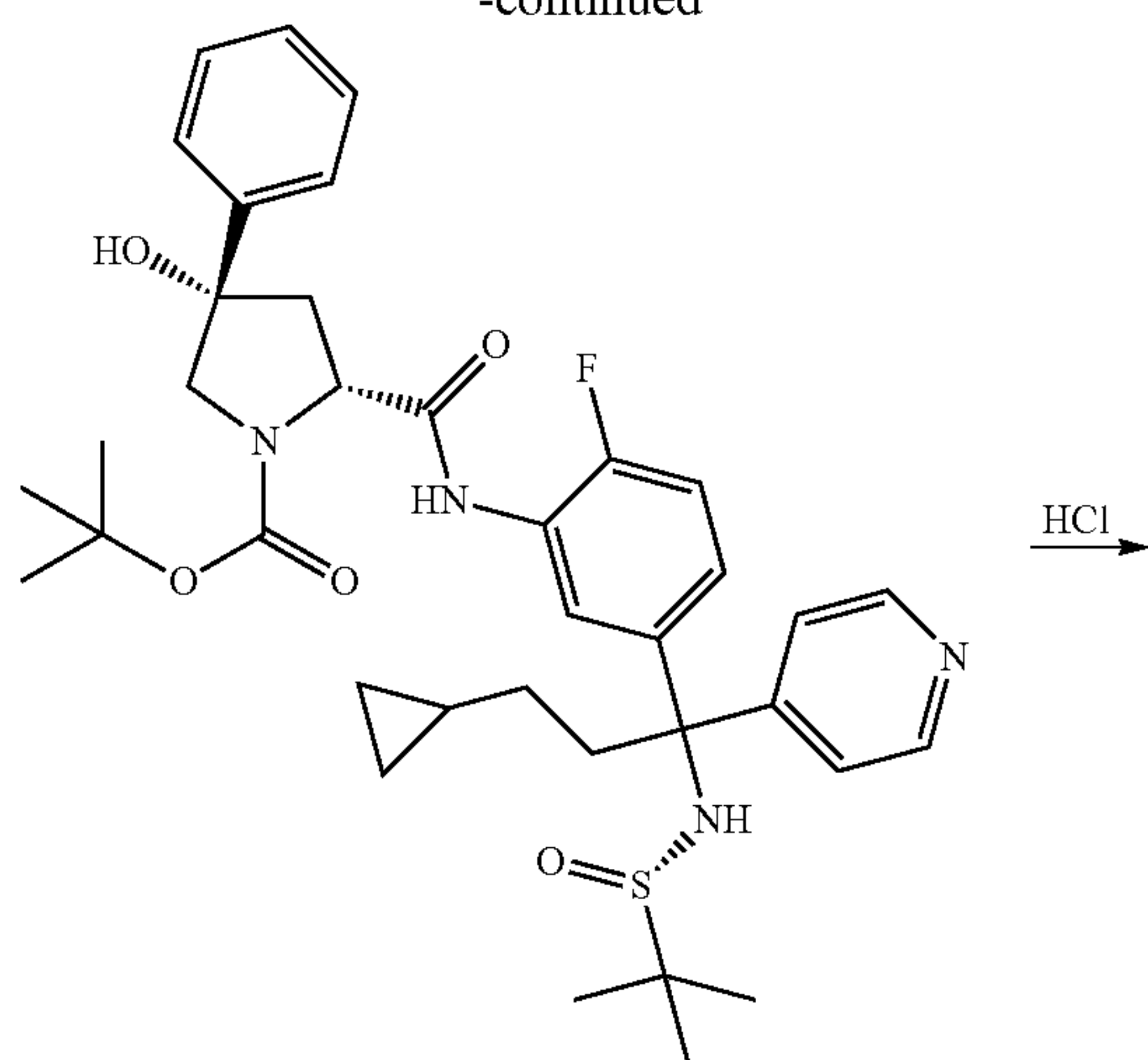
39f (-)-isomer
