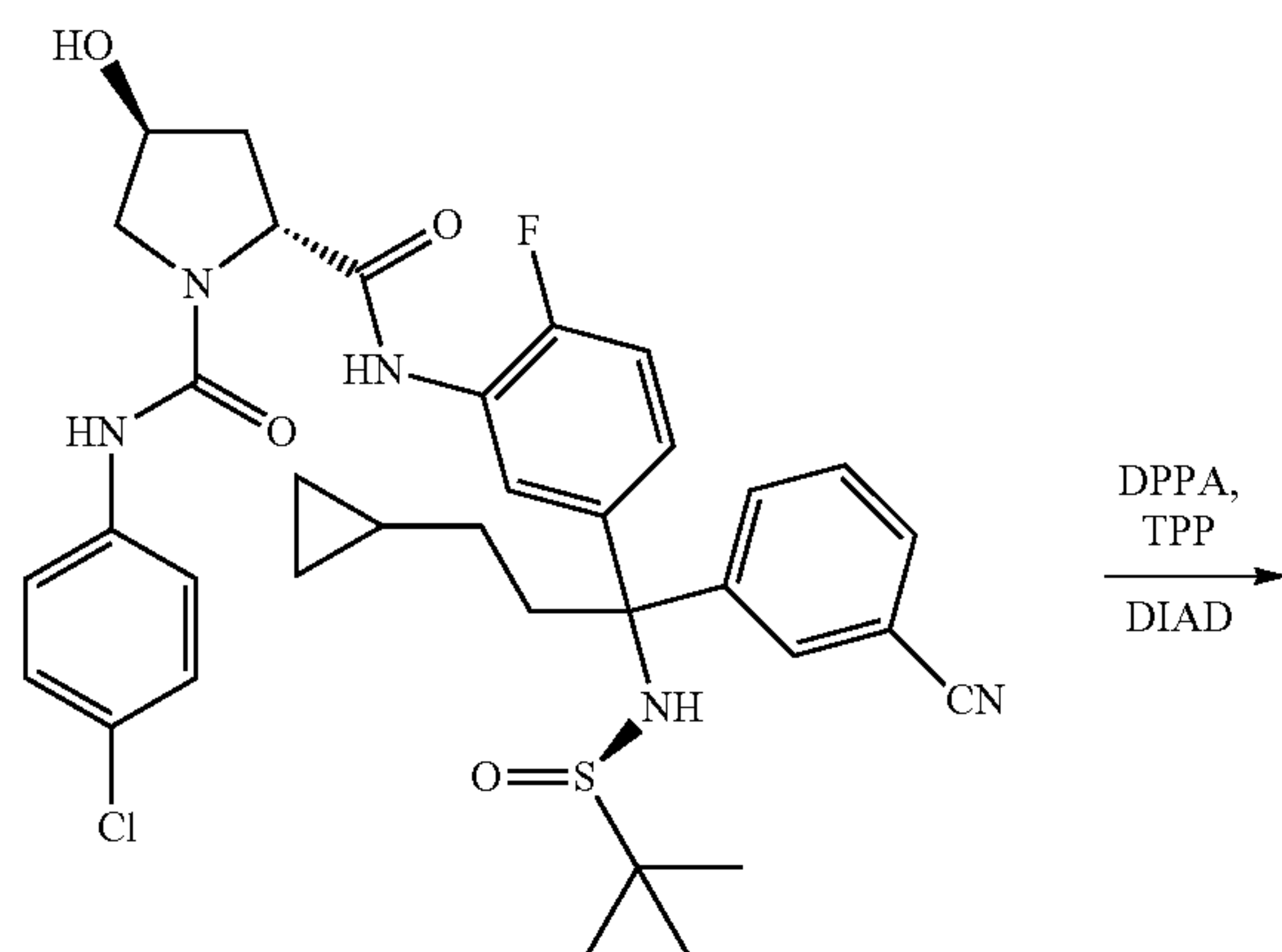
9b (+)-isomer
