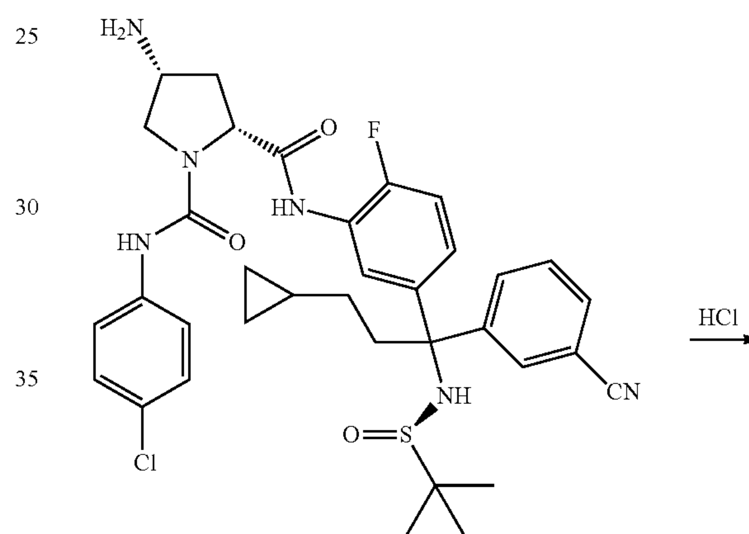
19b
