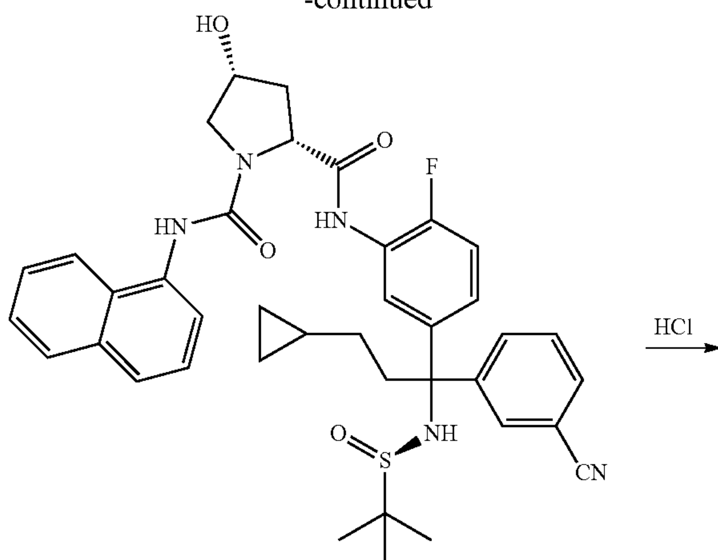
26a (-)-isomer
