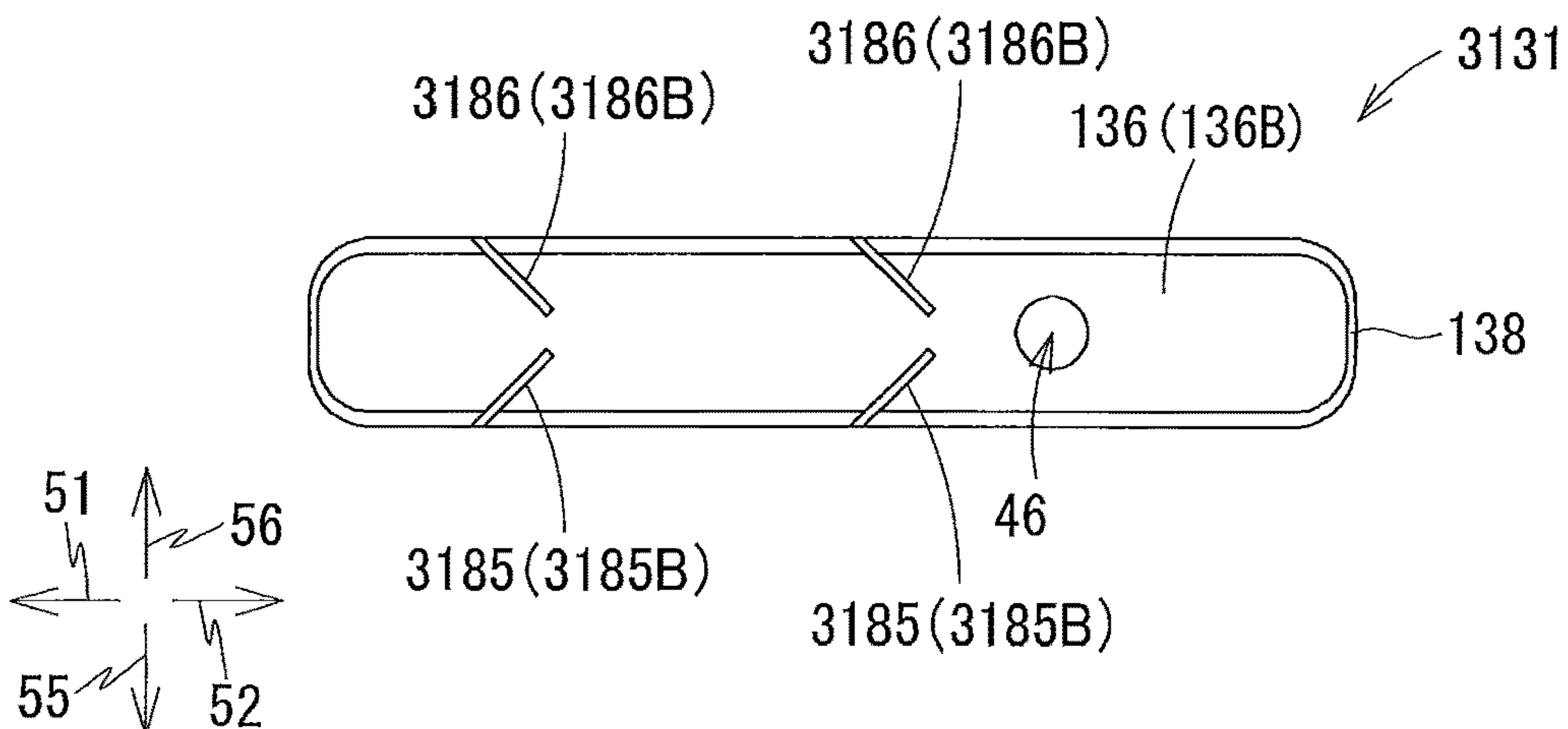
FIG. 26C
