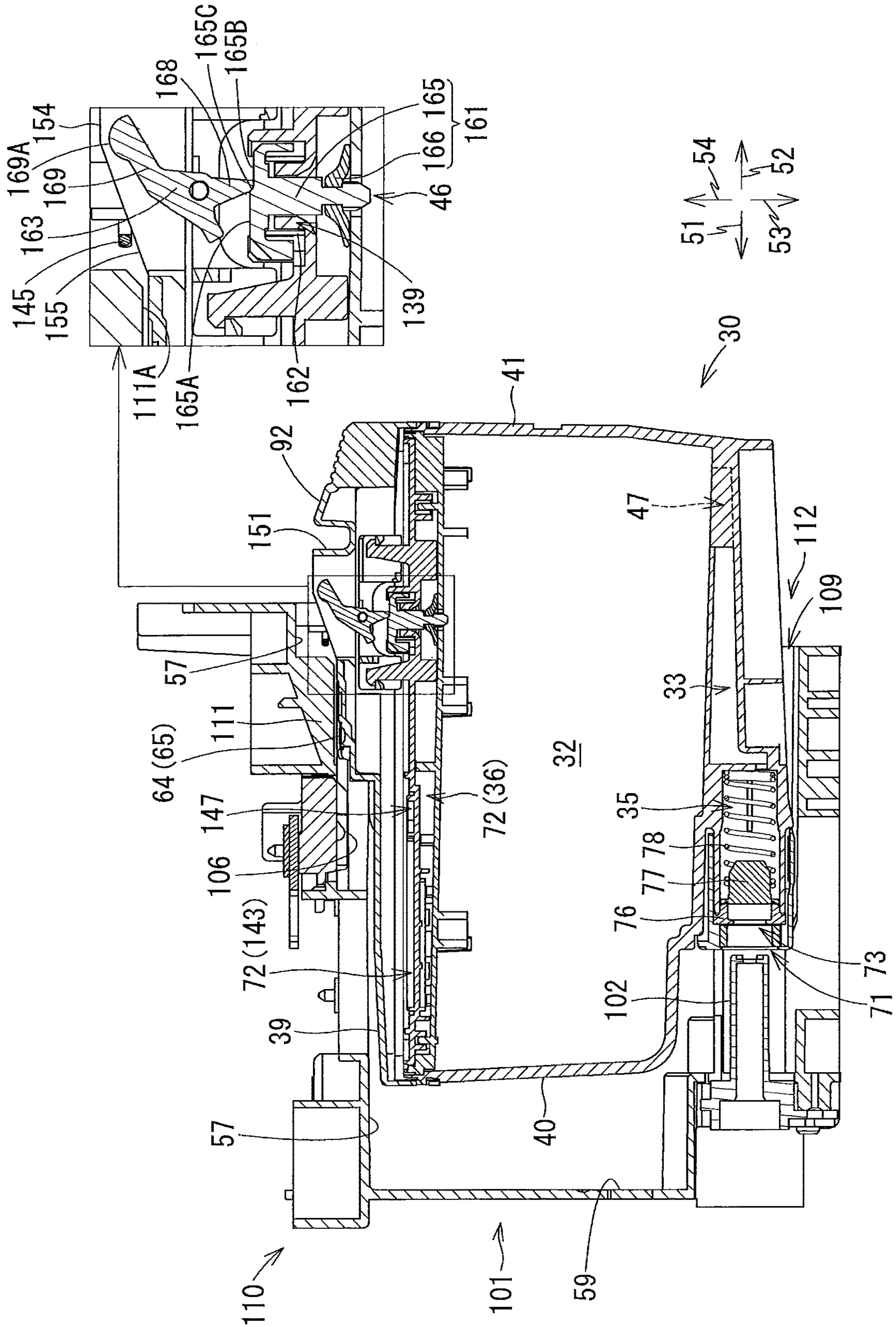
FIG. 16
