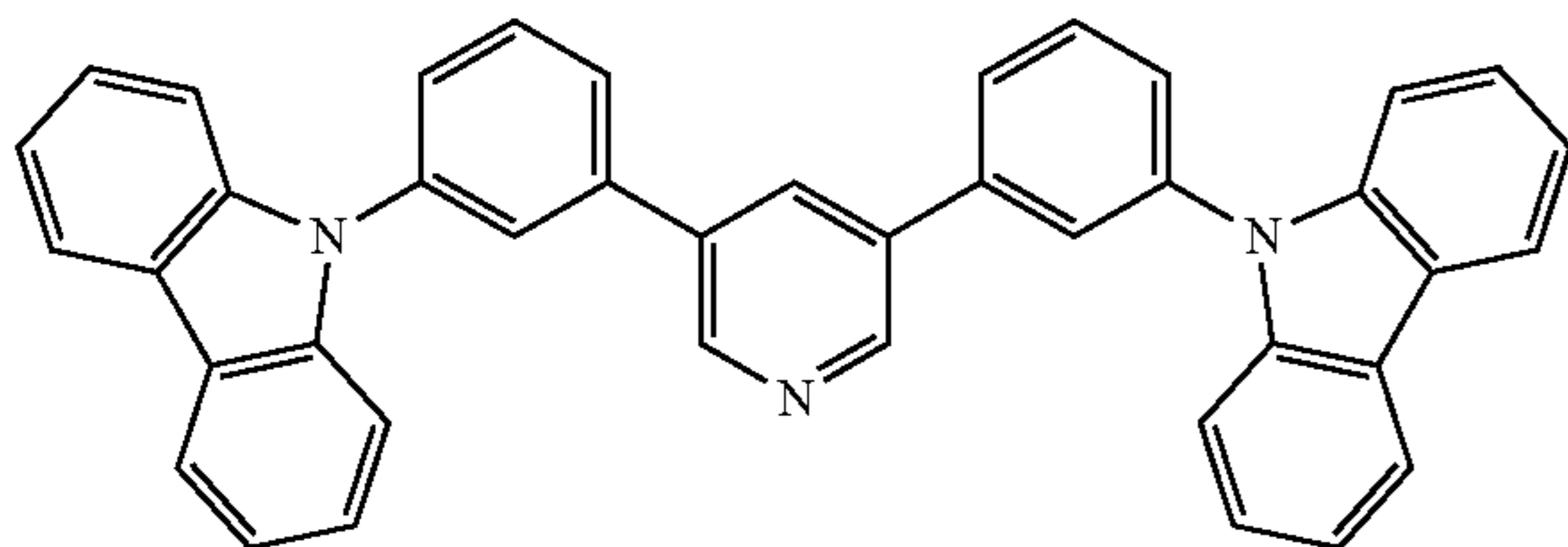
(vii) 3,5DCzPPy
