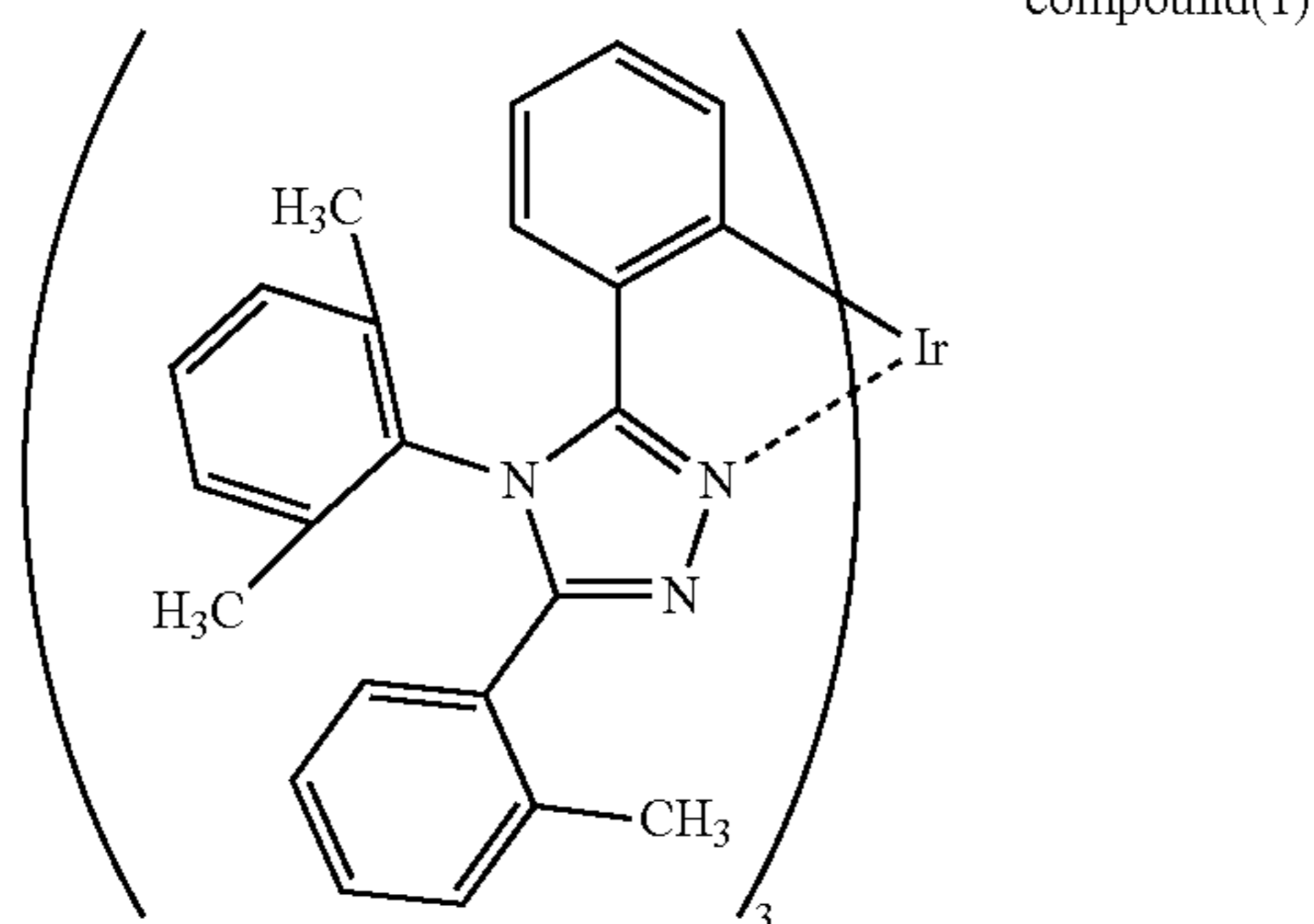
(ix) Ir(mpptz-dmp) 3
