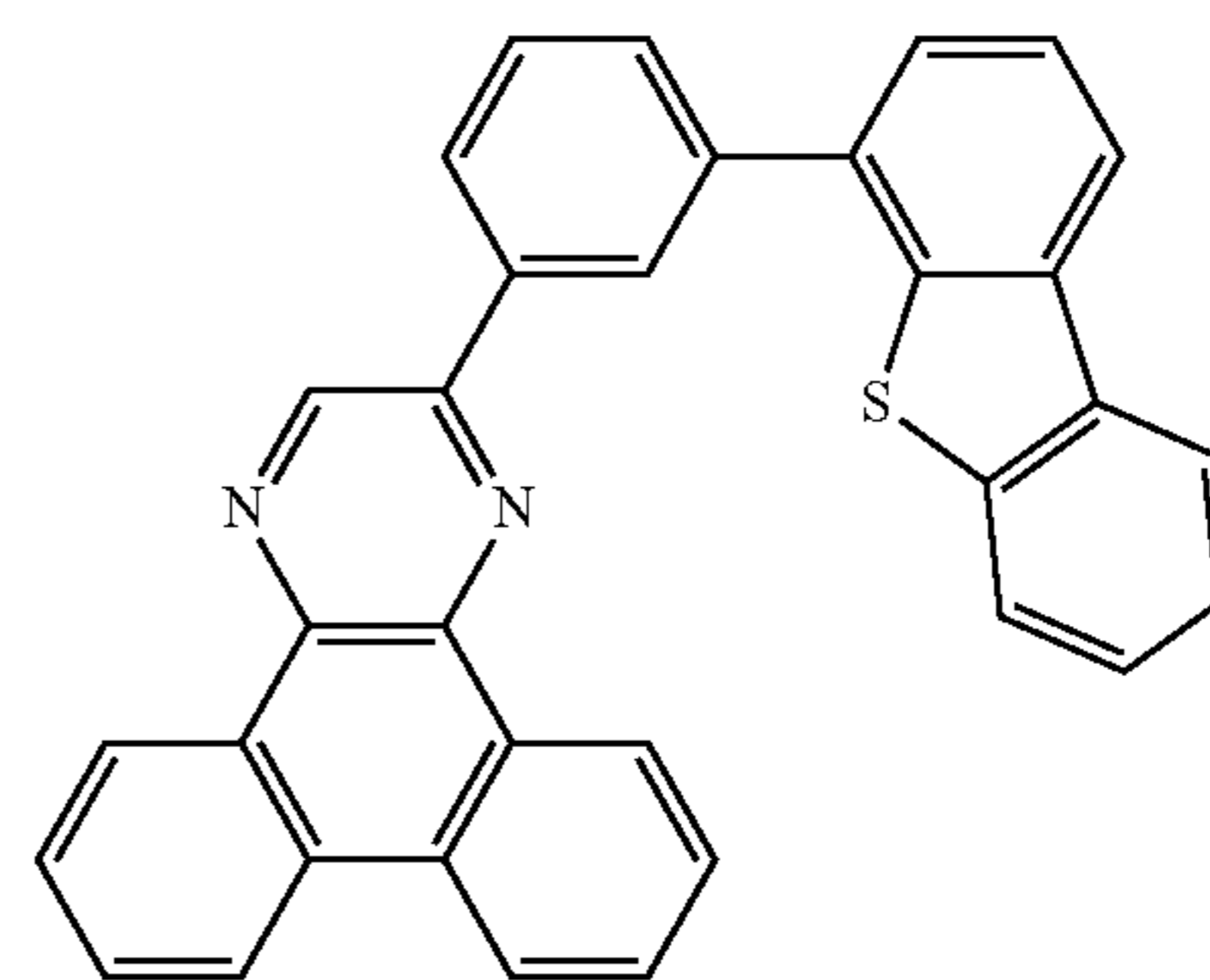
(iii) 2mDBTPDBq-II
