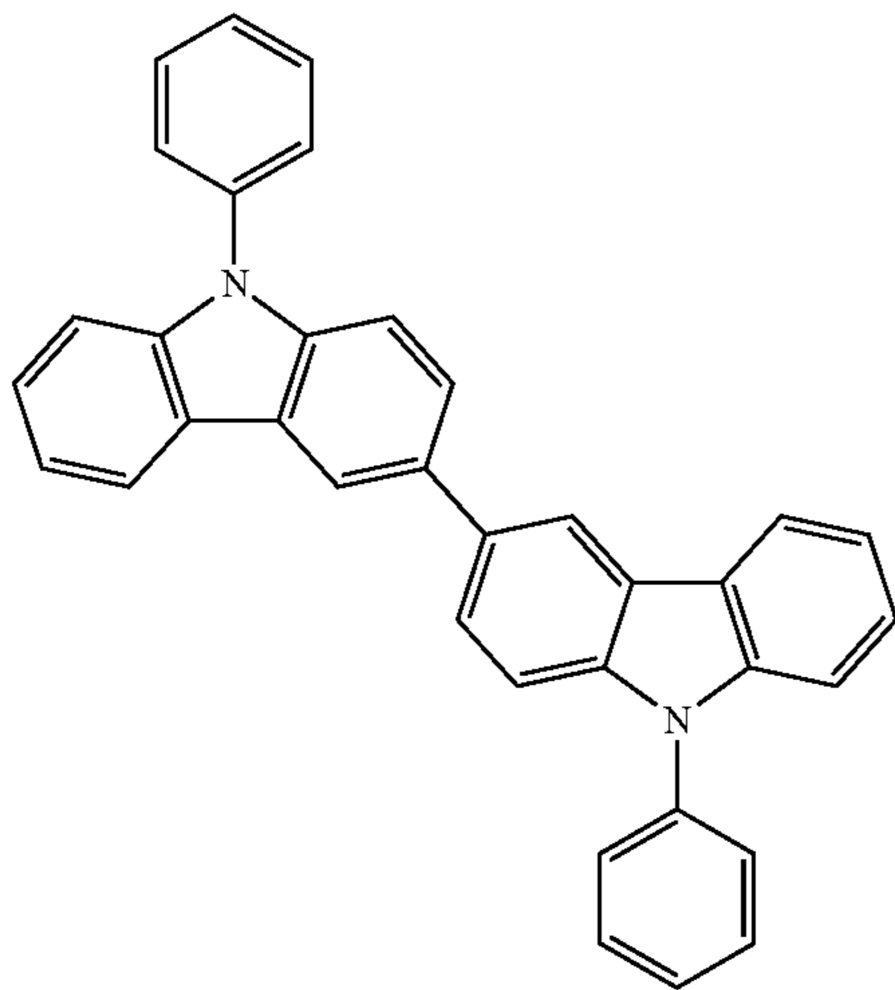
(viii) PCCP
