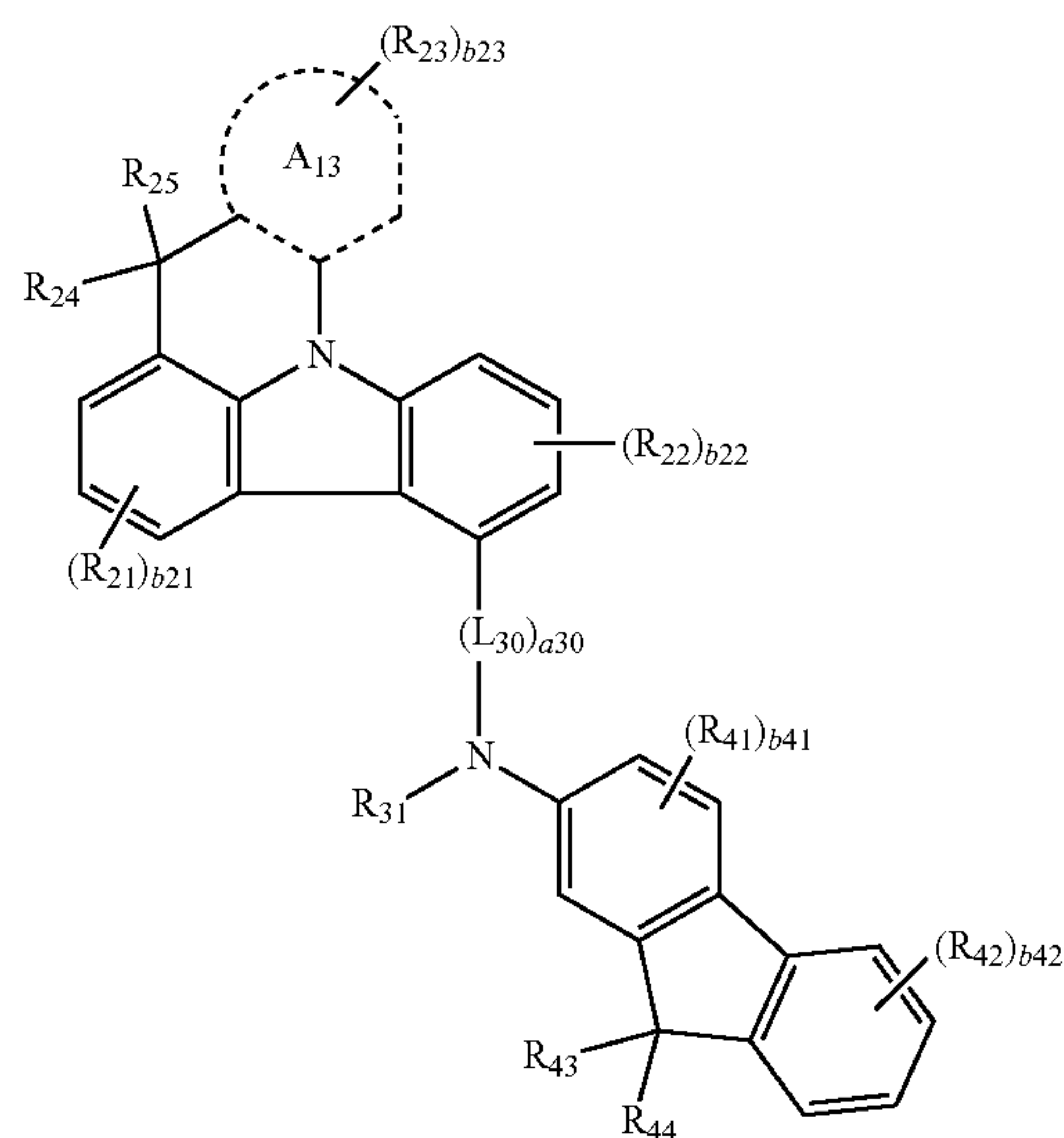
Formula 2B(16)
