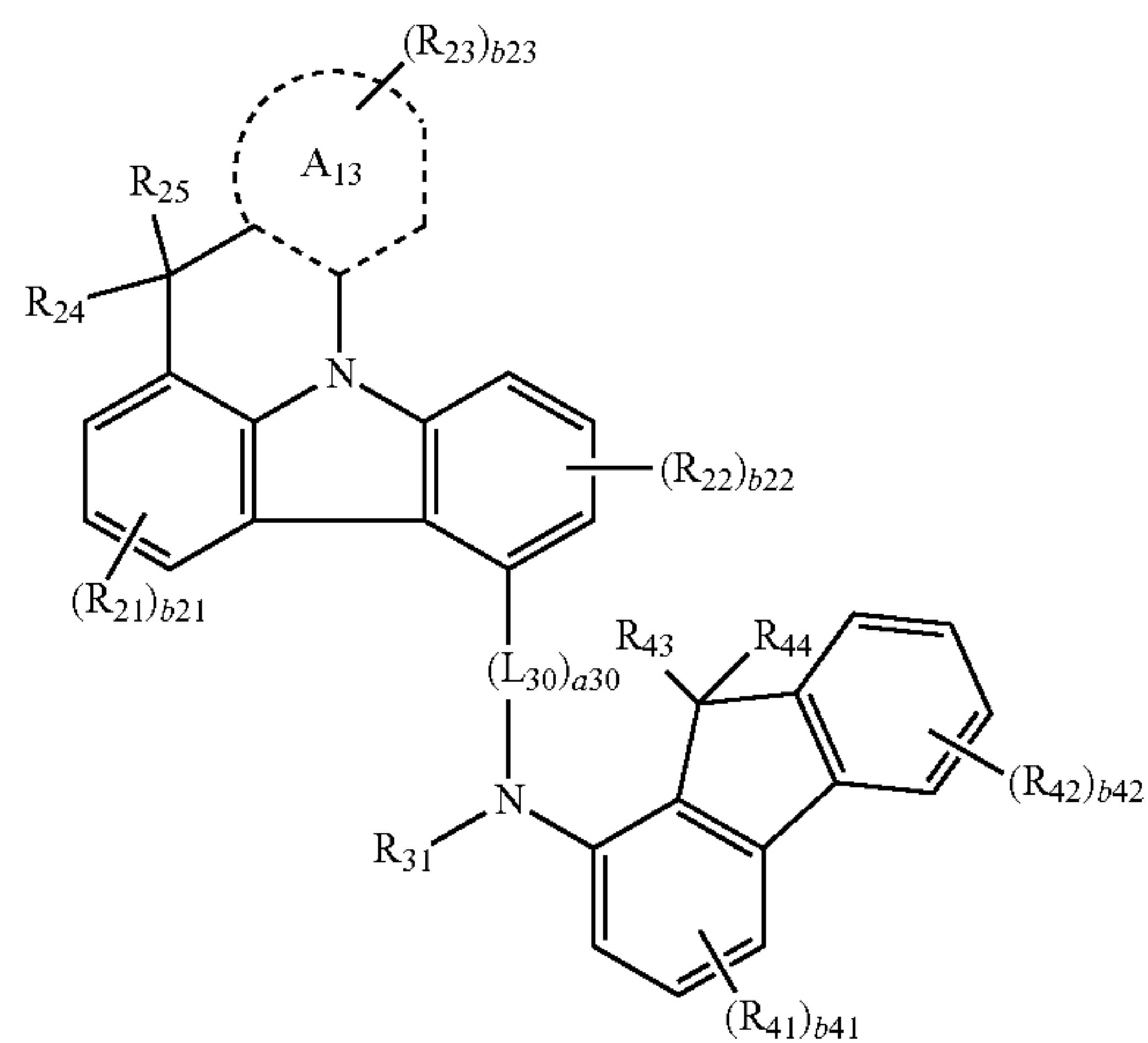
Formula 2B(16)
