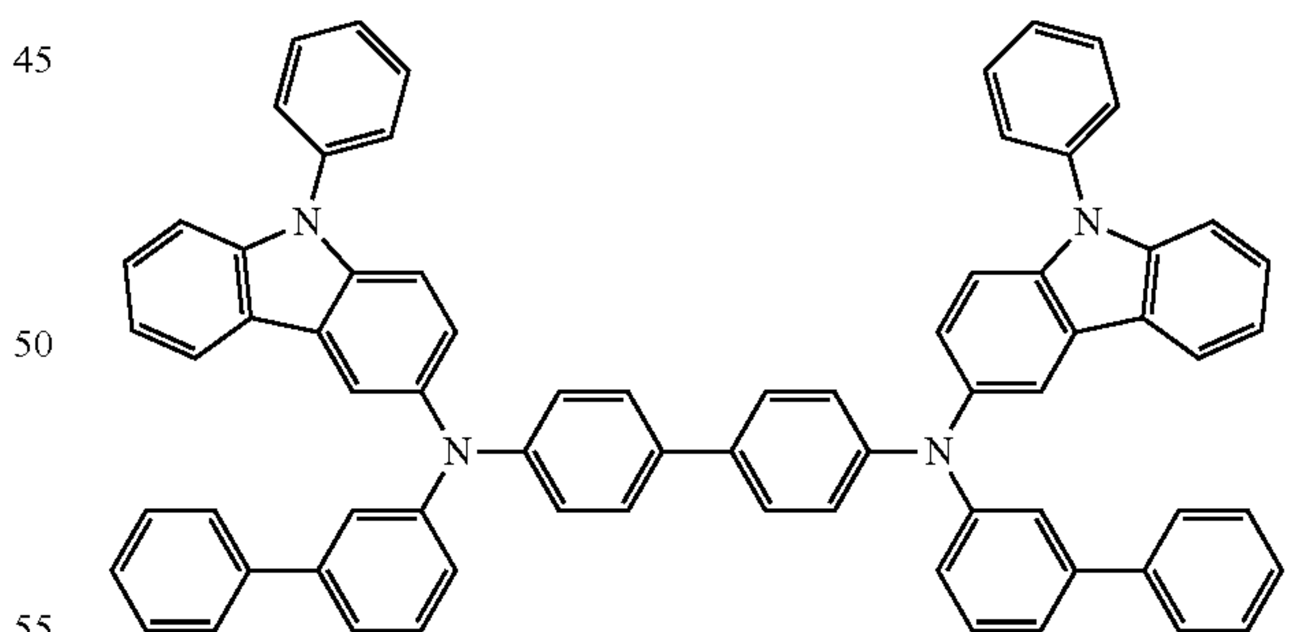
CP5
