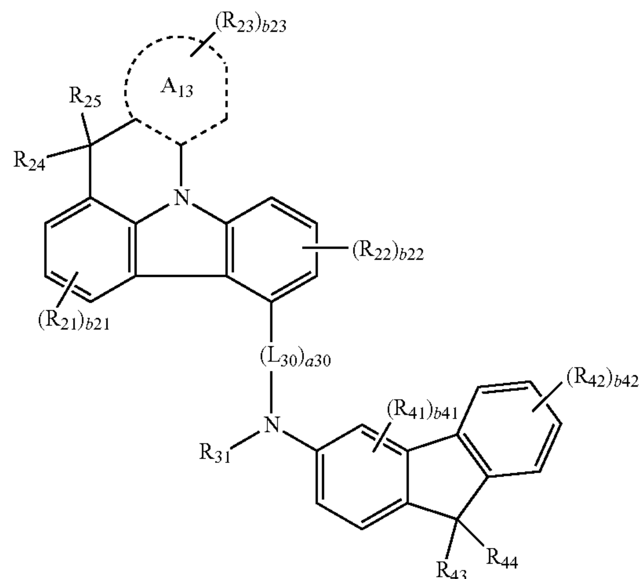
Formula 2B(15)
