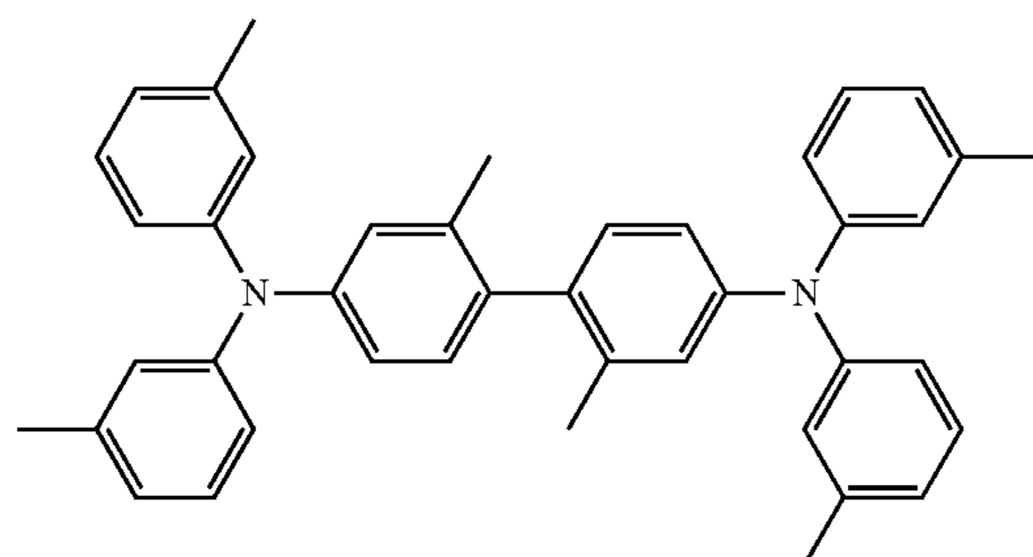
HMTPD
