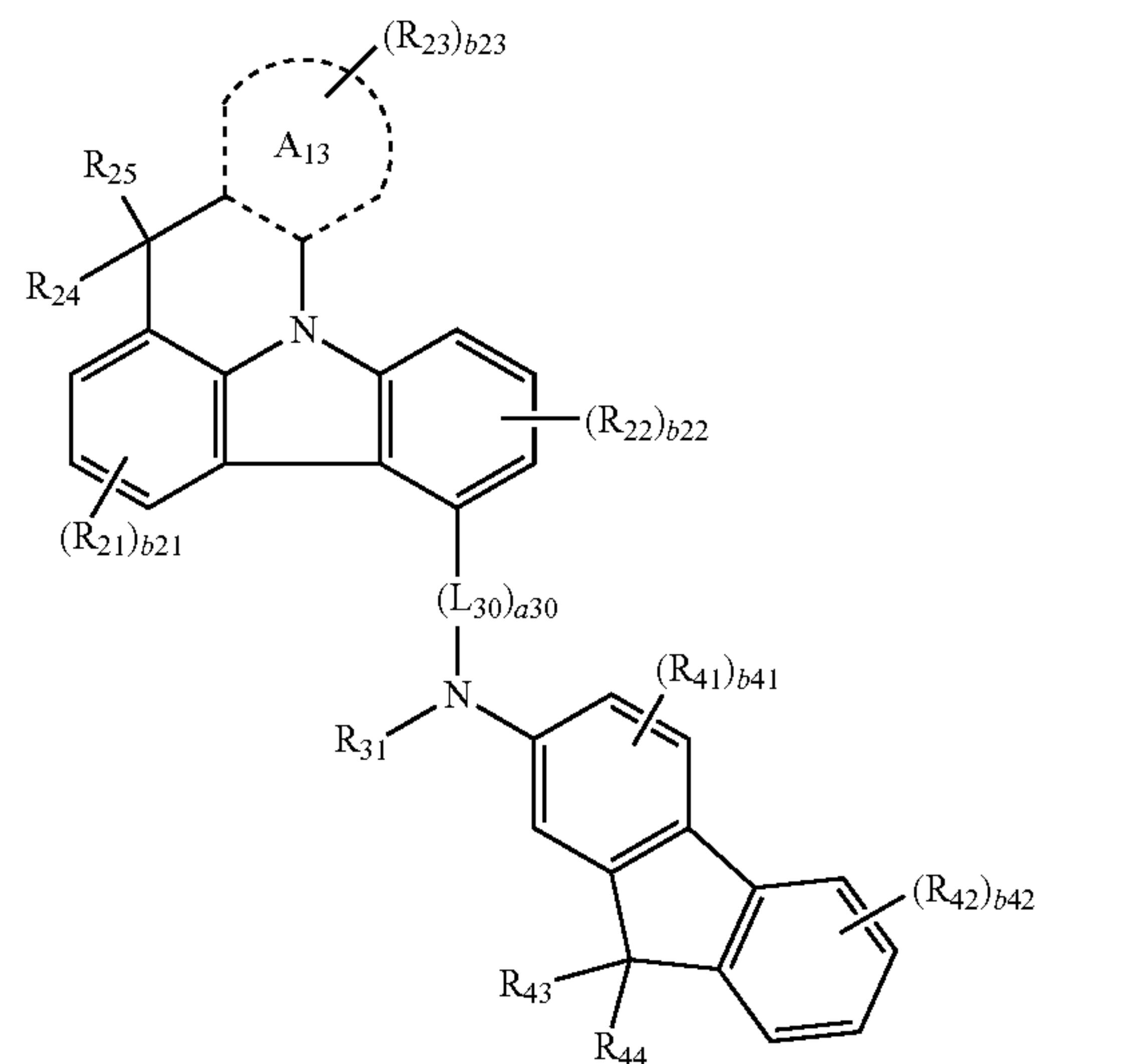
Formula 2B(16)
