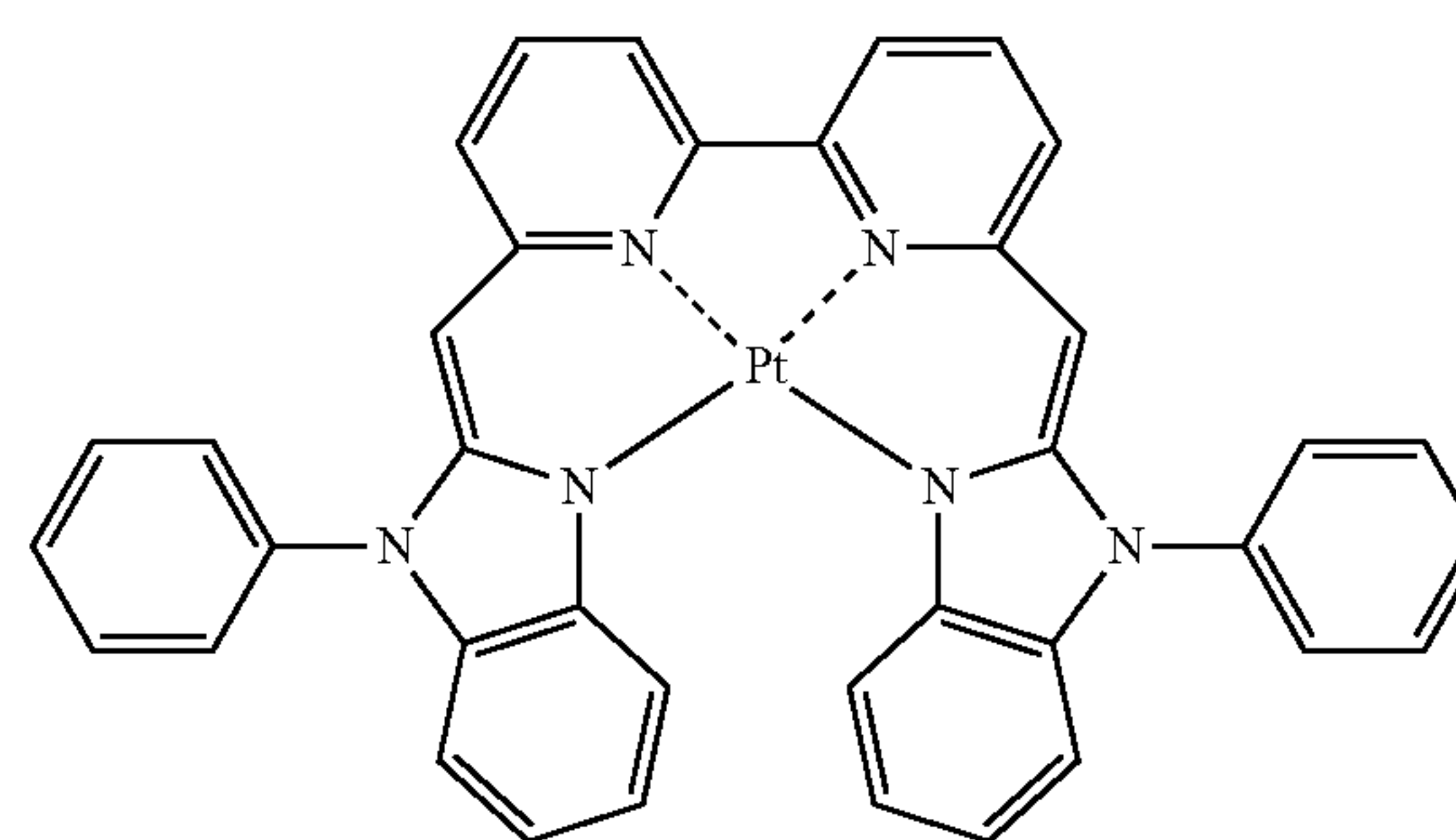
PD2
