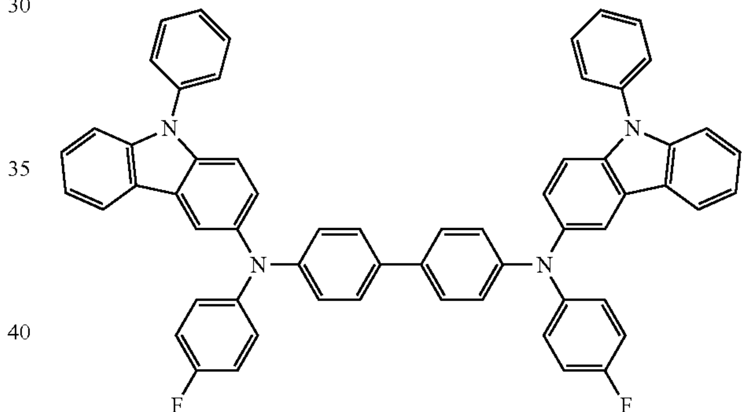
CP5
