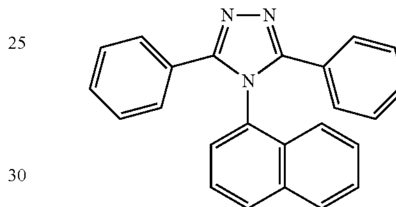
NTAZ
