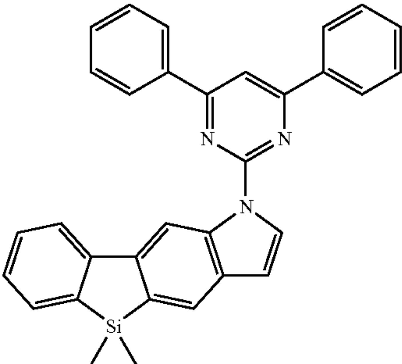
1-8
