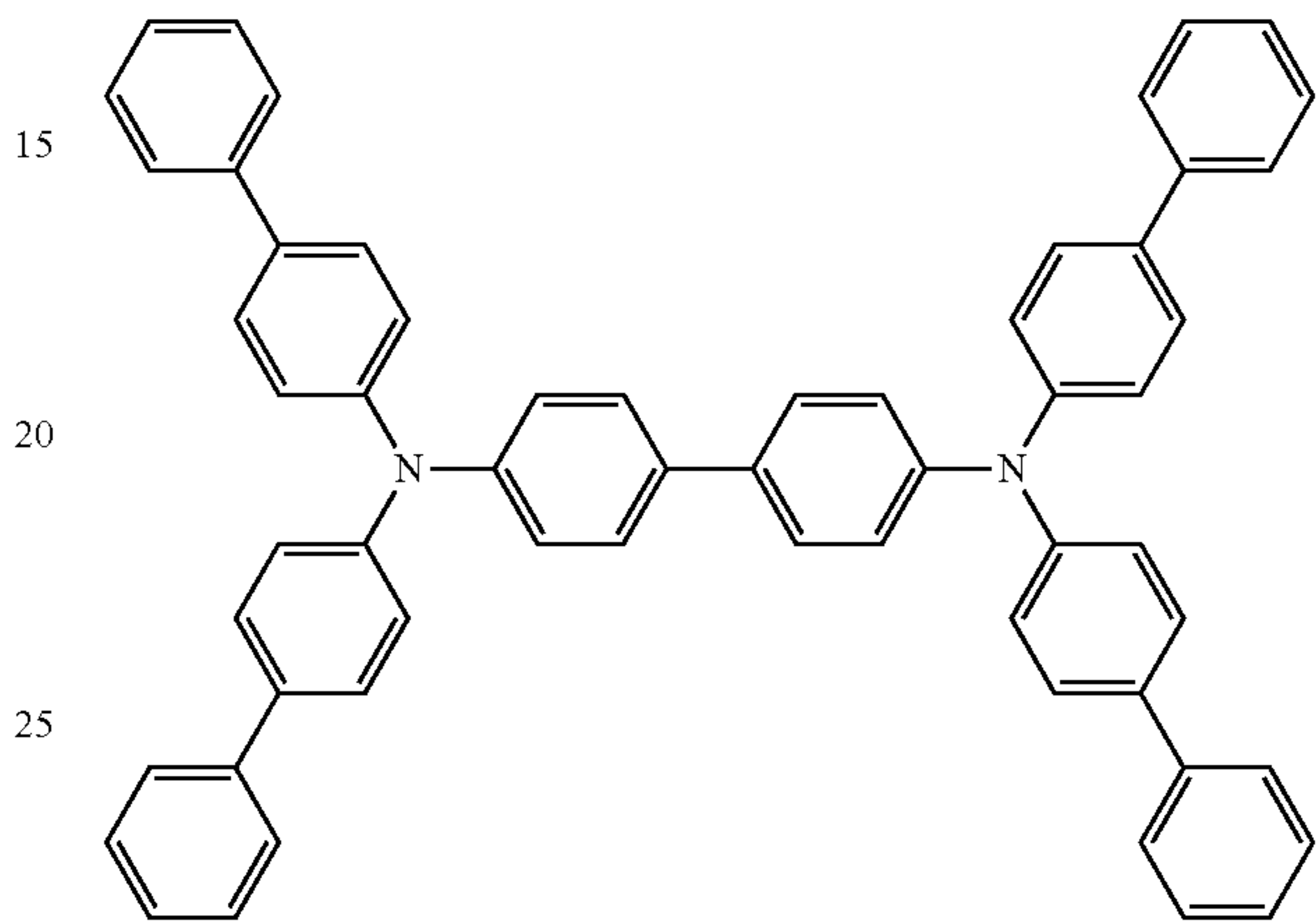
CP4
