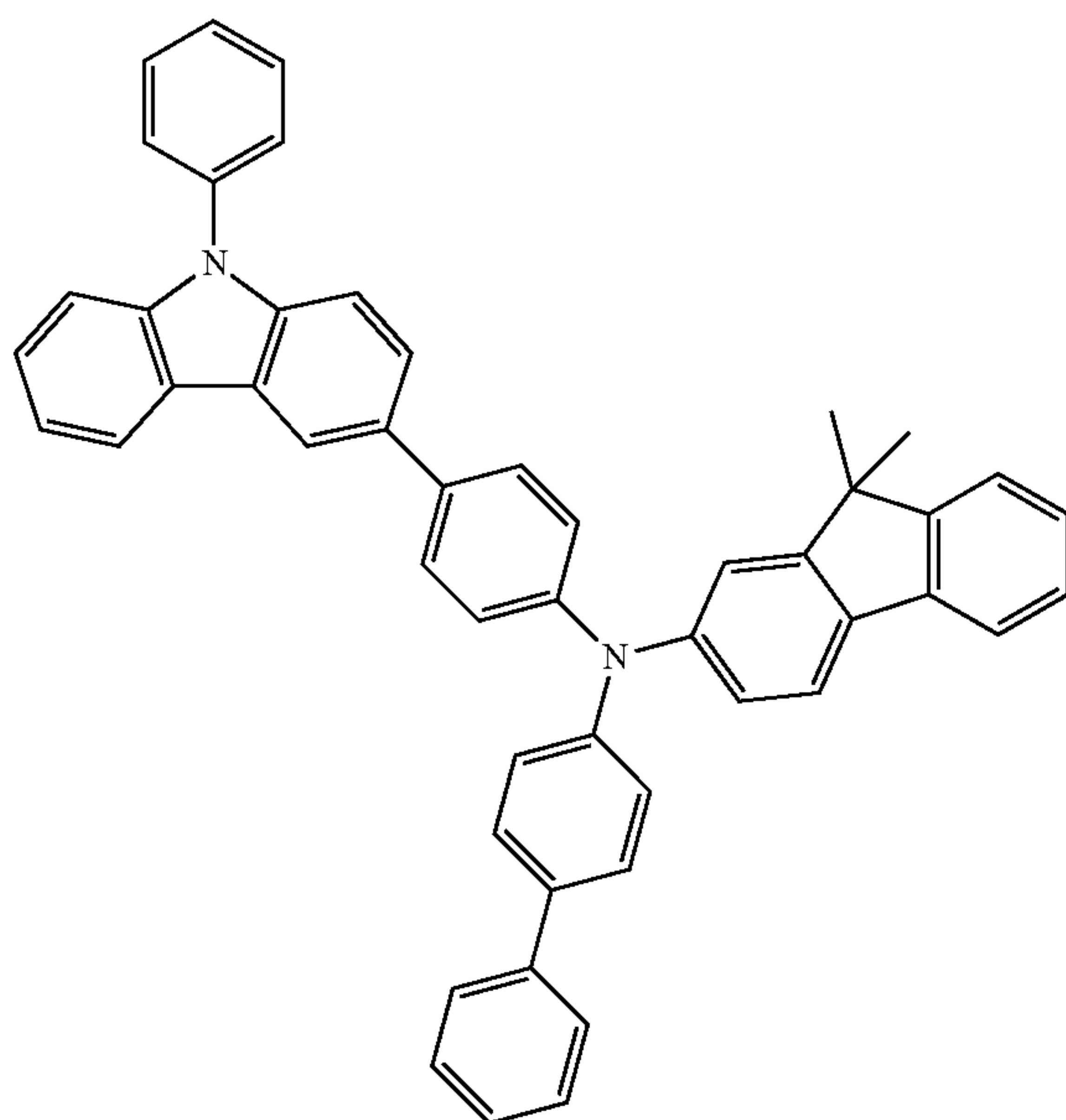
HT3
