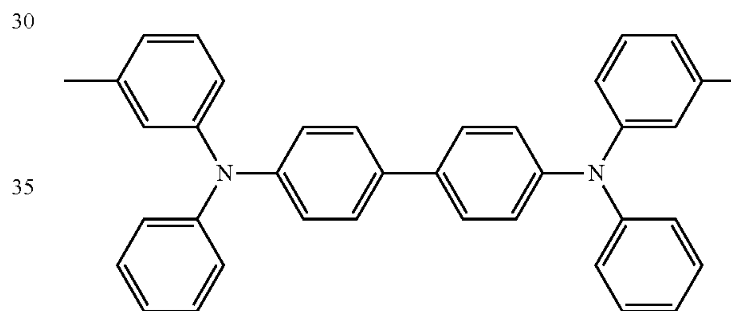
TPD
