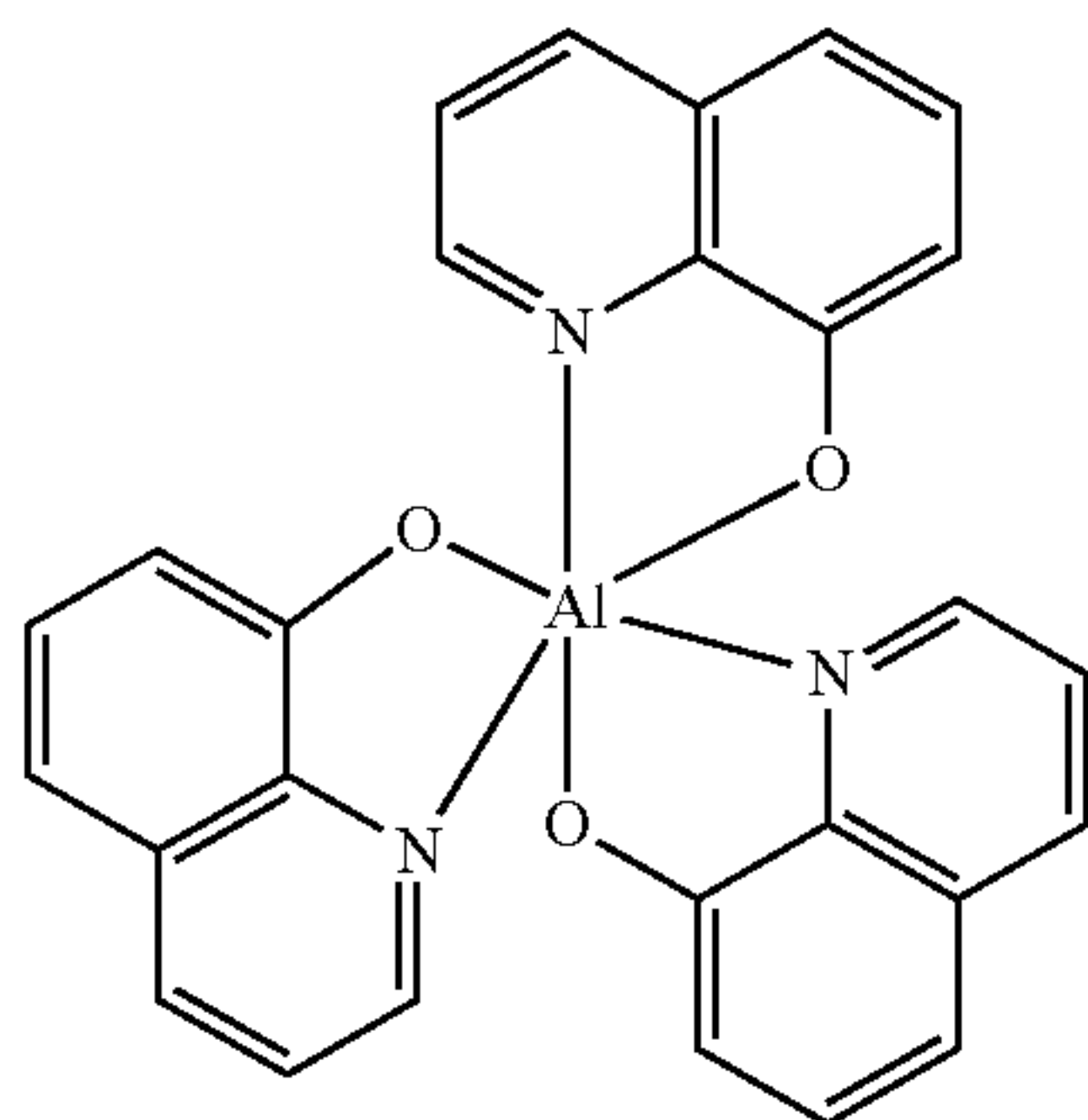
Alq 3
