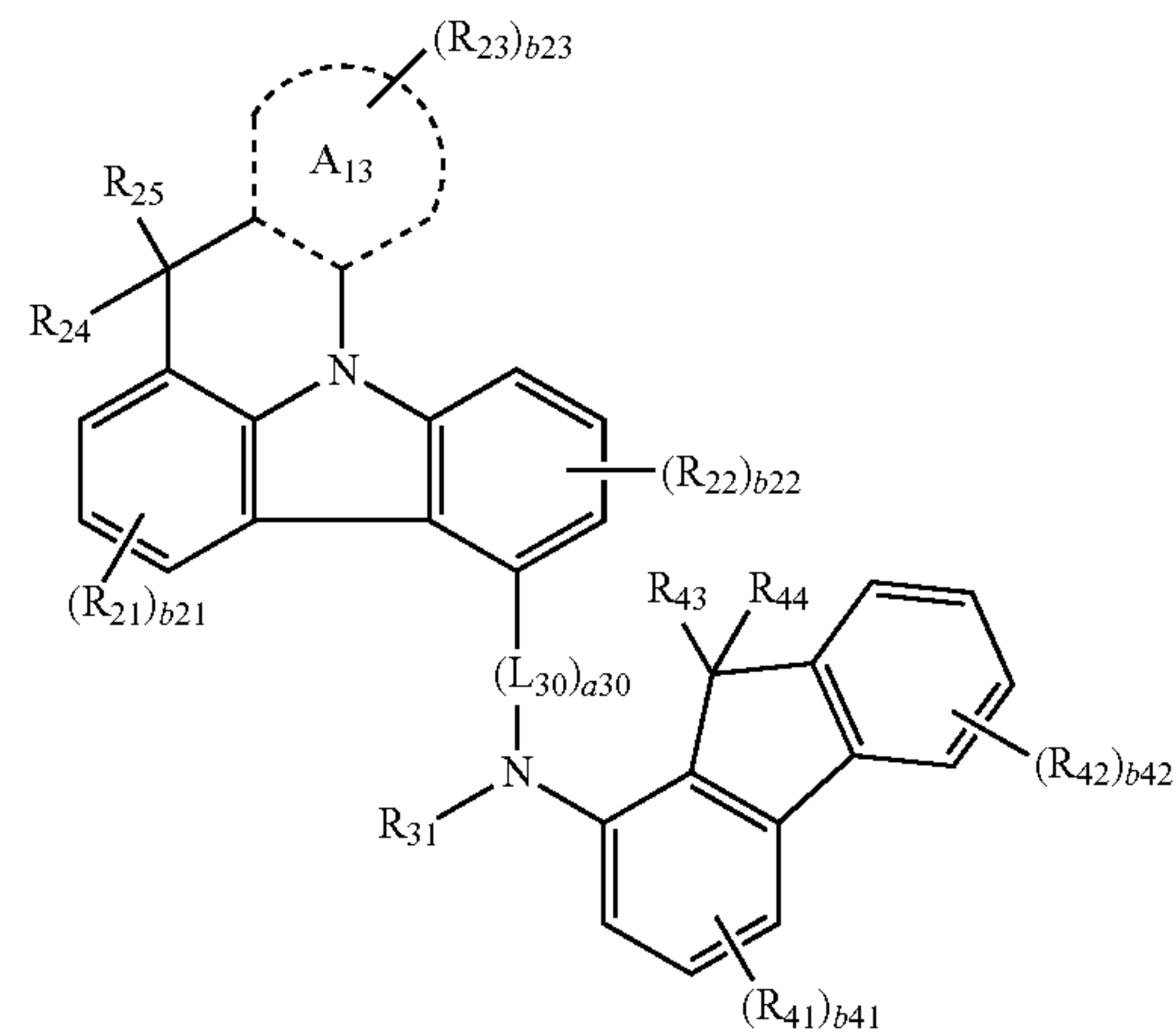
Formula 2B(16)
