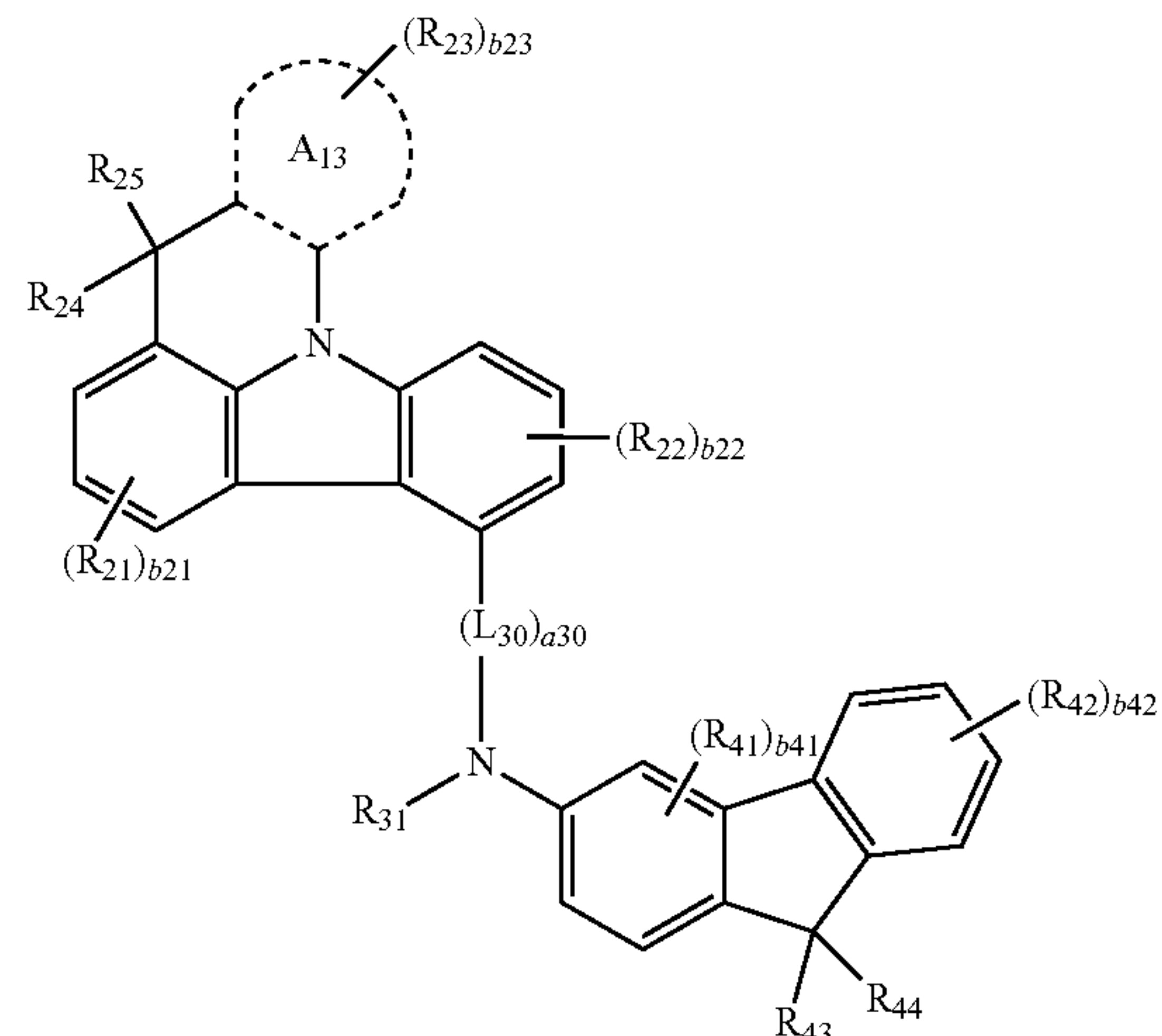
Formula 2B(15)
