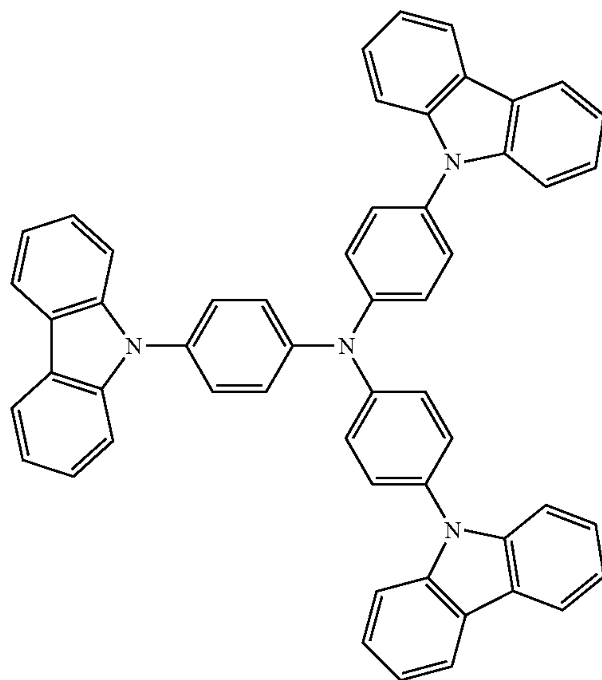
TCTA
