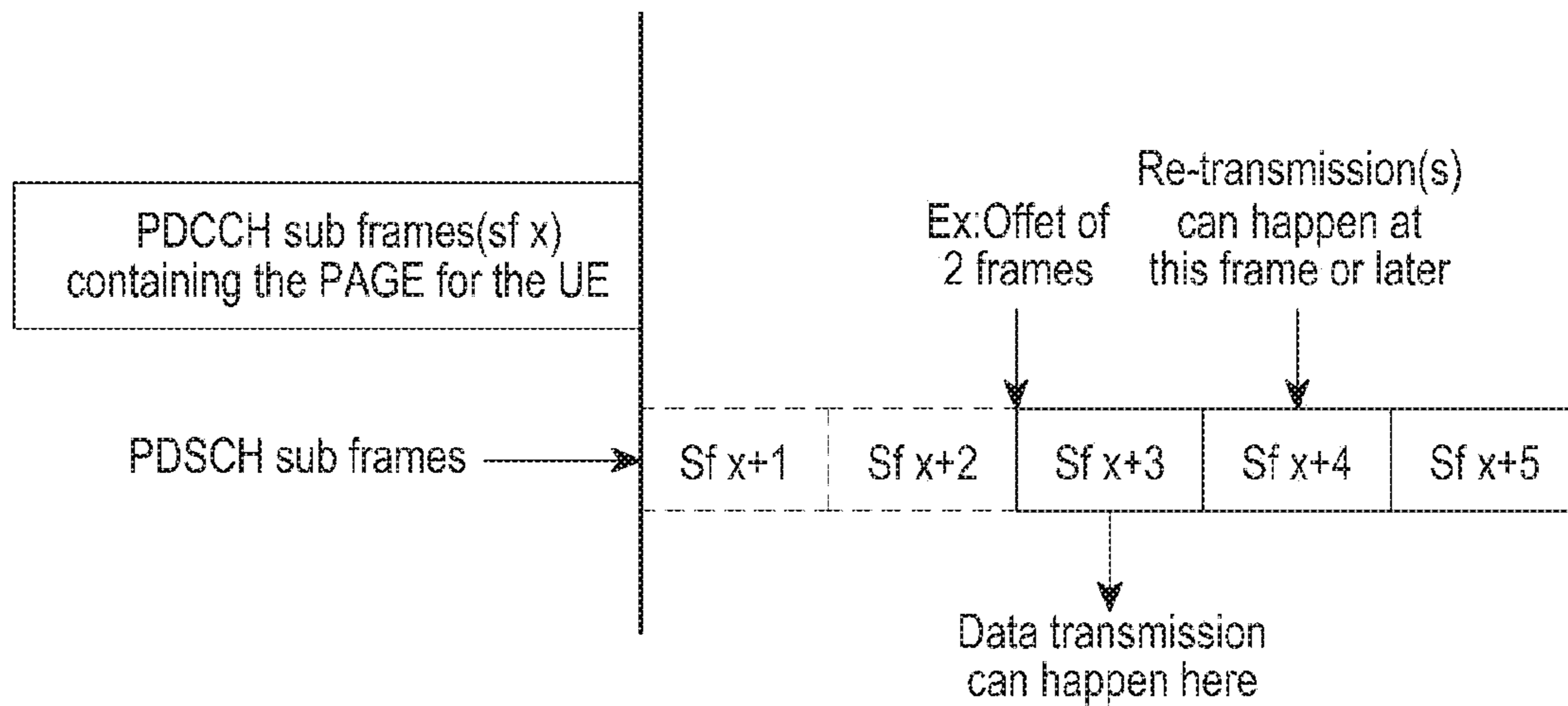
FIG.20
