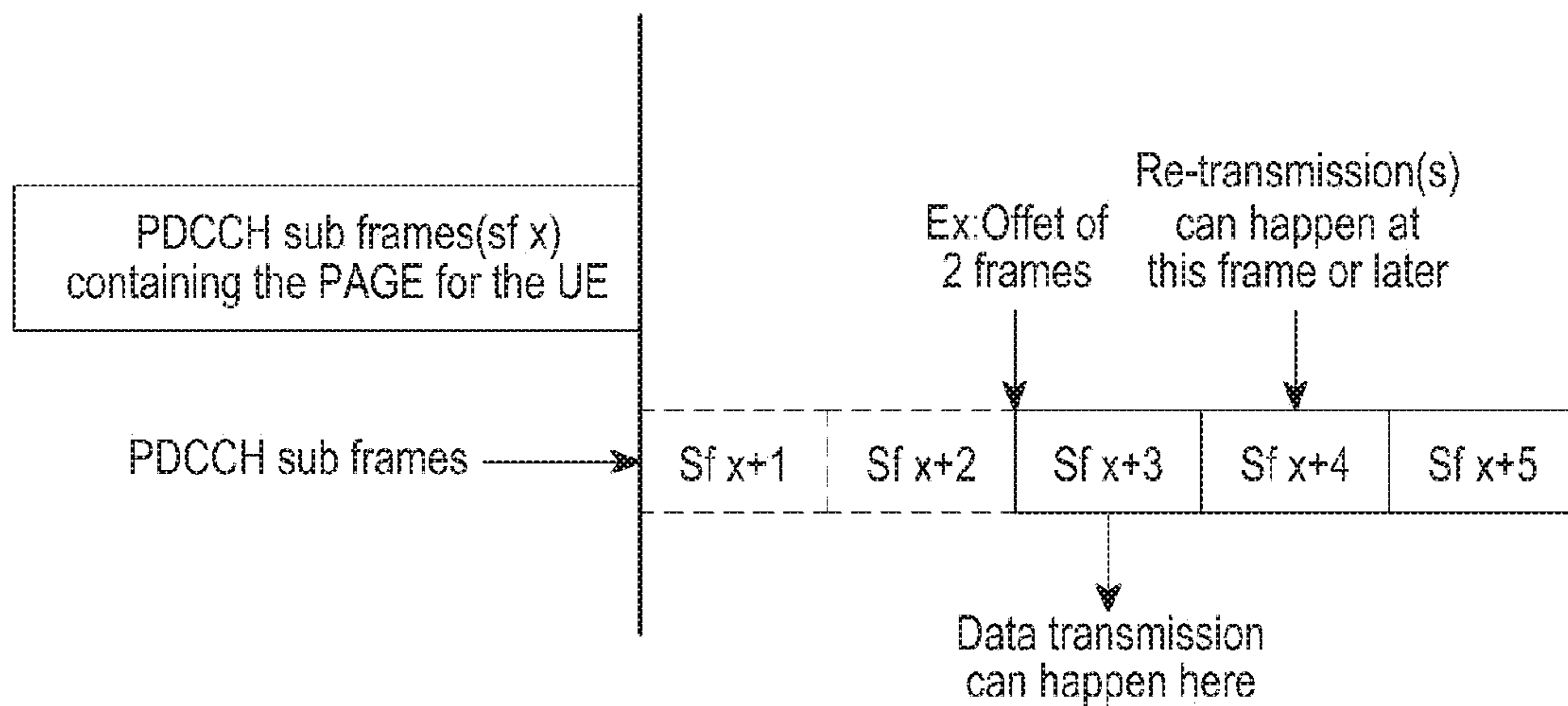
FIG.21
