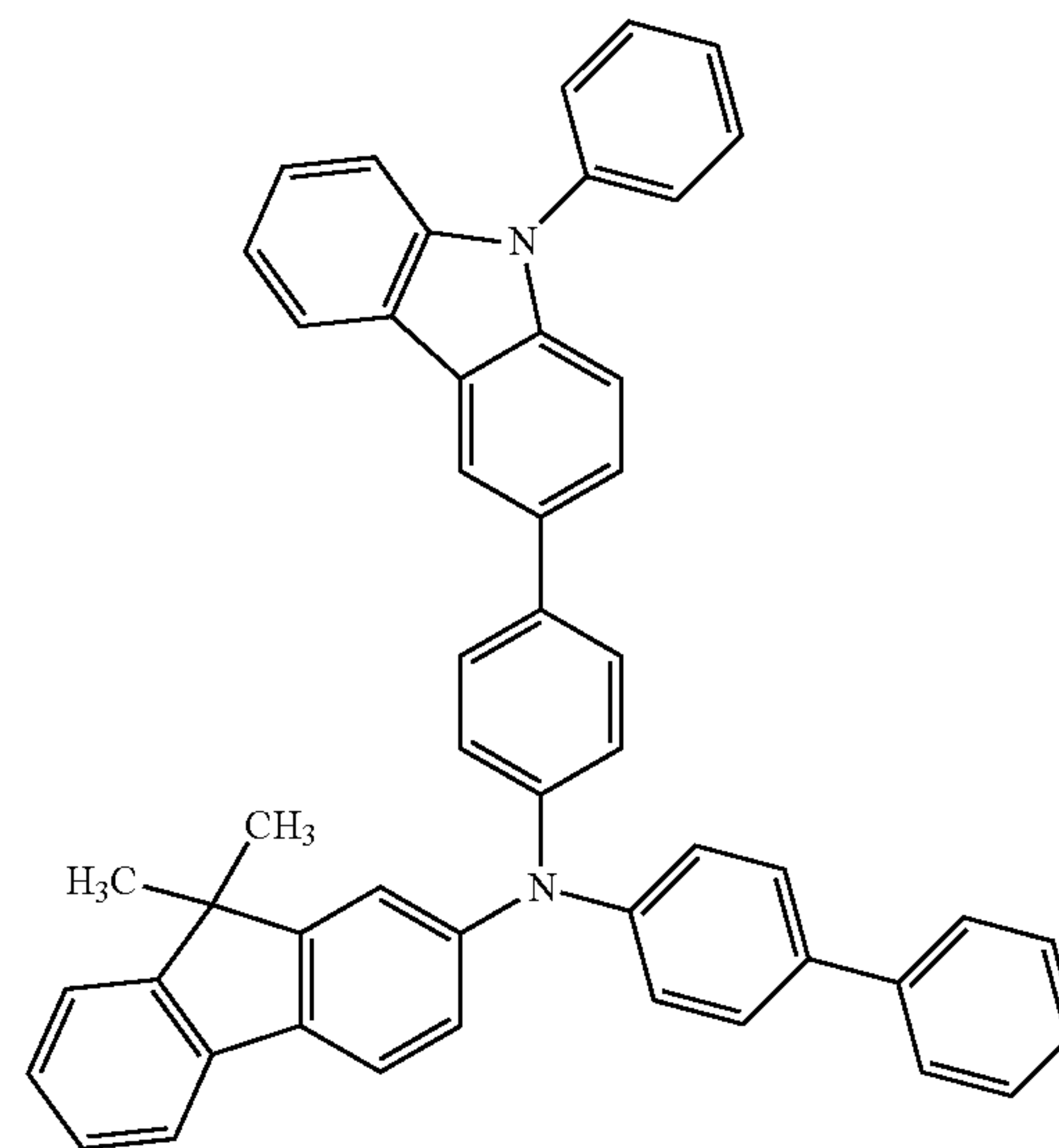
PCBBiF
