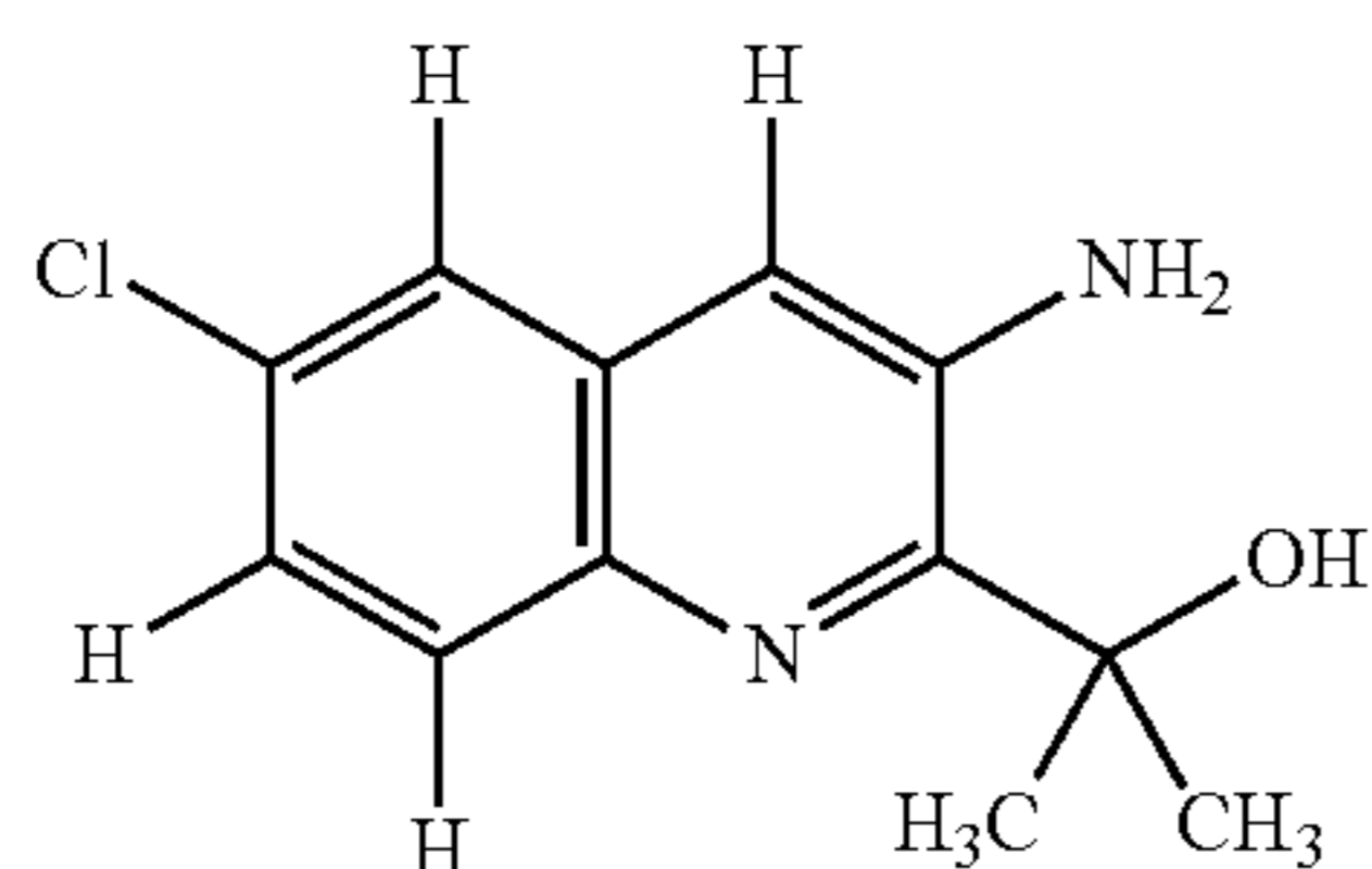
2-(3-amino-6-chloroquinolin-2-yl)propan-2-ol
