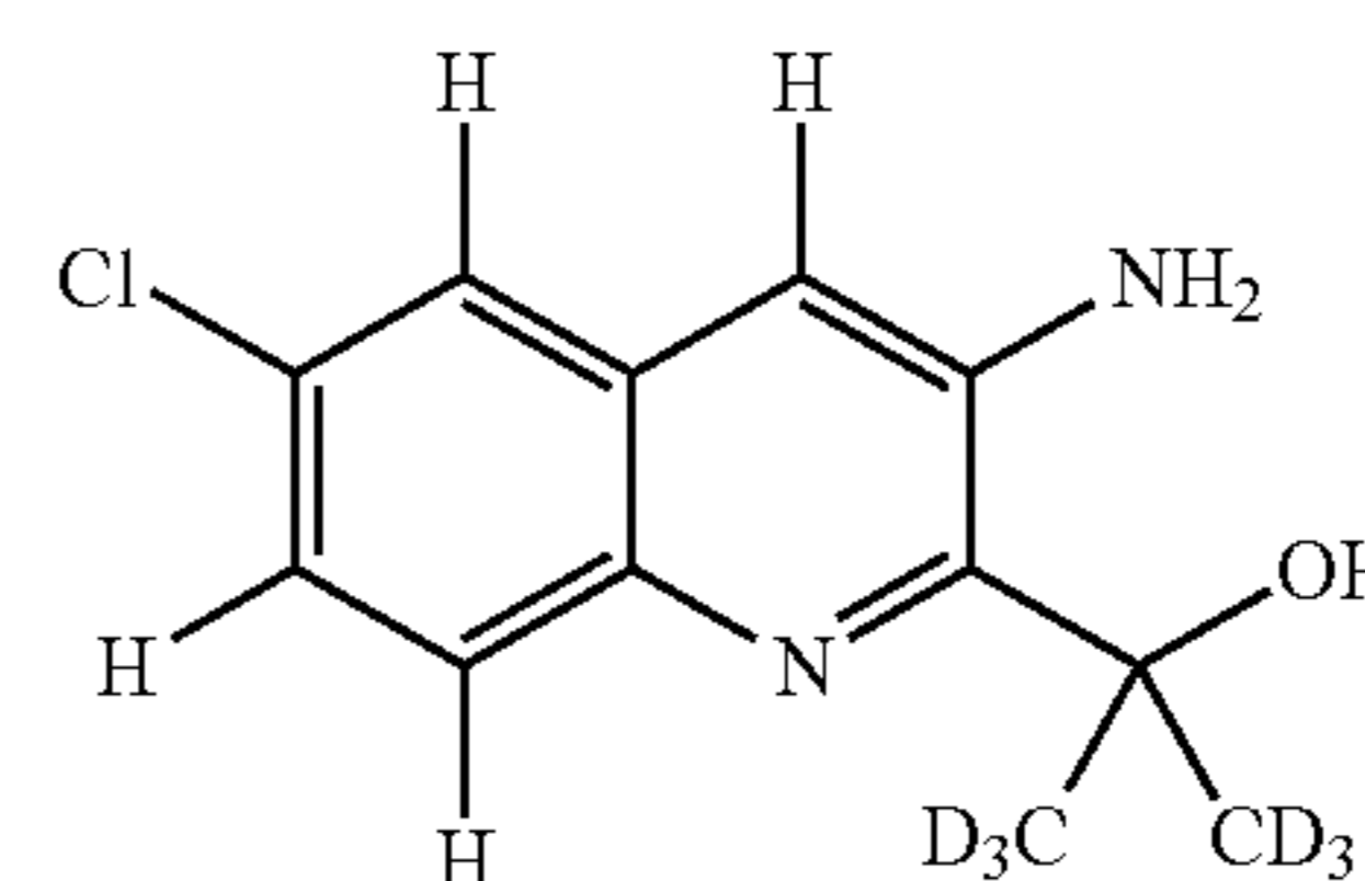
2-(6-chloroquinolin-2-yl)propan-1,1,1,3,3,3-d 6 -2-ol
