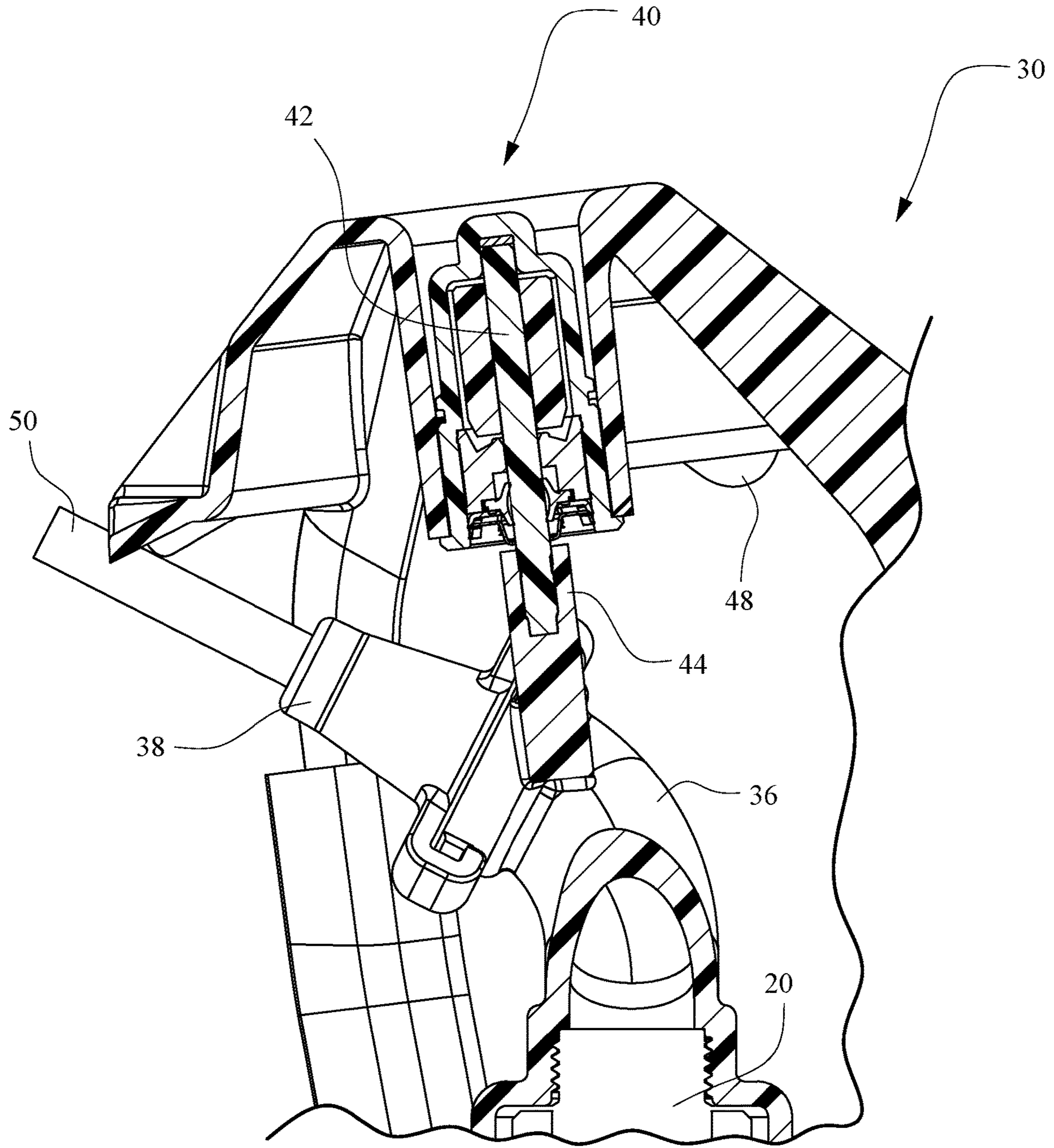
Fig. 6
