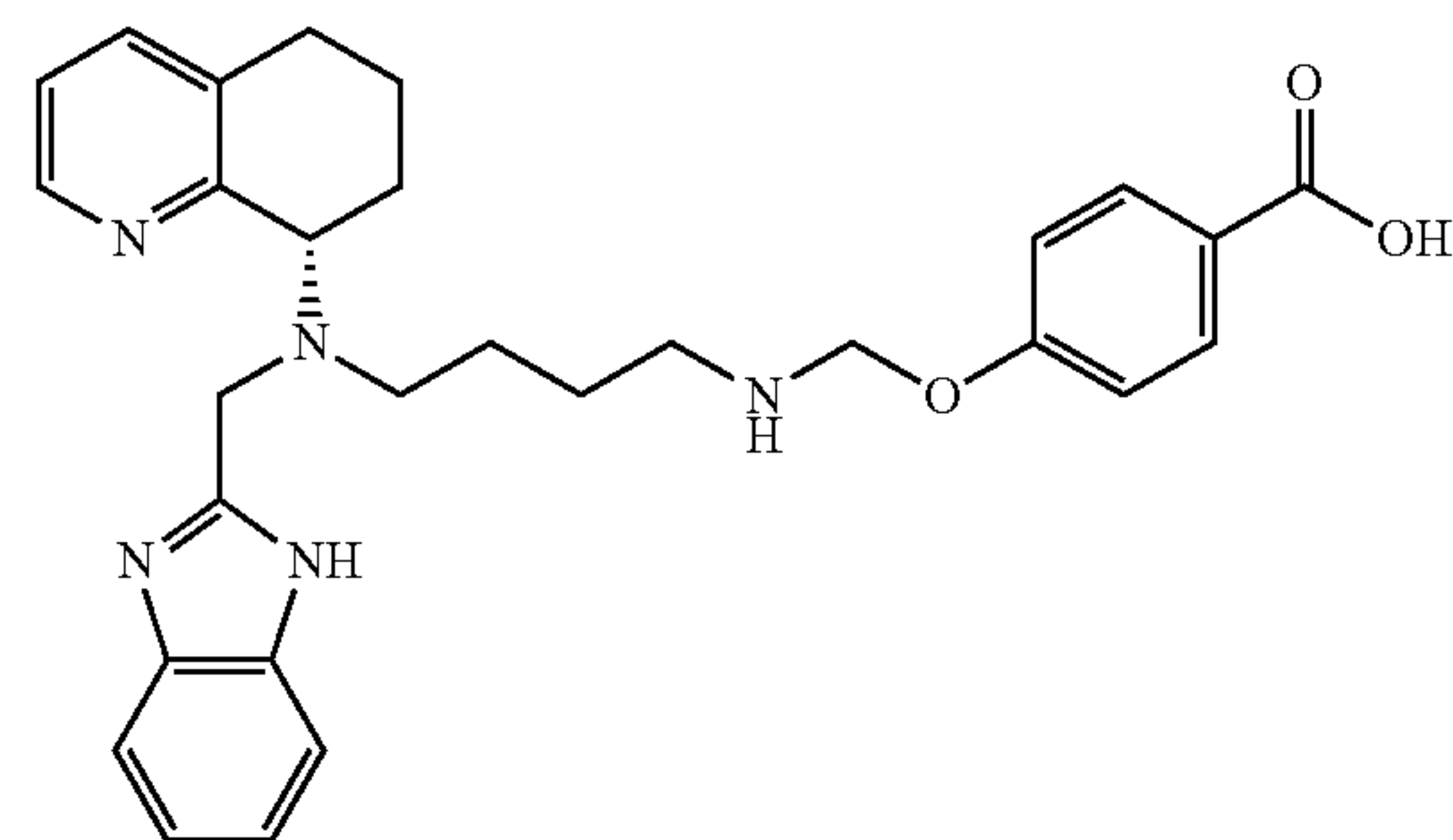
(S)-4-(((4-(((1H-benzo[d]imidazol-2-yl)methyl)(5,6,7,8-tetrahydroquinolin-8-yl)amino)butyl)amino)methoxy)benzoic acid
