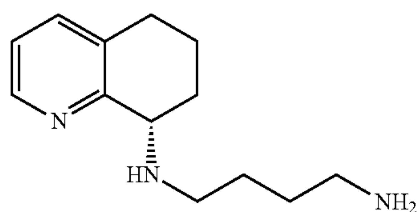
de-Boc-NT-316 F
