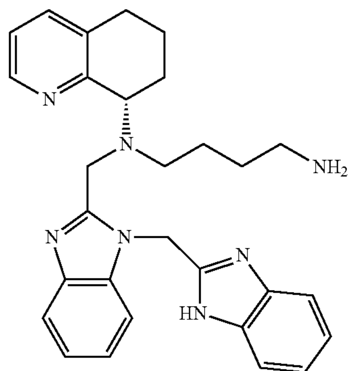
benzimidazole E
