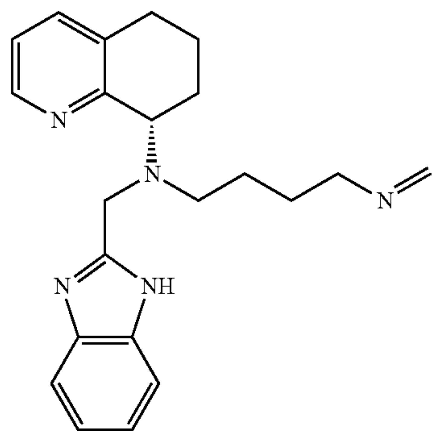
(S)-N-((1H-benzo[d]imidazol-2-yl)methyl)-N-(4-(methyleneamino)butyl)-5,6,7,8-tetrahydroquinolin-8-amine
