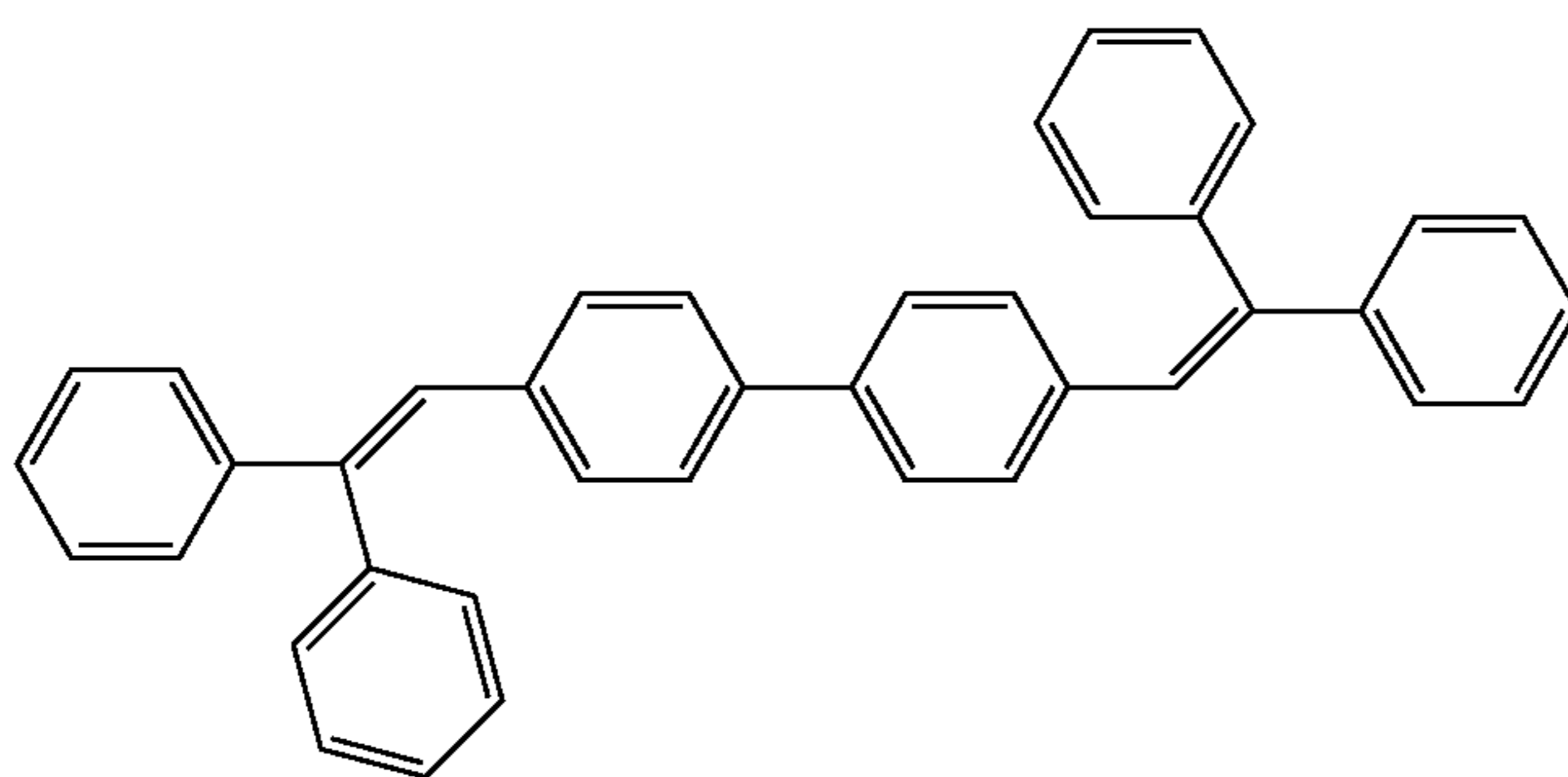
DPAVBi
