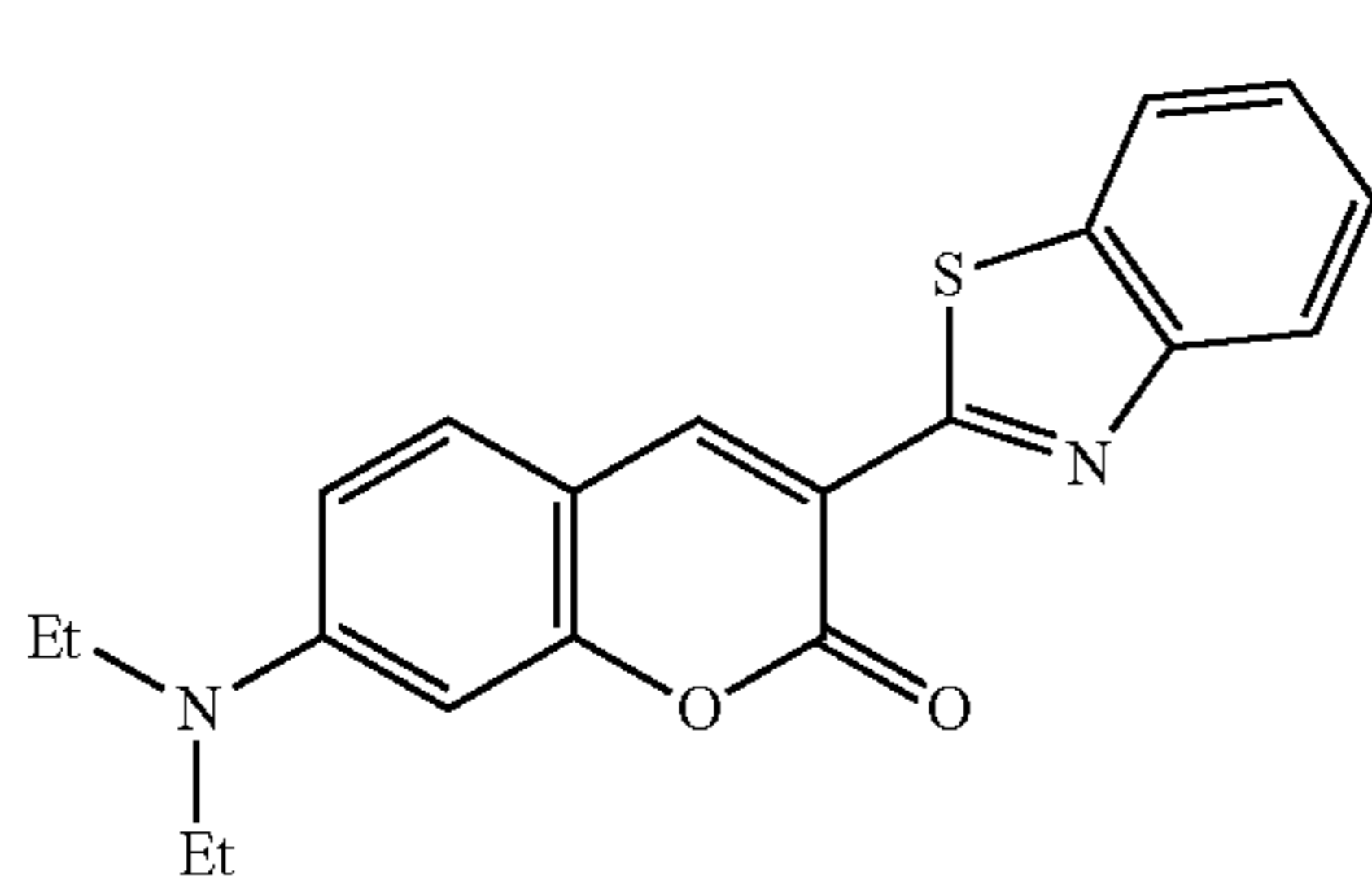
Coumarin 6
