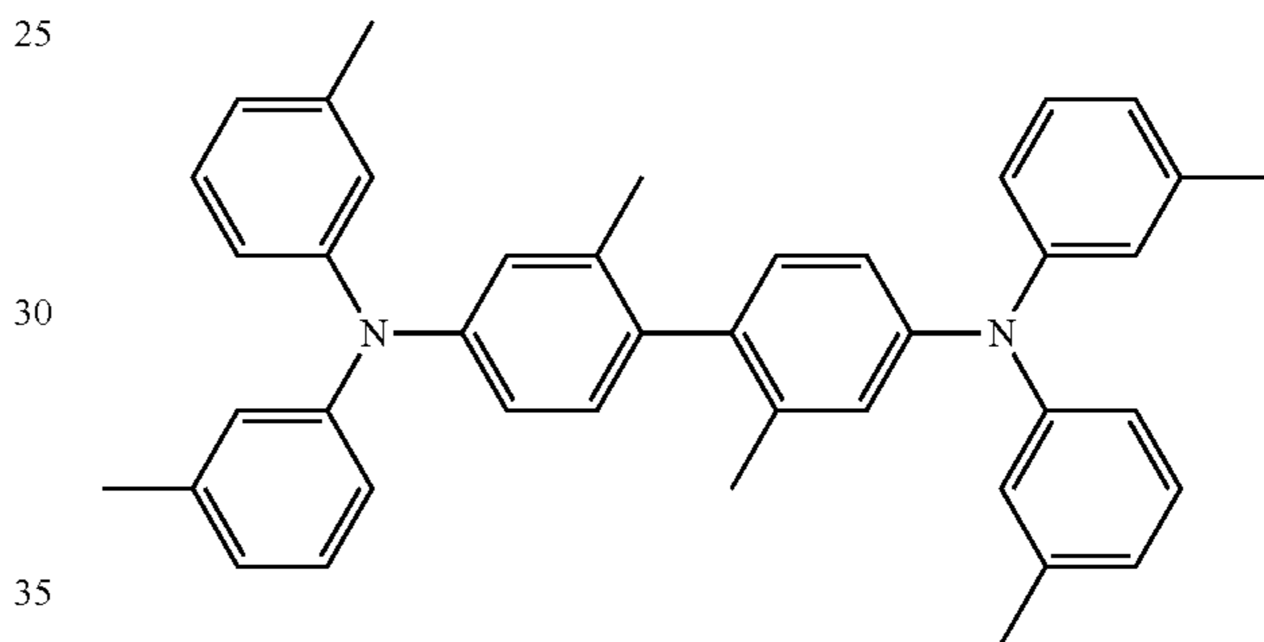
HMTPD
