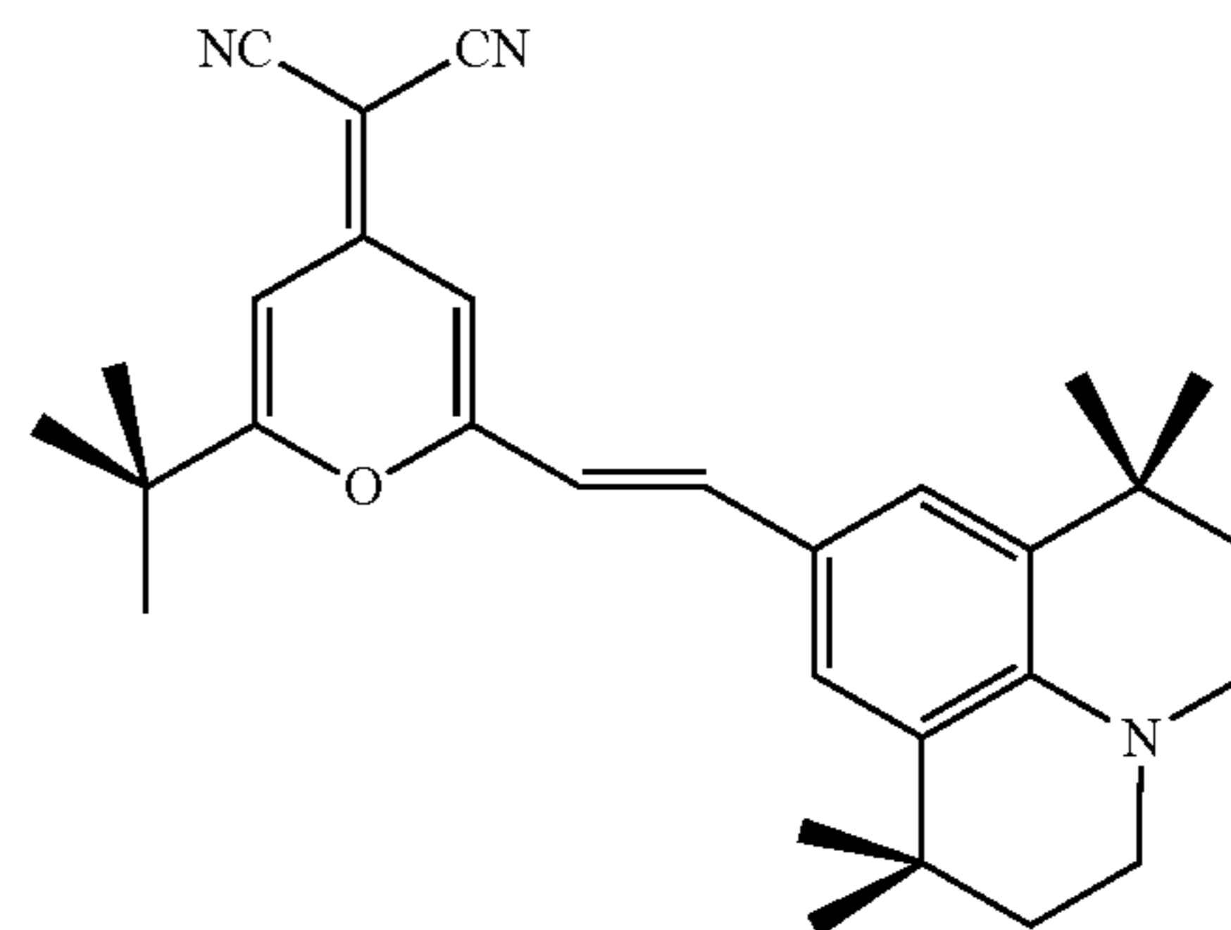
DCJTb
