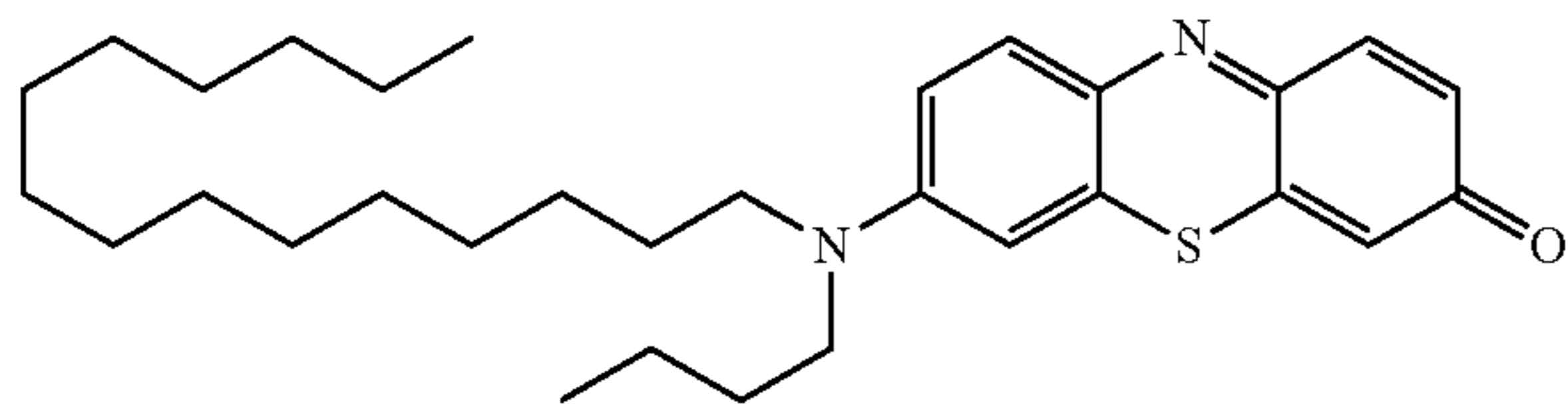
7-(butyl(pentadecyl)amino)-3H-phenothiazin-3-one (33)
