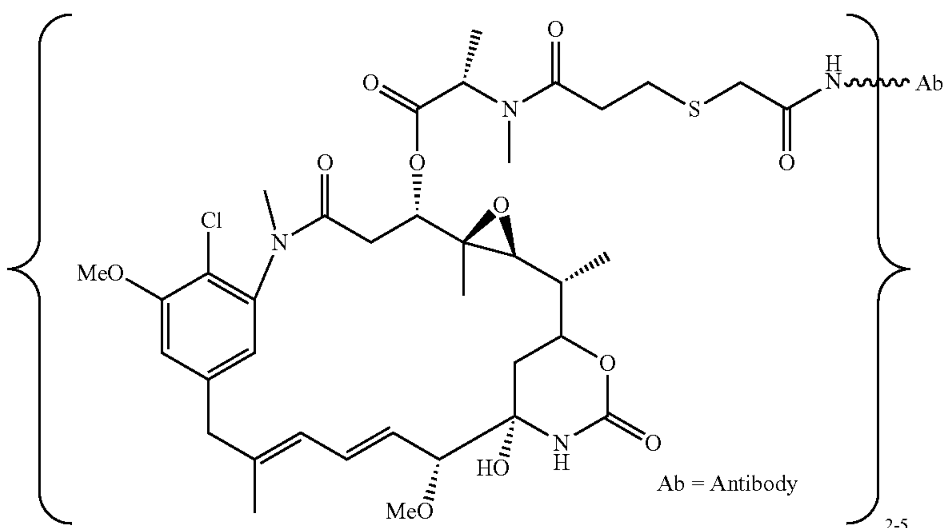
Ab-SIA-DM1
