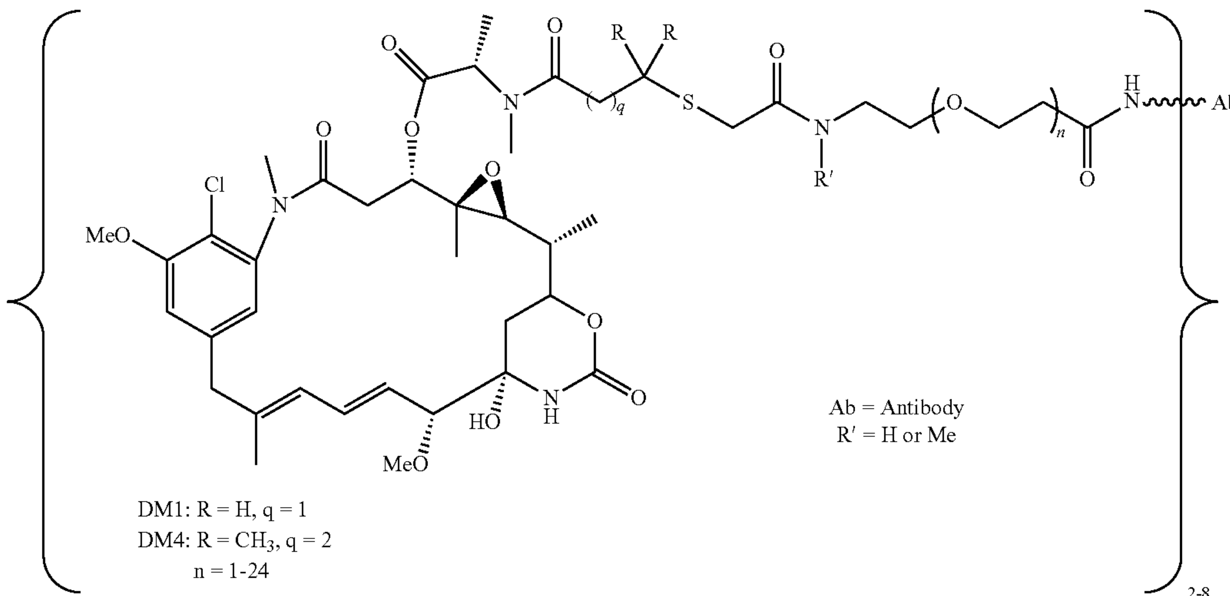
Ab-PEG-SIA-DM1/DM4
