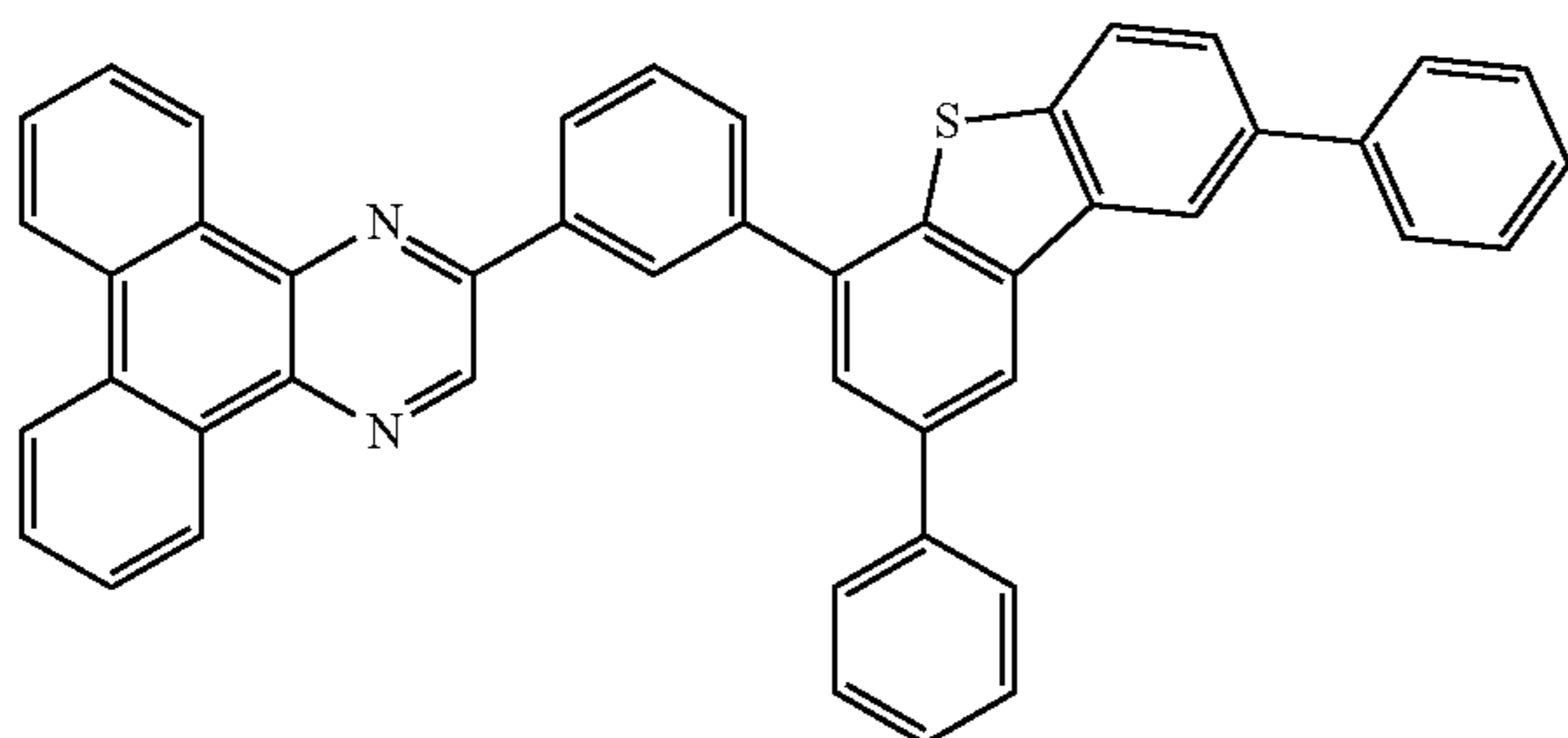
2mDBTPDBq-III
