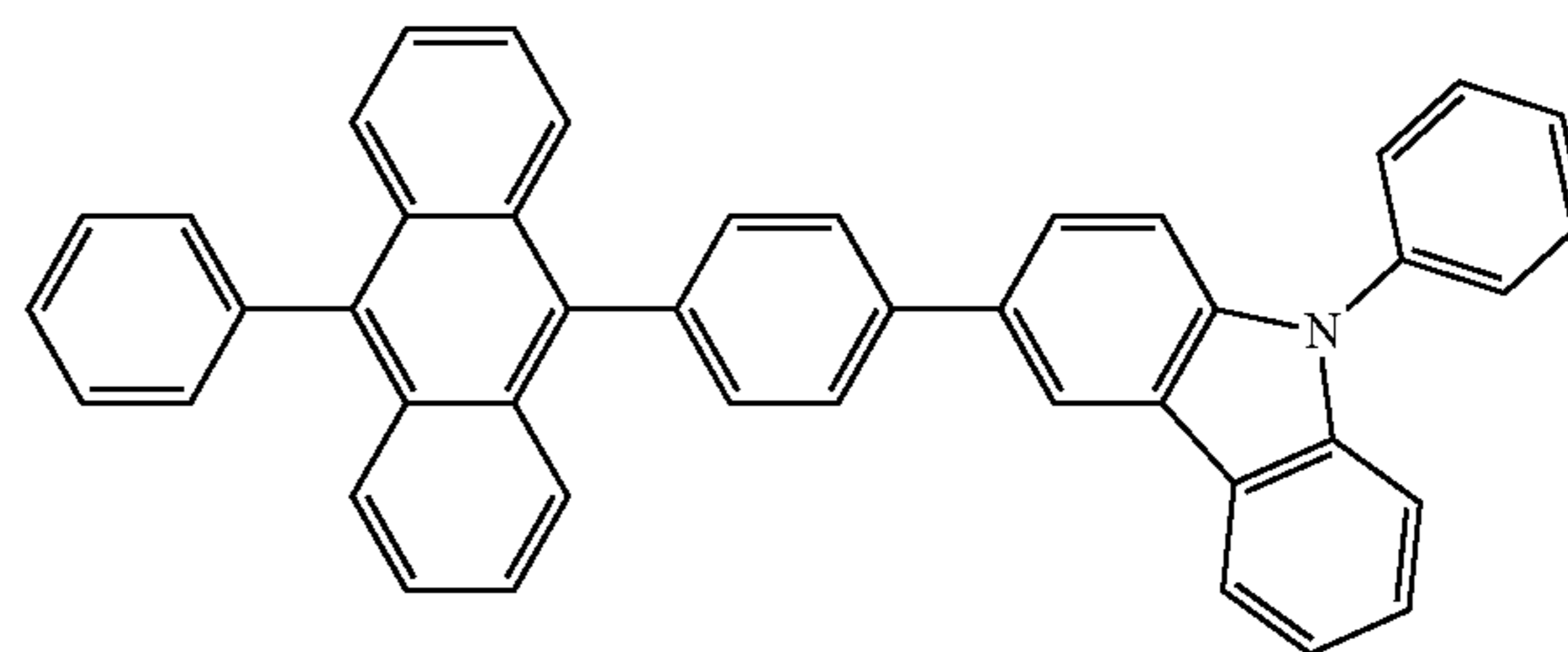
PCzPA
