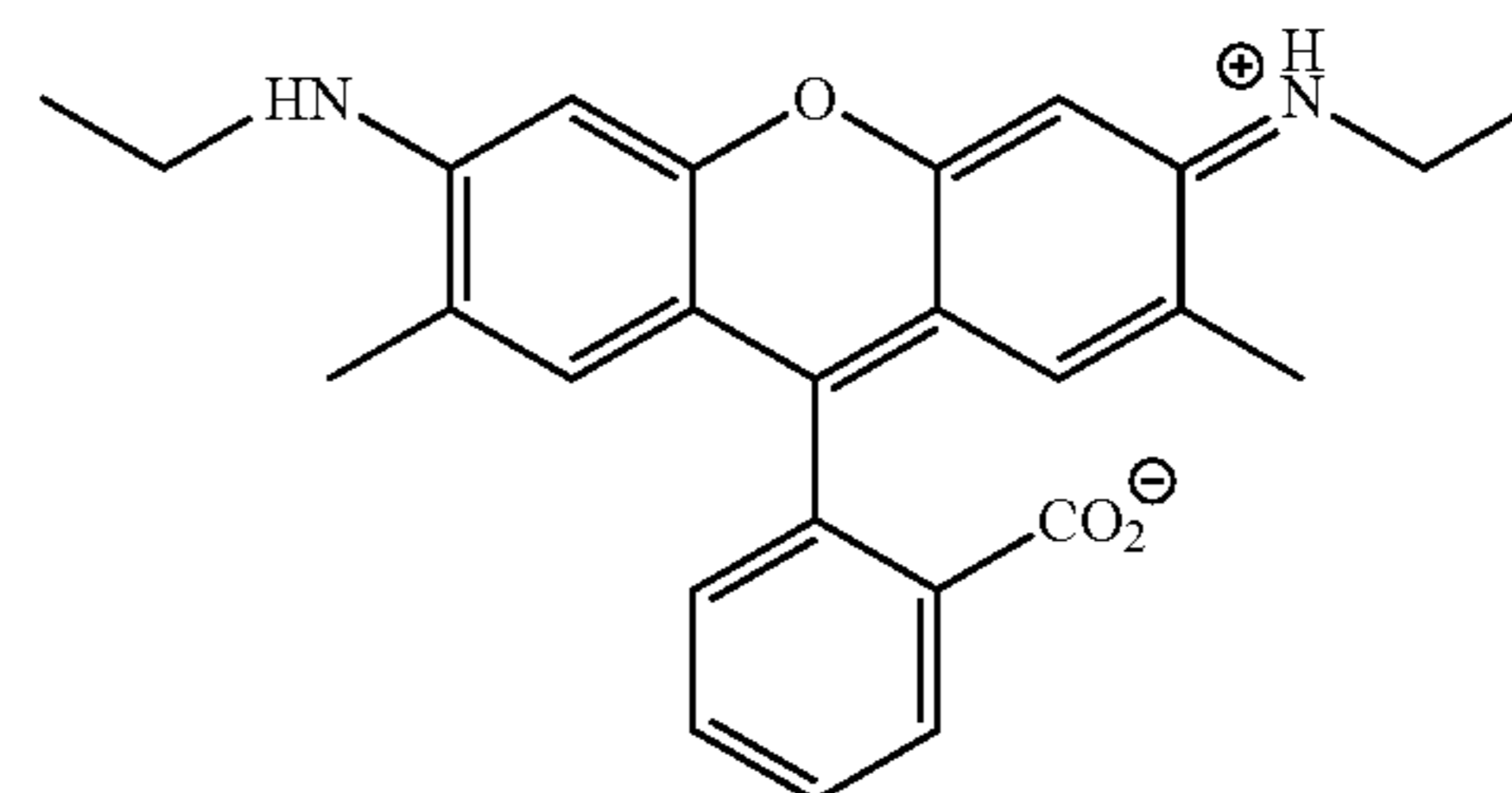
Rhodamine 575
