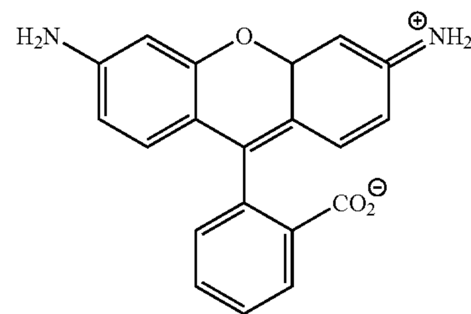
Rhodamine 110
