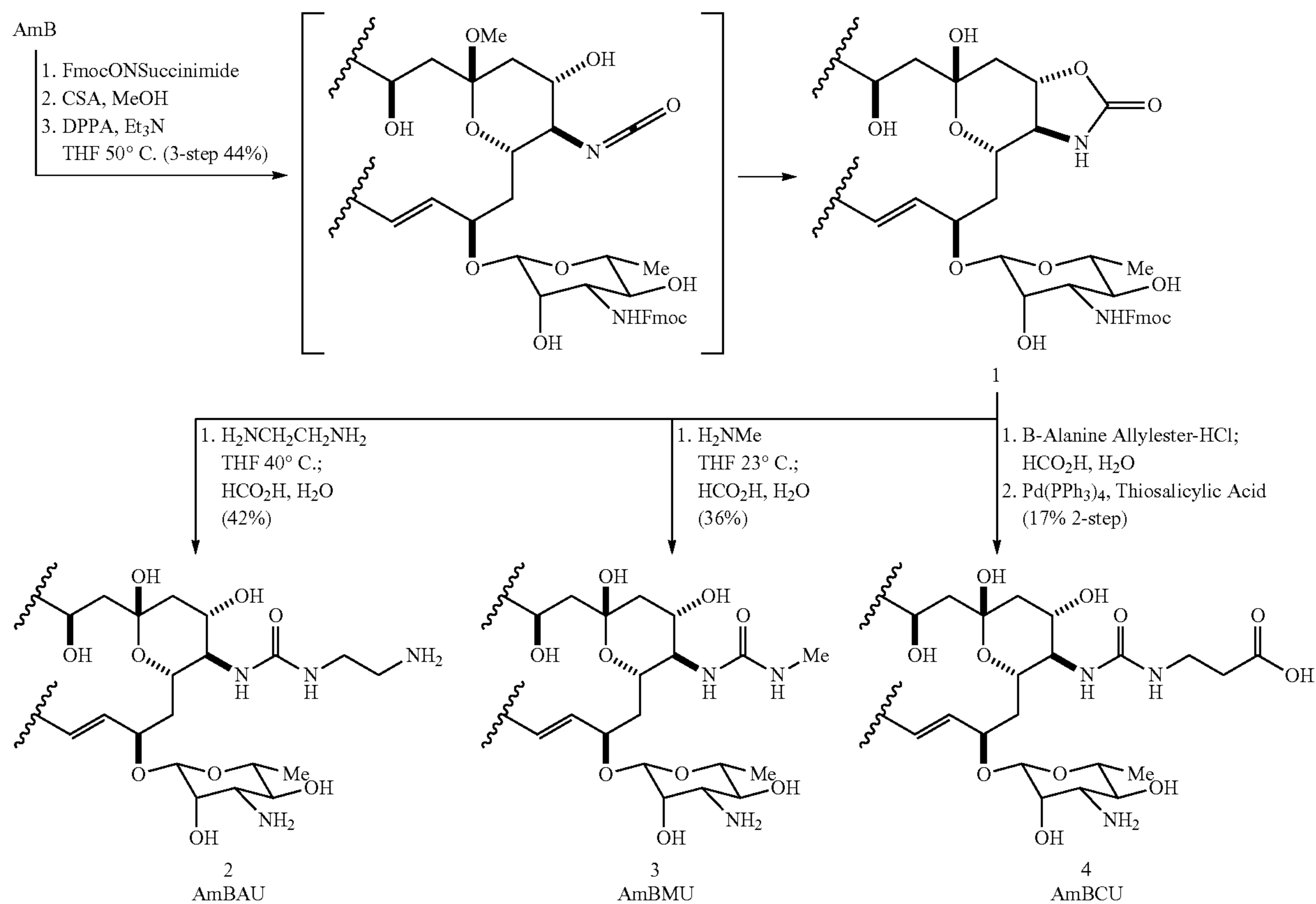
Scheme 1: Synthesis of C16 AmB derivatives
