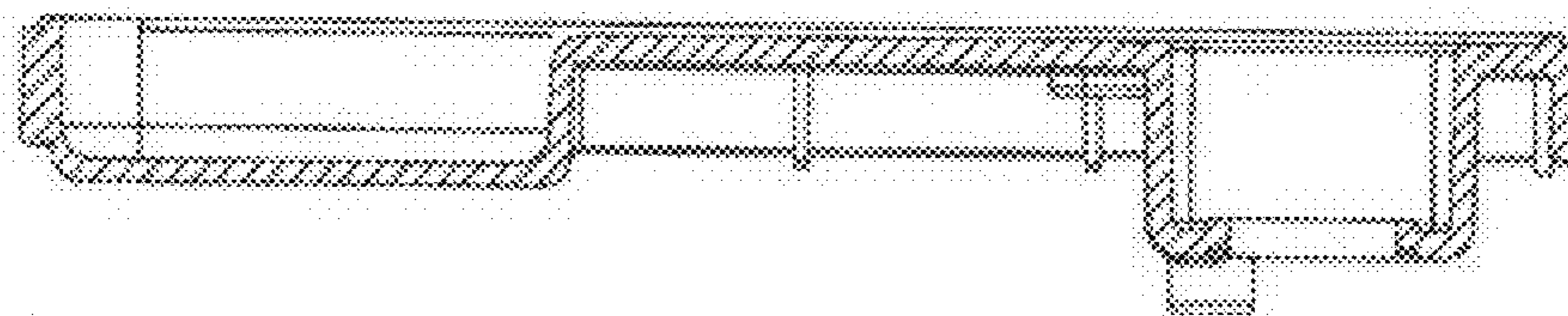
SECTION D-D
