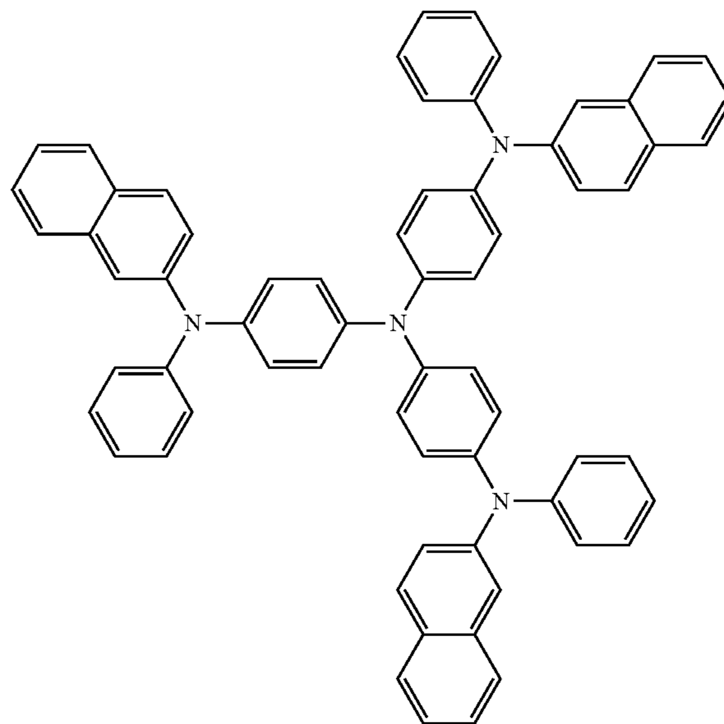
2-TDATA
