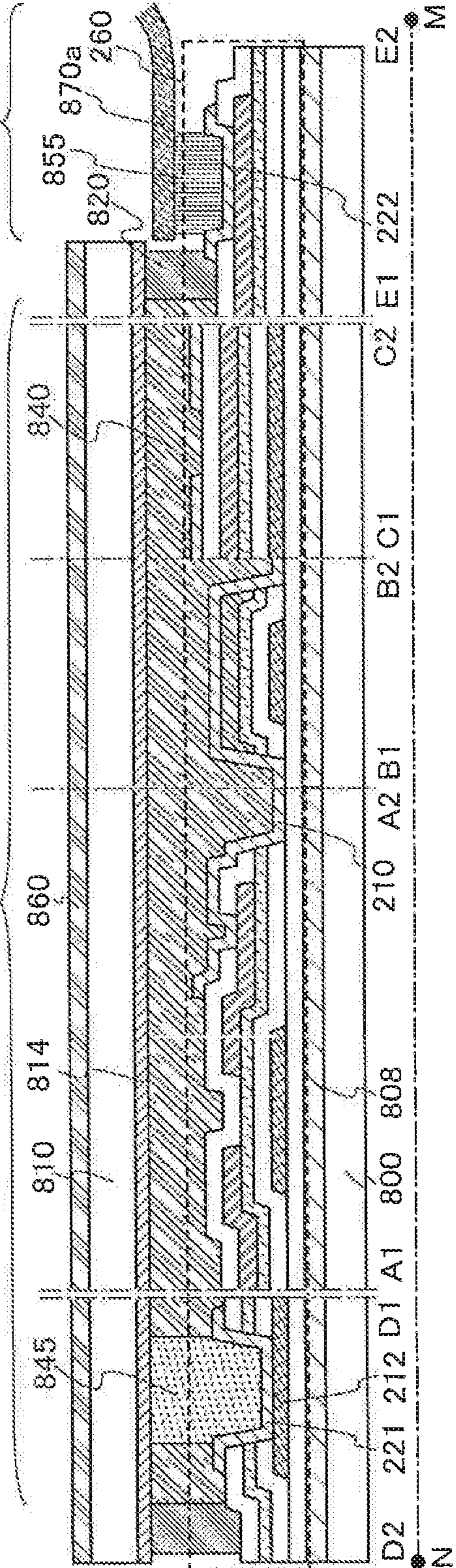
FIG. 11B
