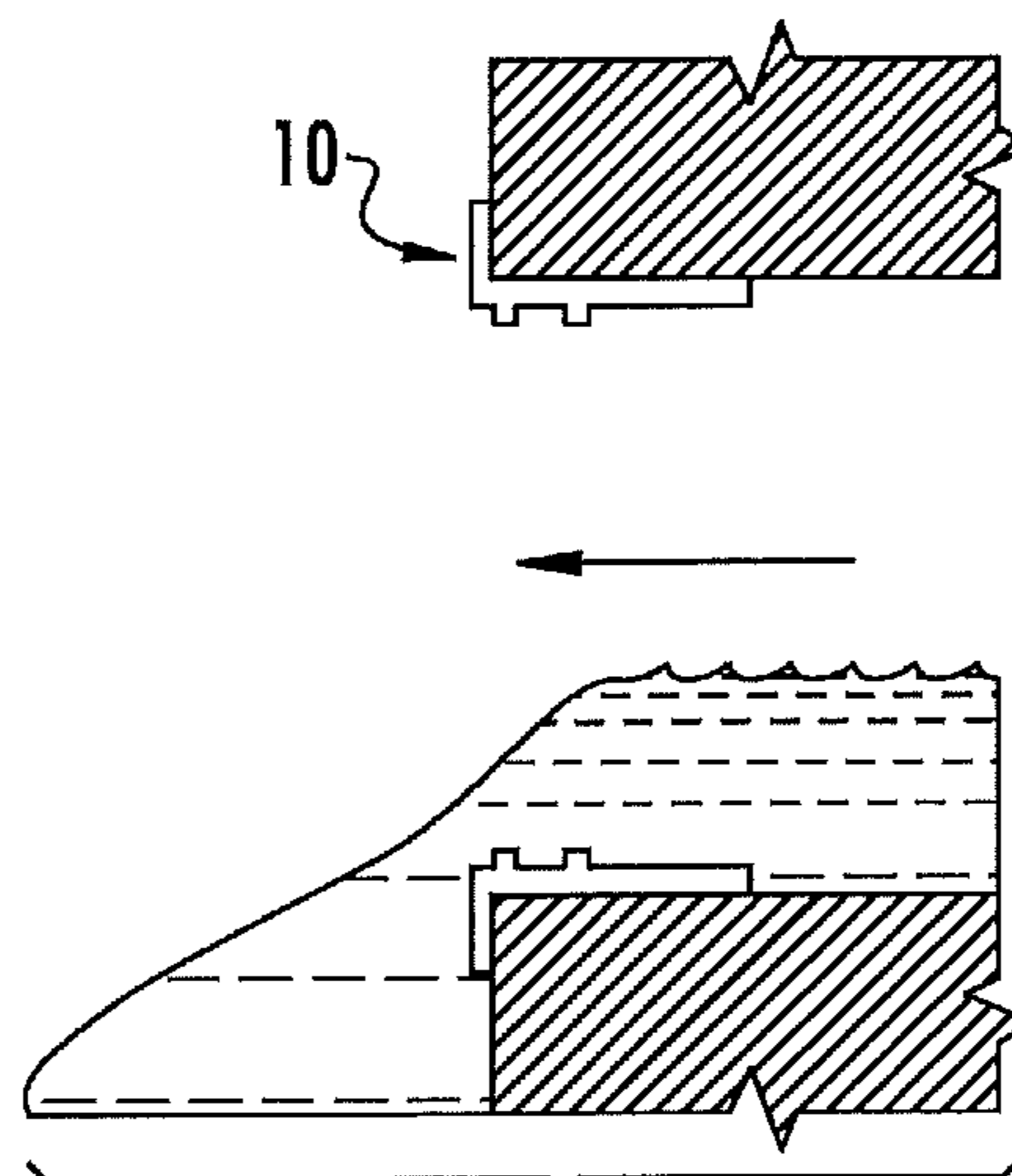
FIG. 3C
