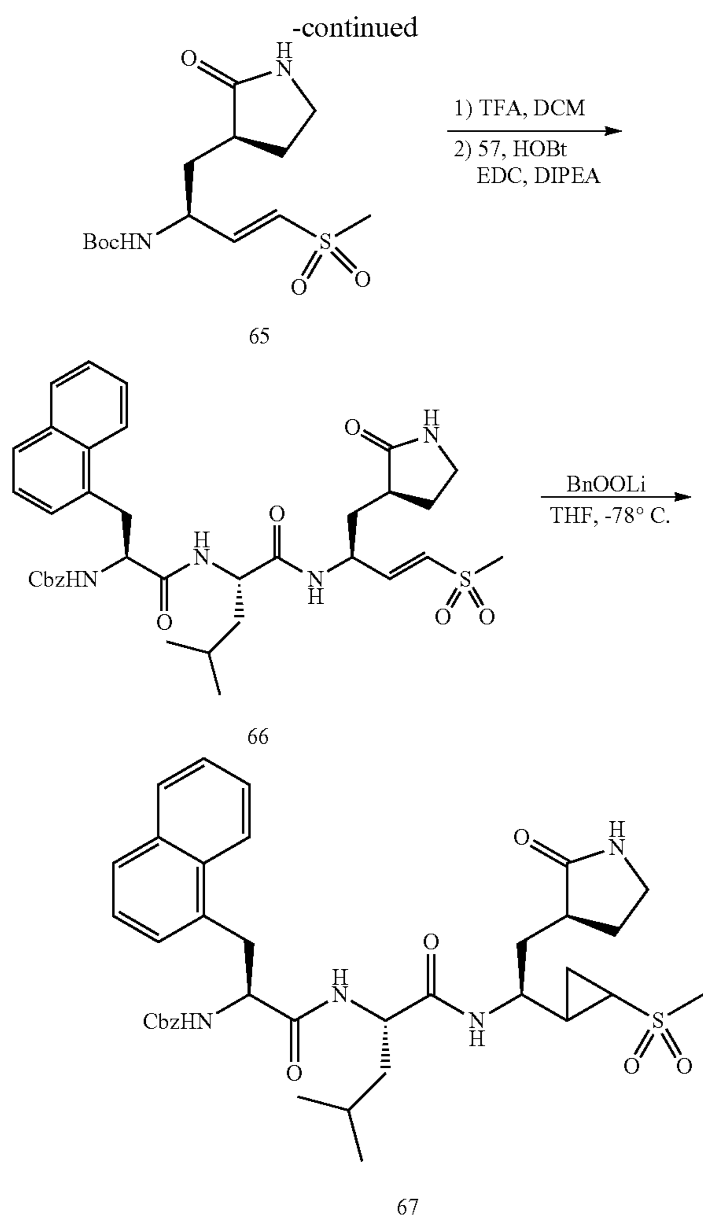
tert-Butyl ((S,E)-4-(methylsulfonyl)-1-((S)-2-oxopyrrolidin-3-yl)but-3-en-2-yl)carbamate (65)
