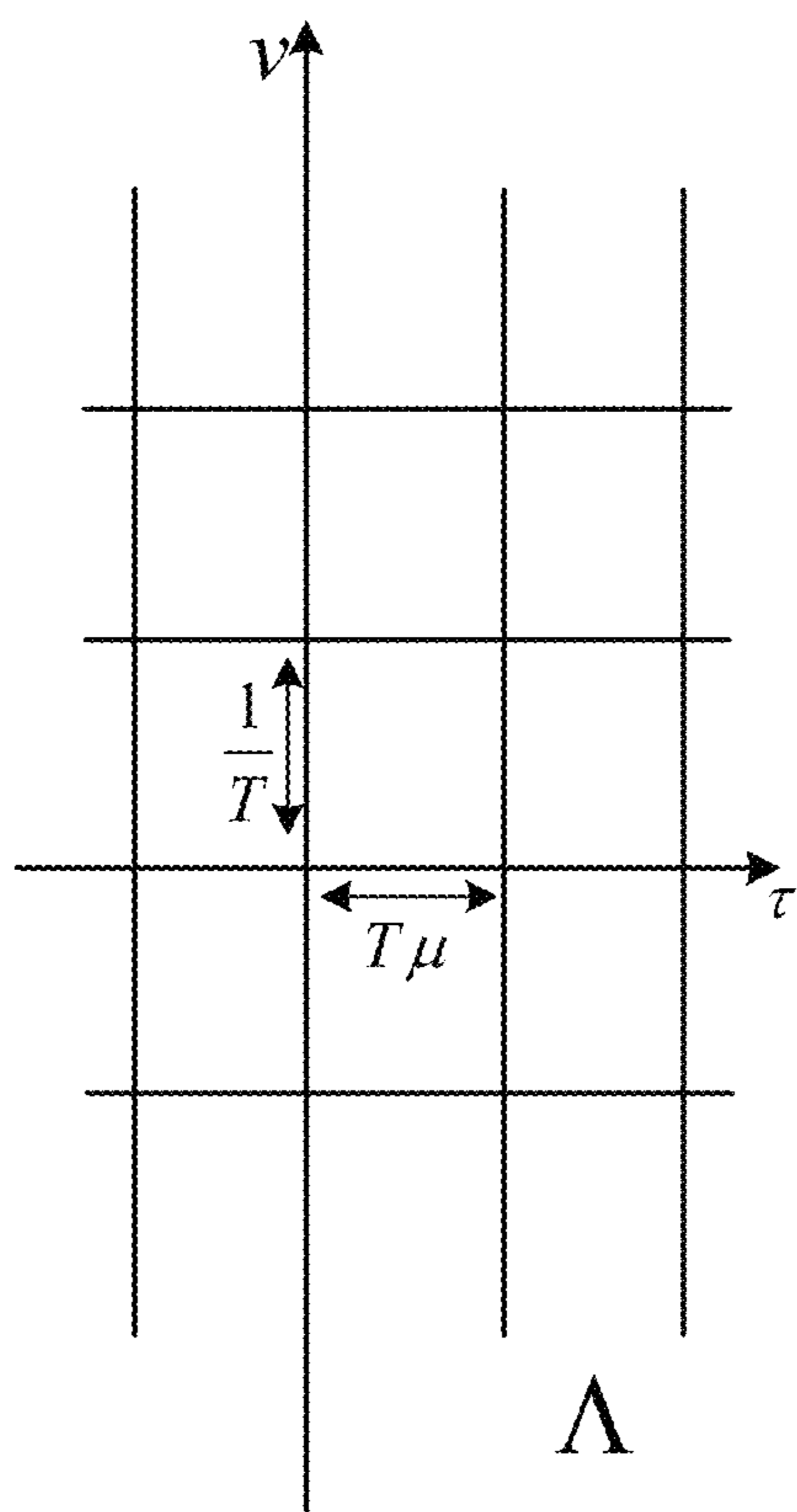
Primal lattice
