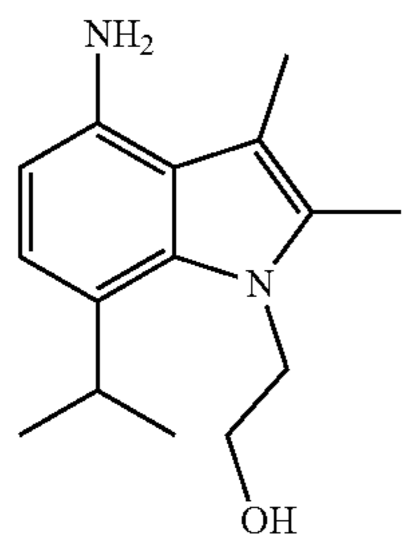
2-[4-amino-2,3-dimethyl-7-(propan-2-yl)-1H-indol-1-yl]ethanol
