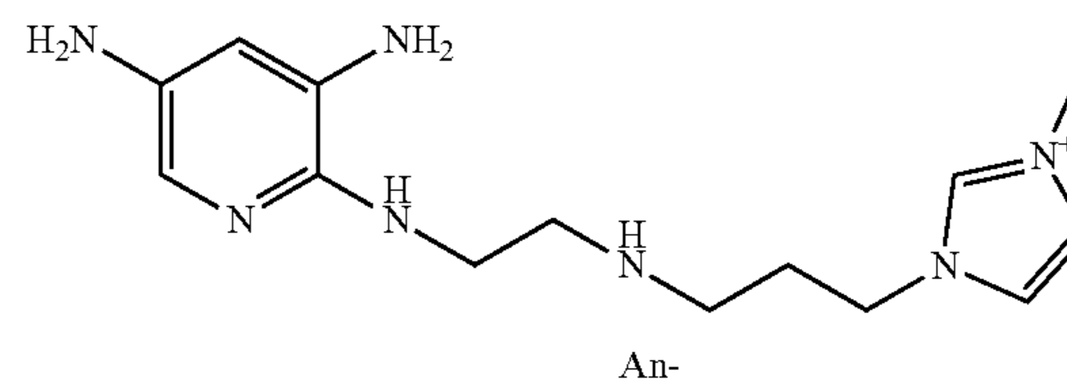
1-[3-((2-[(3,5-diaminopyridin-2-yl)amino]ethyl)amino)propyl]-3-methyl-1H-imidazol-3-ium, An -
