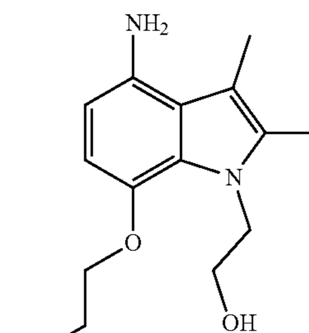
2-[4-amino-7-(2-hydroxyethoxy)-2,3-dimethyl-1H-indol-1-yl]ethanol
