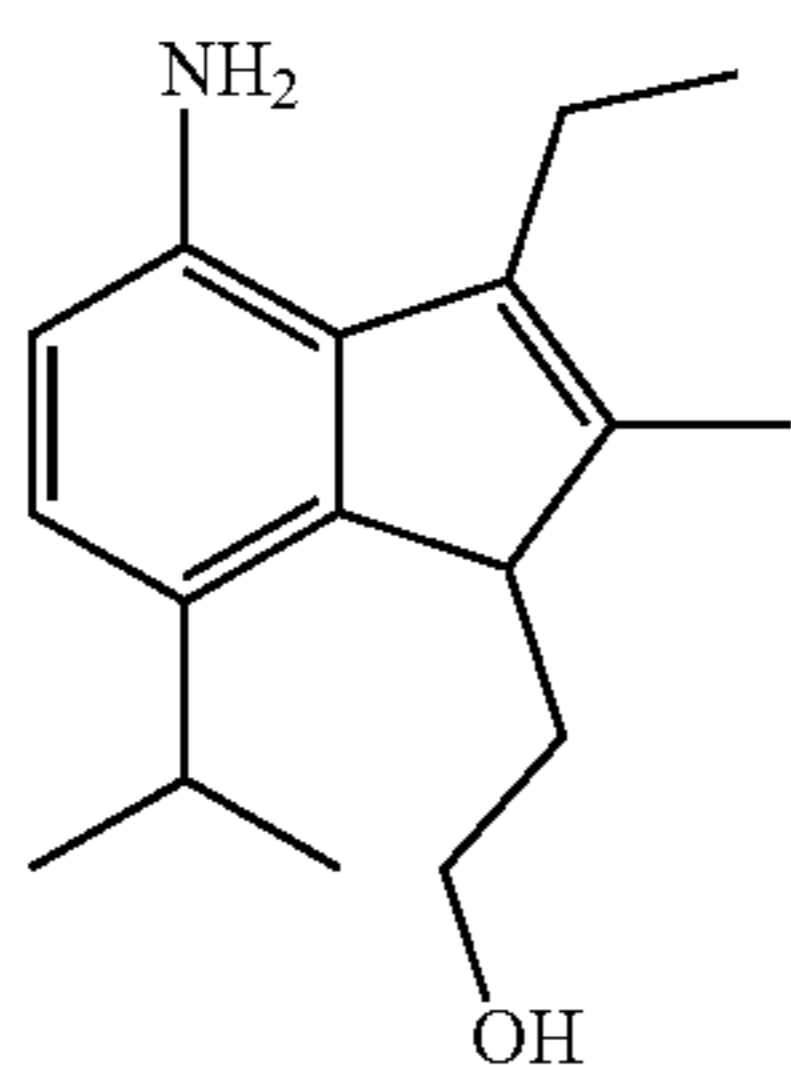
2-[4-amino-3-ethyl-2-methyl-7-(propan-2-yl)-1H-indol-1-yl]ethanol
