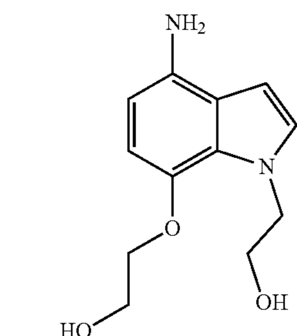
2-[4-amino-7-(2-hydroxyethoxy)-1H-indol-1-yl]ethanol
