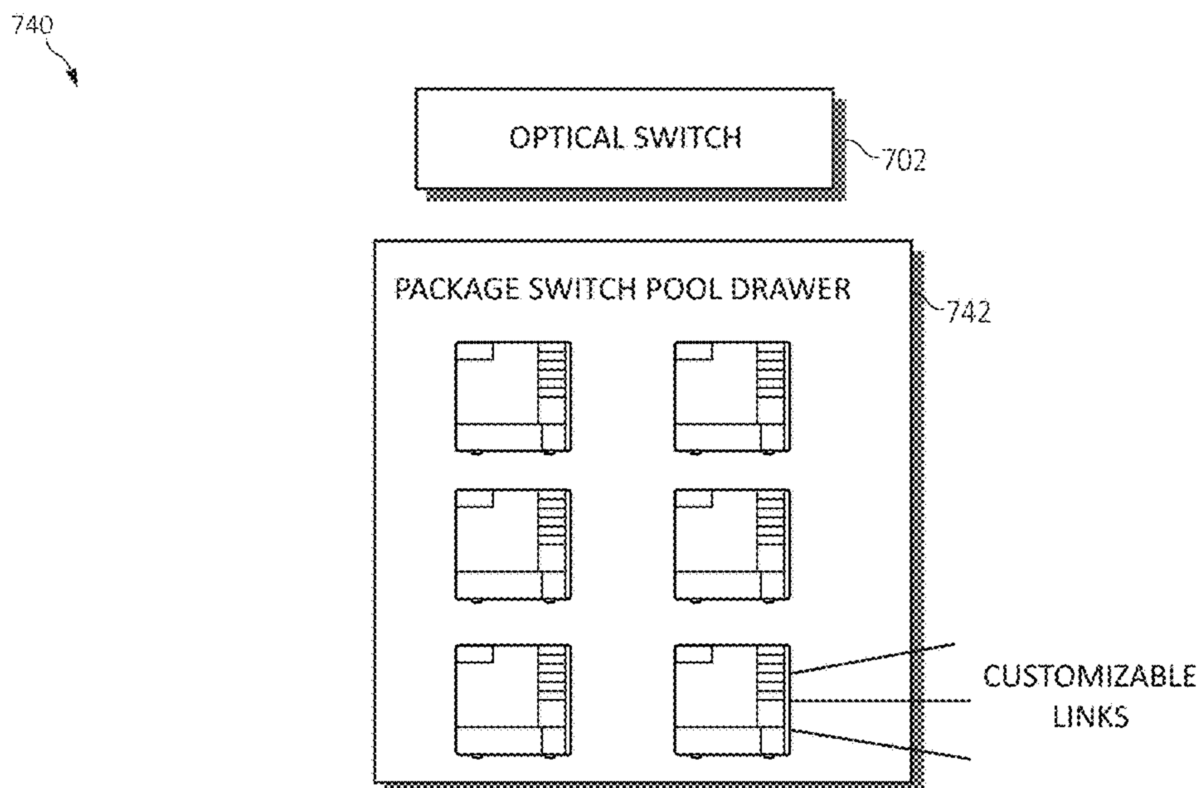
FIG. 7C
