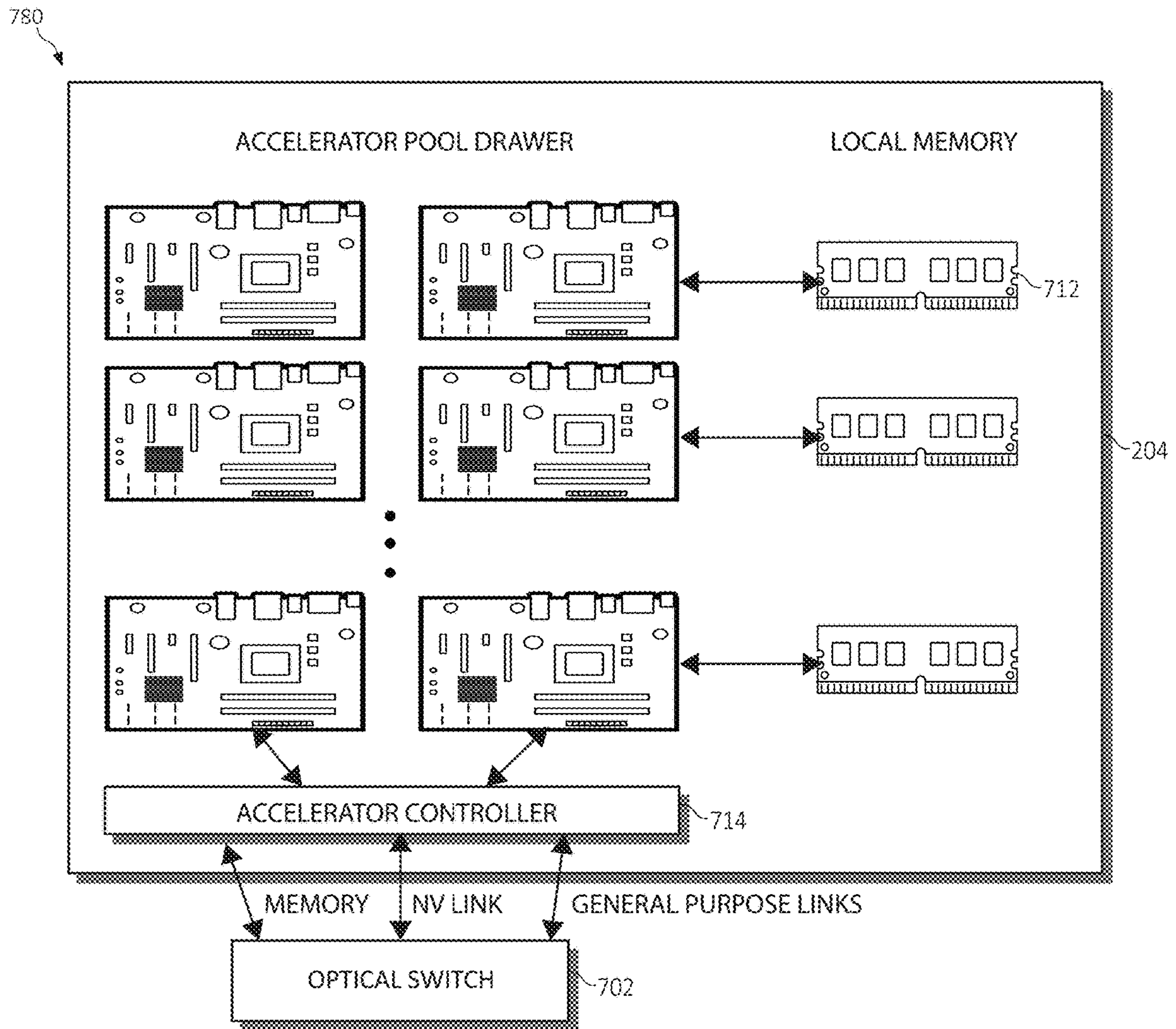
FIG. 7E
