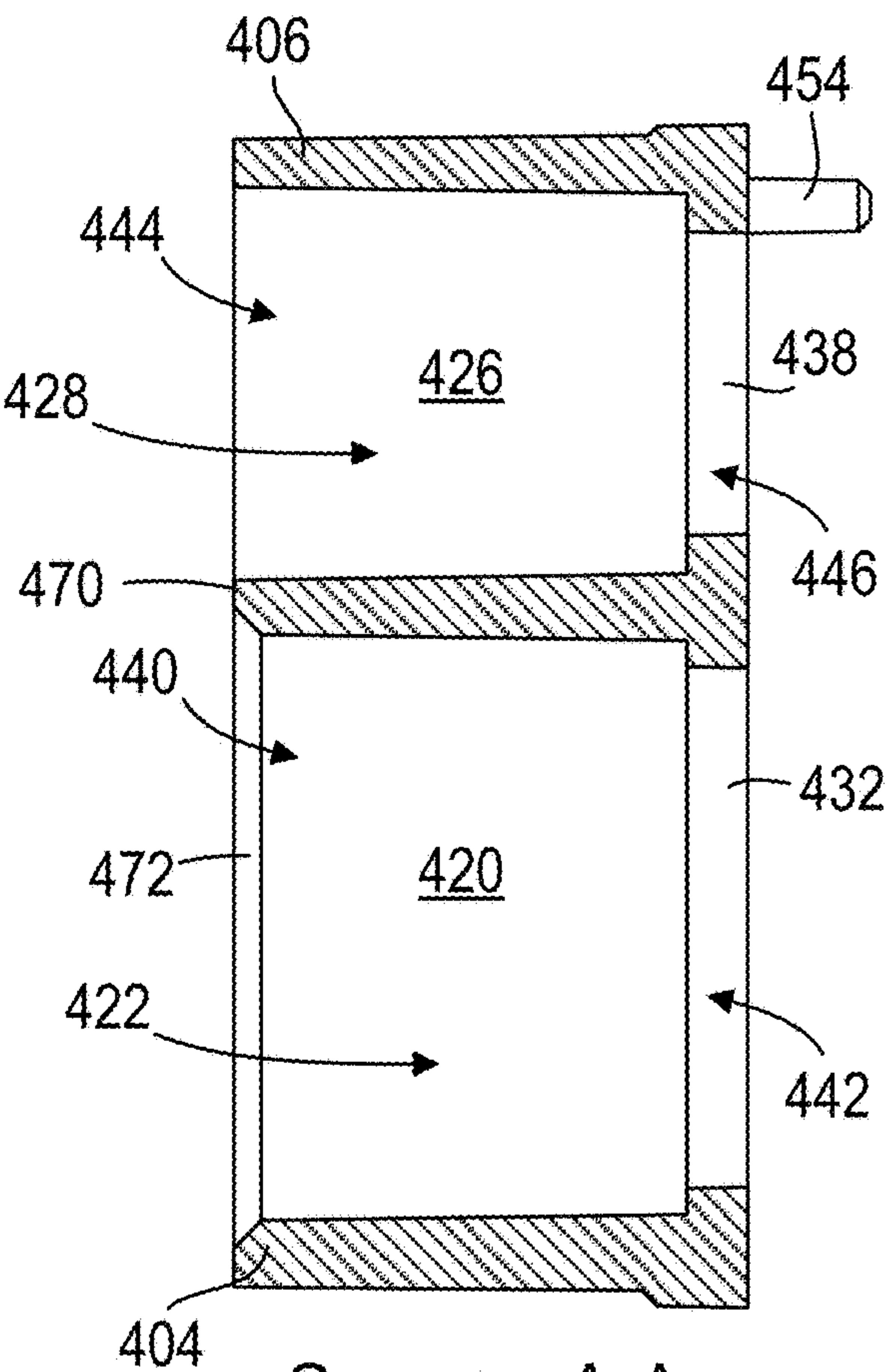
SECTION A-A FIG. 34
