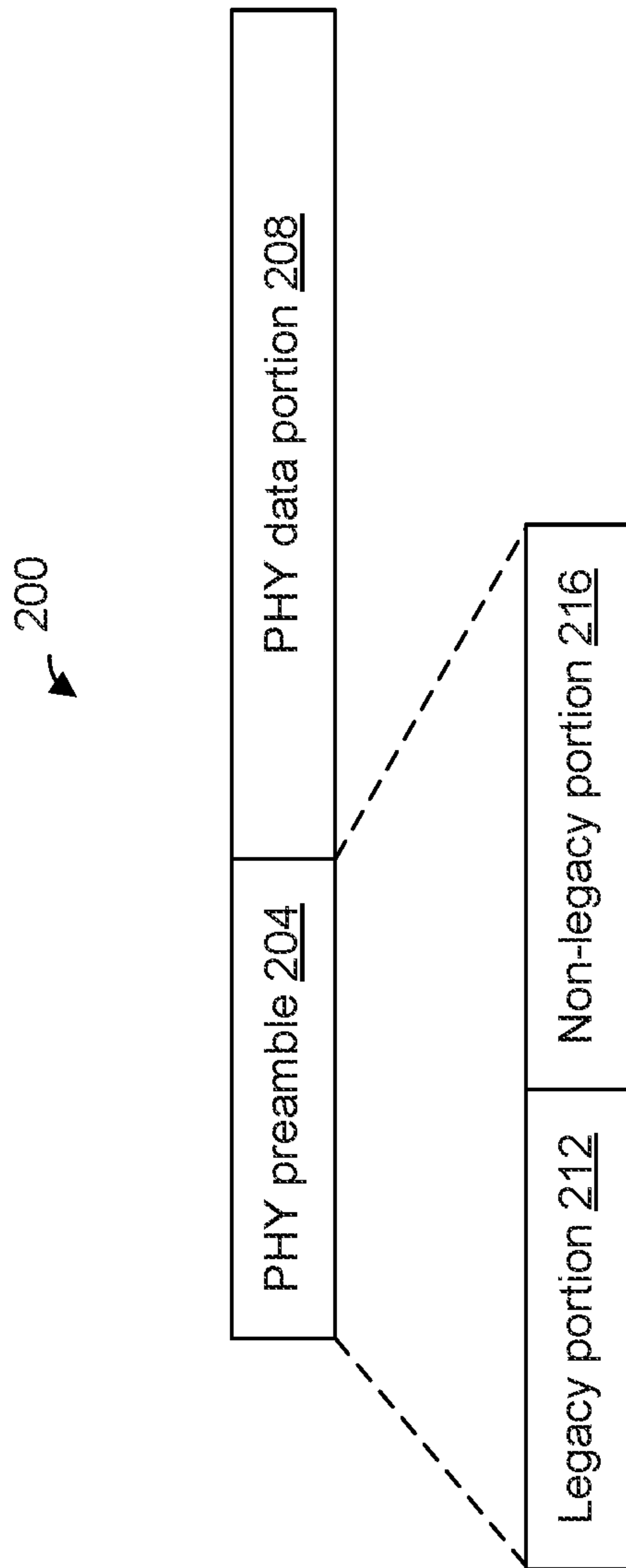
FIG. 2A
