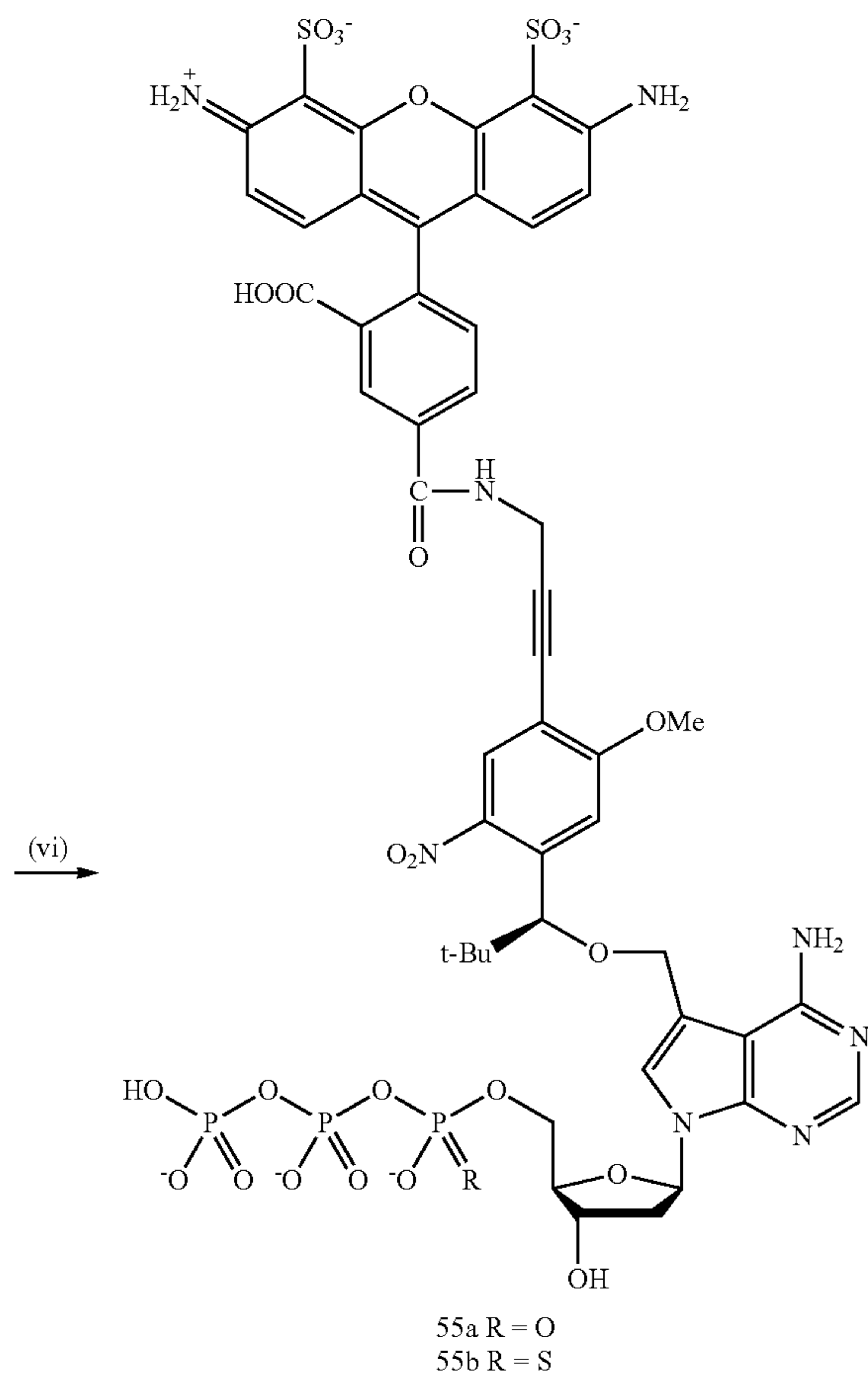
Scheme S25b.
