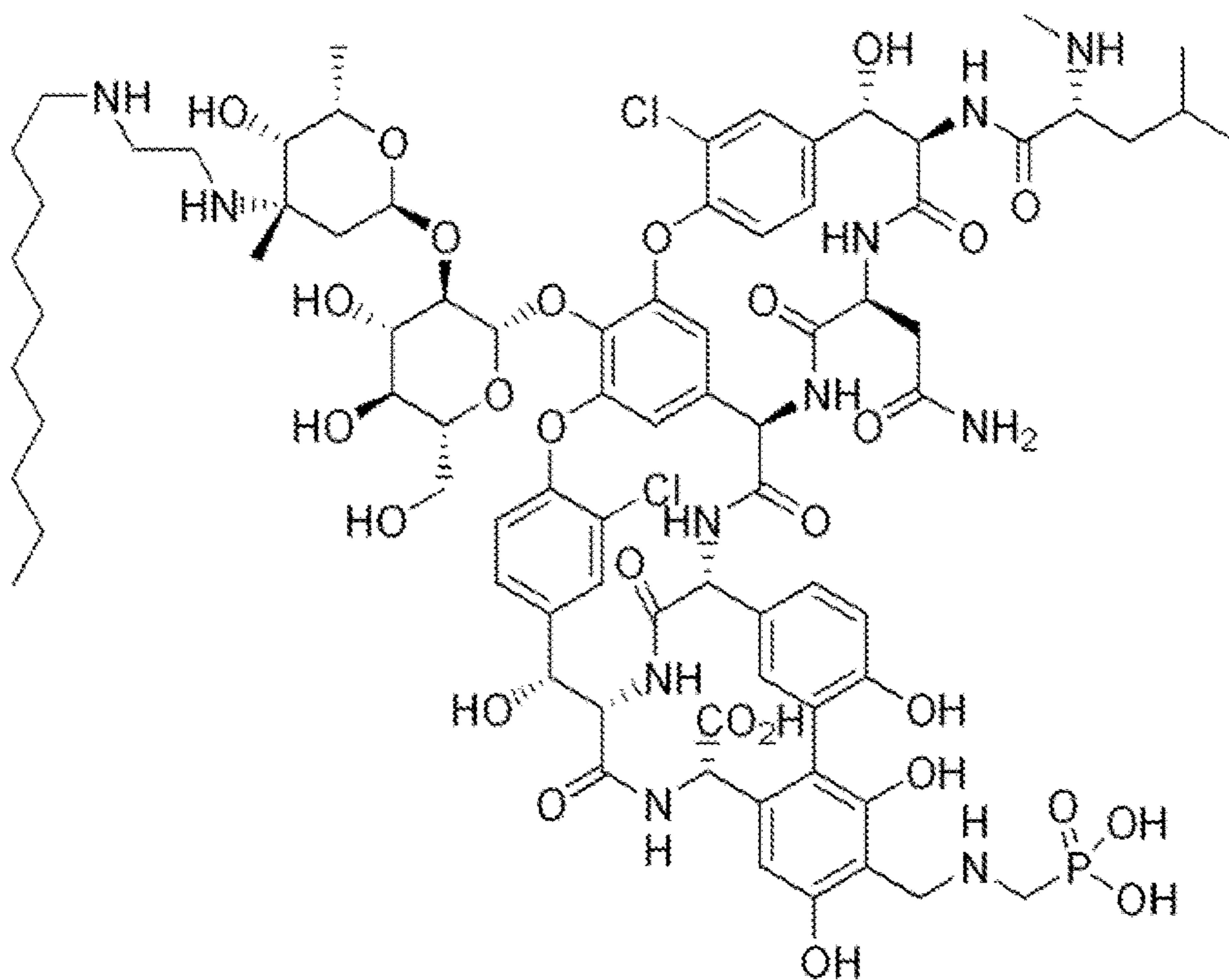
Telavancin
