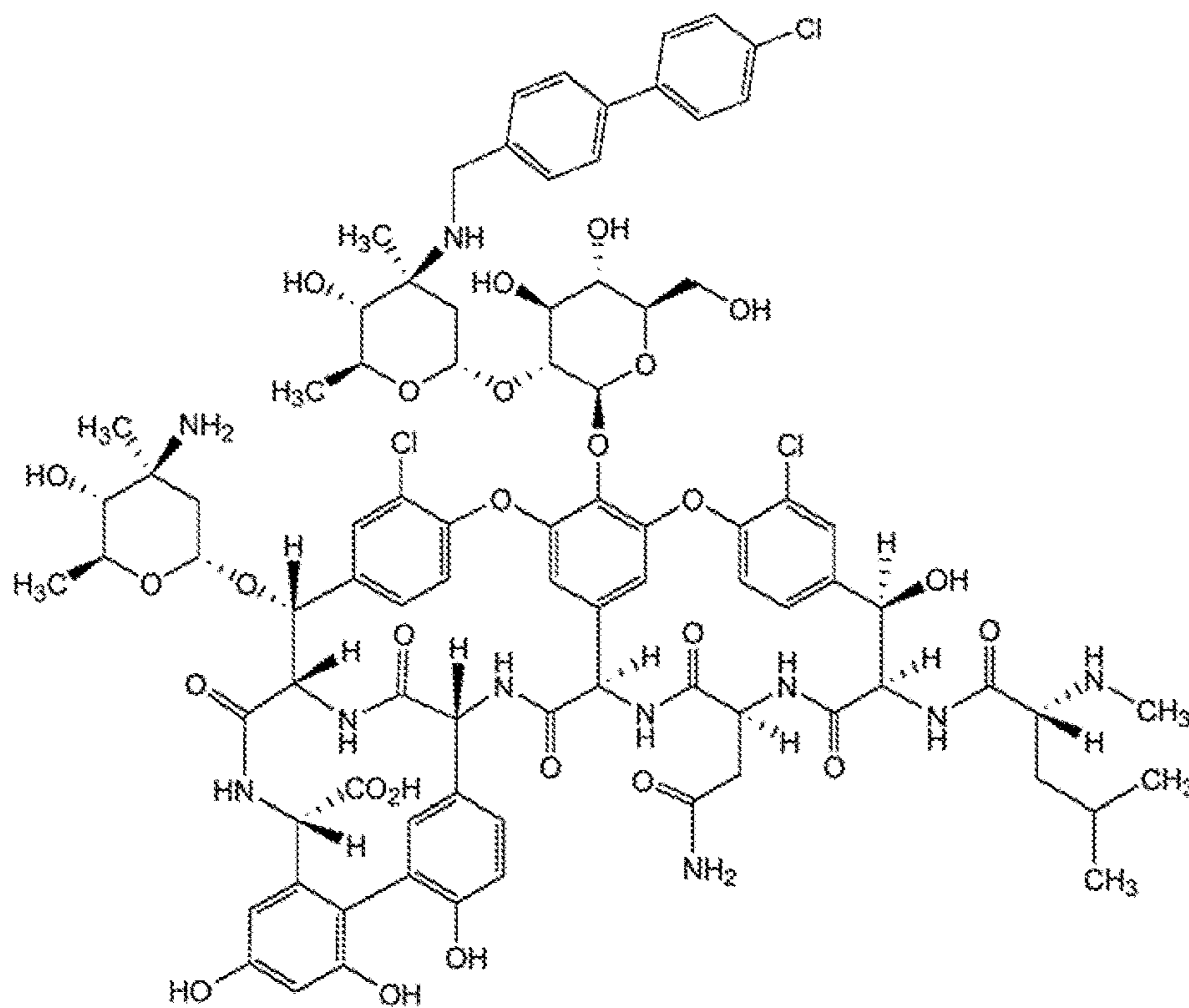
Oritavancin
