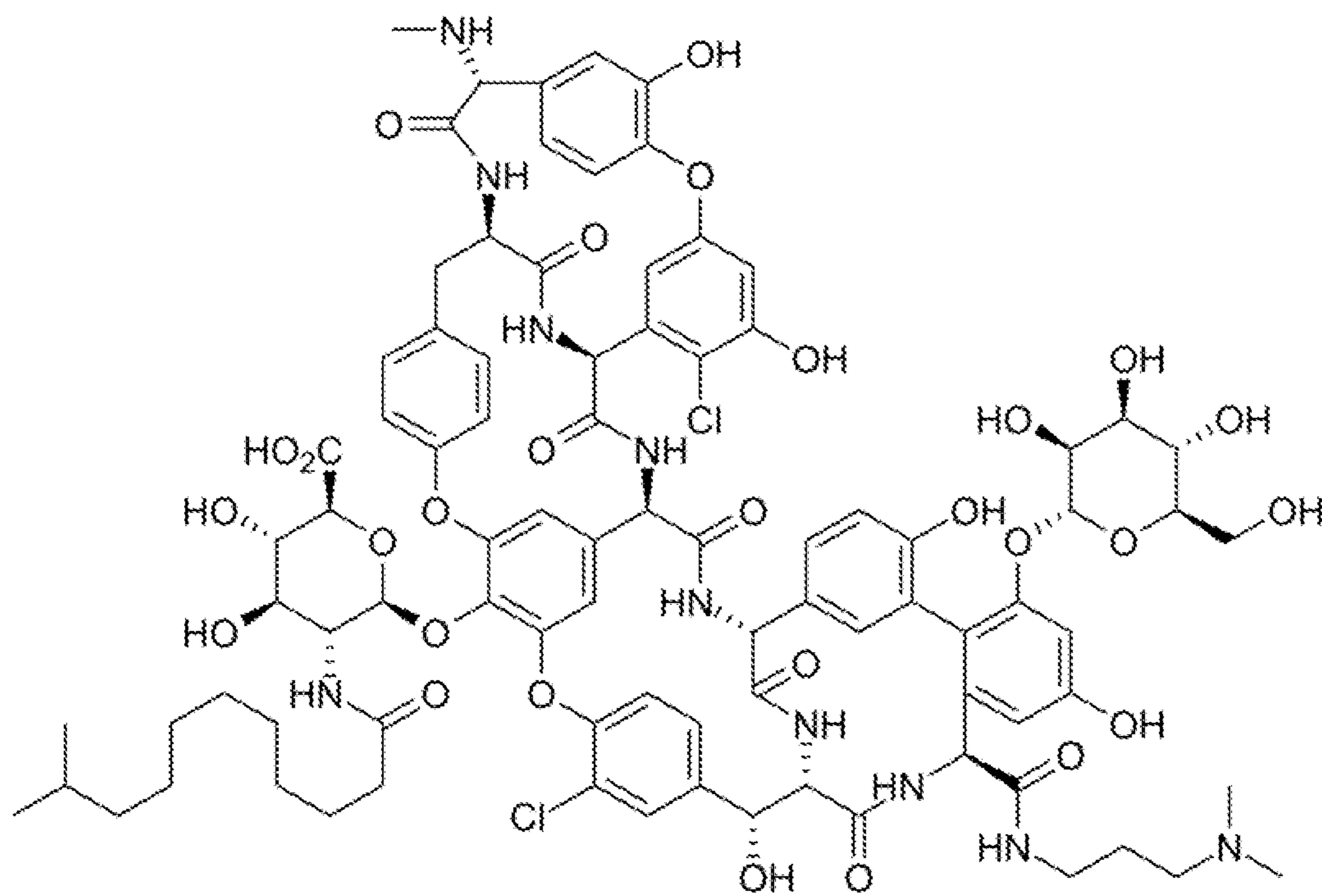
Dalbavancin
