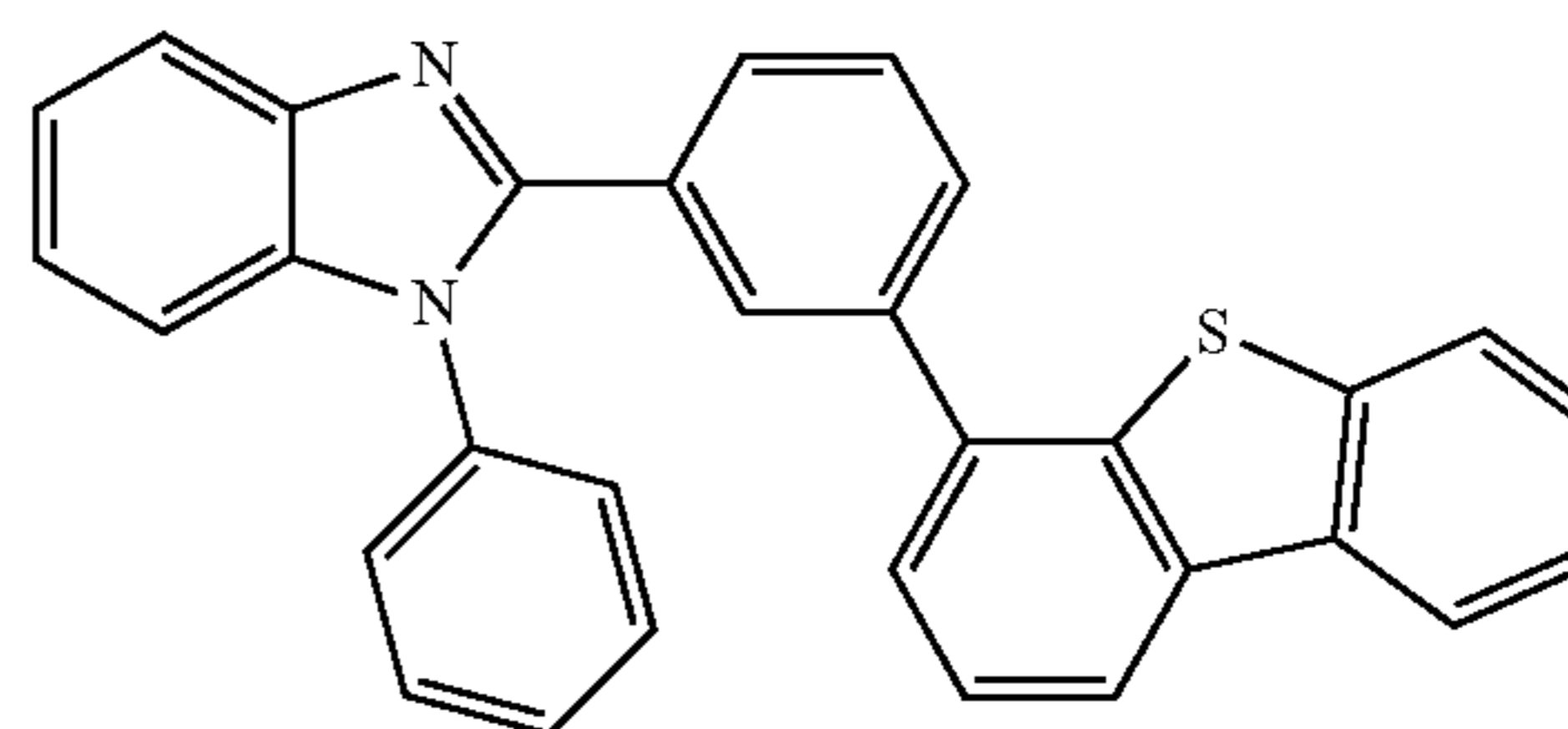
mDBTBlm-II
