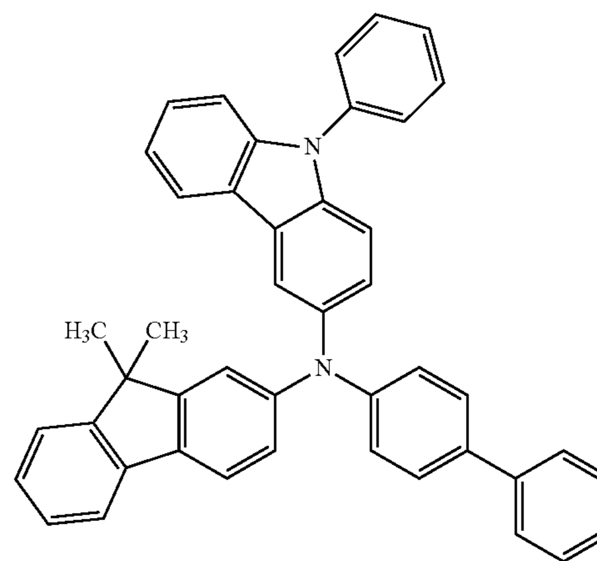
PCBiF
