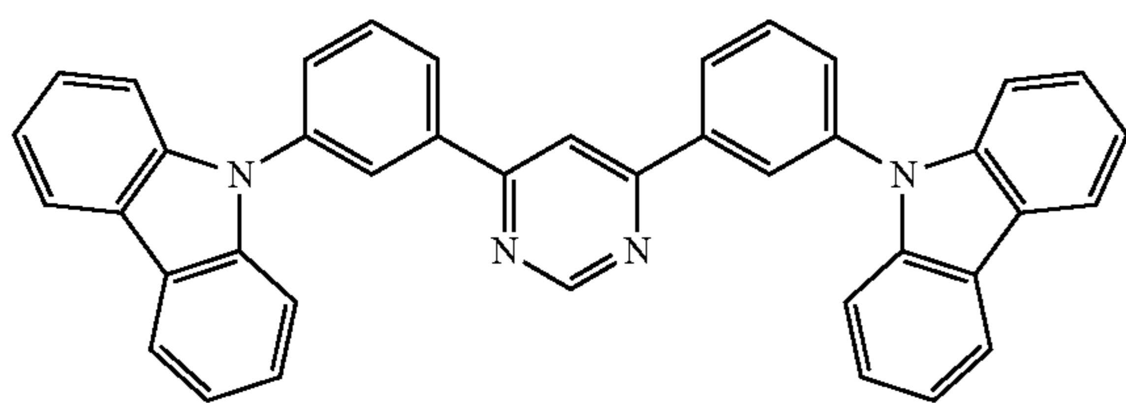
4,6mCzP2Pm
