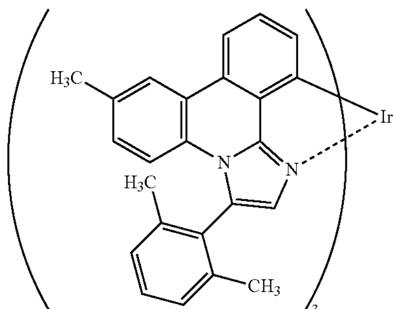
Ir(dmpimpt-Me) 3
