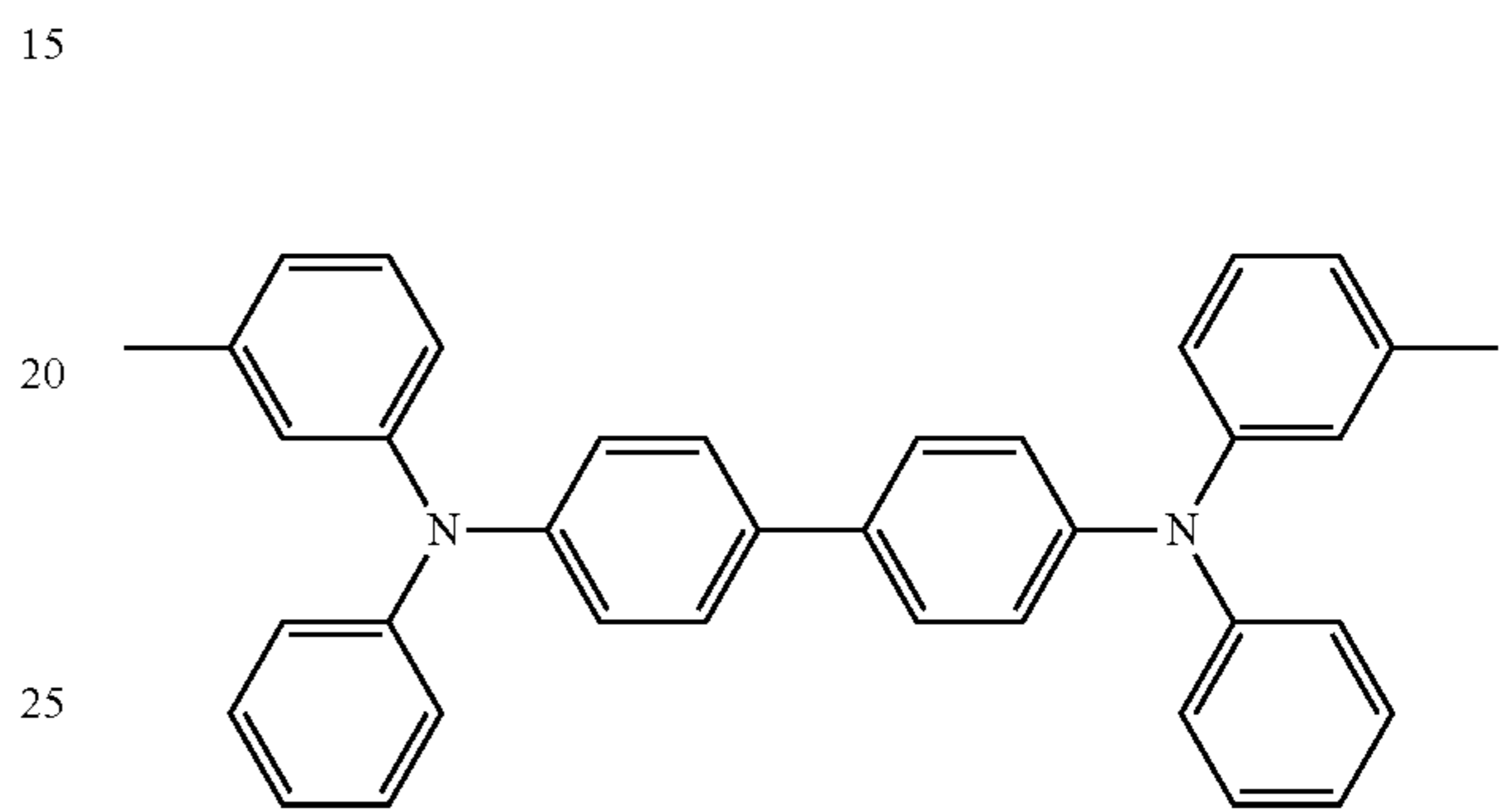
TPD
