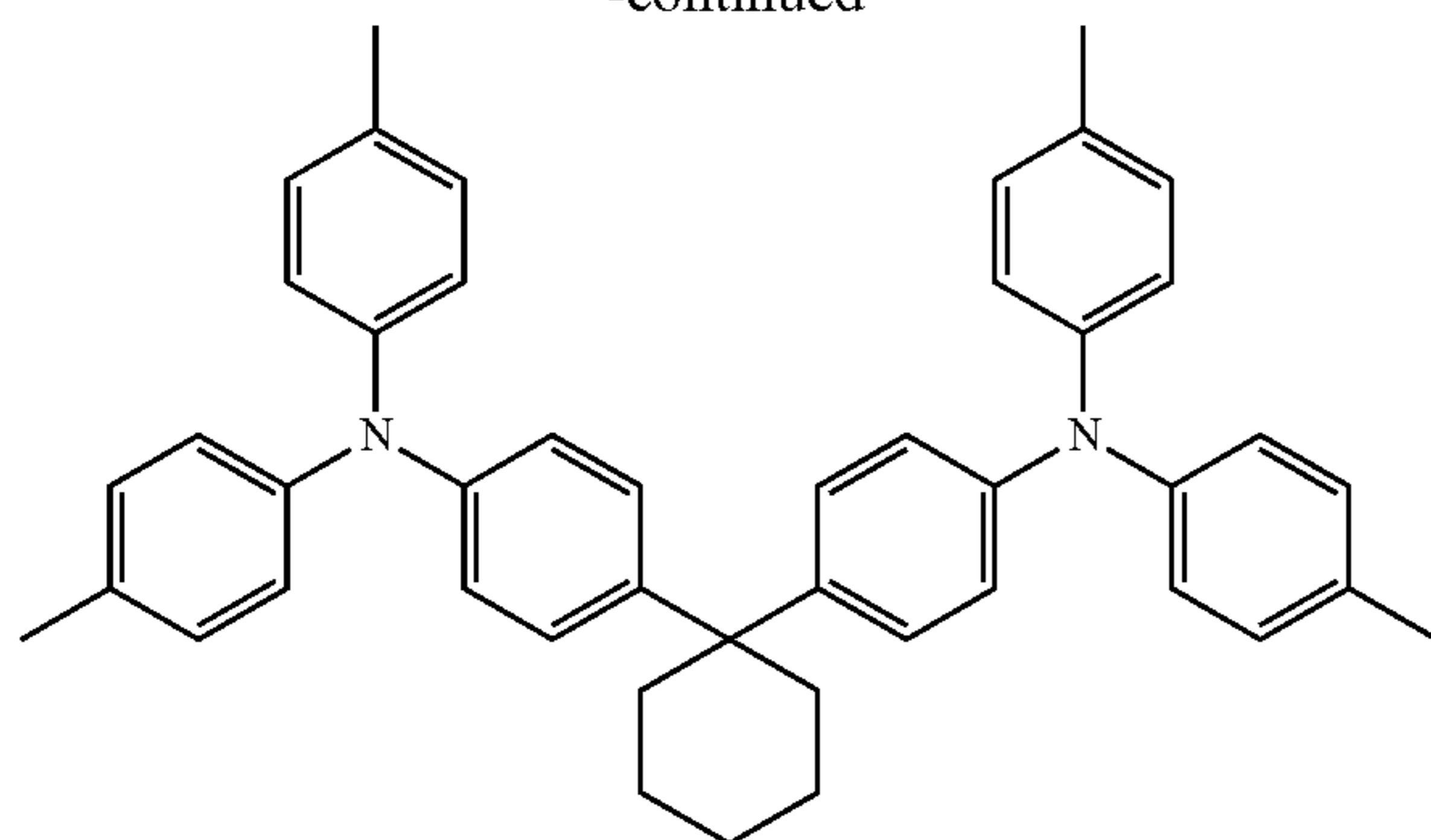
TAPC
