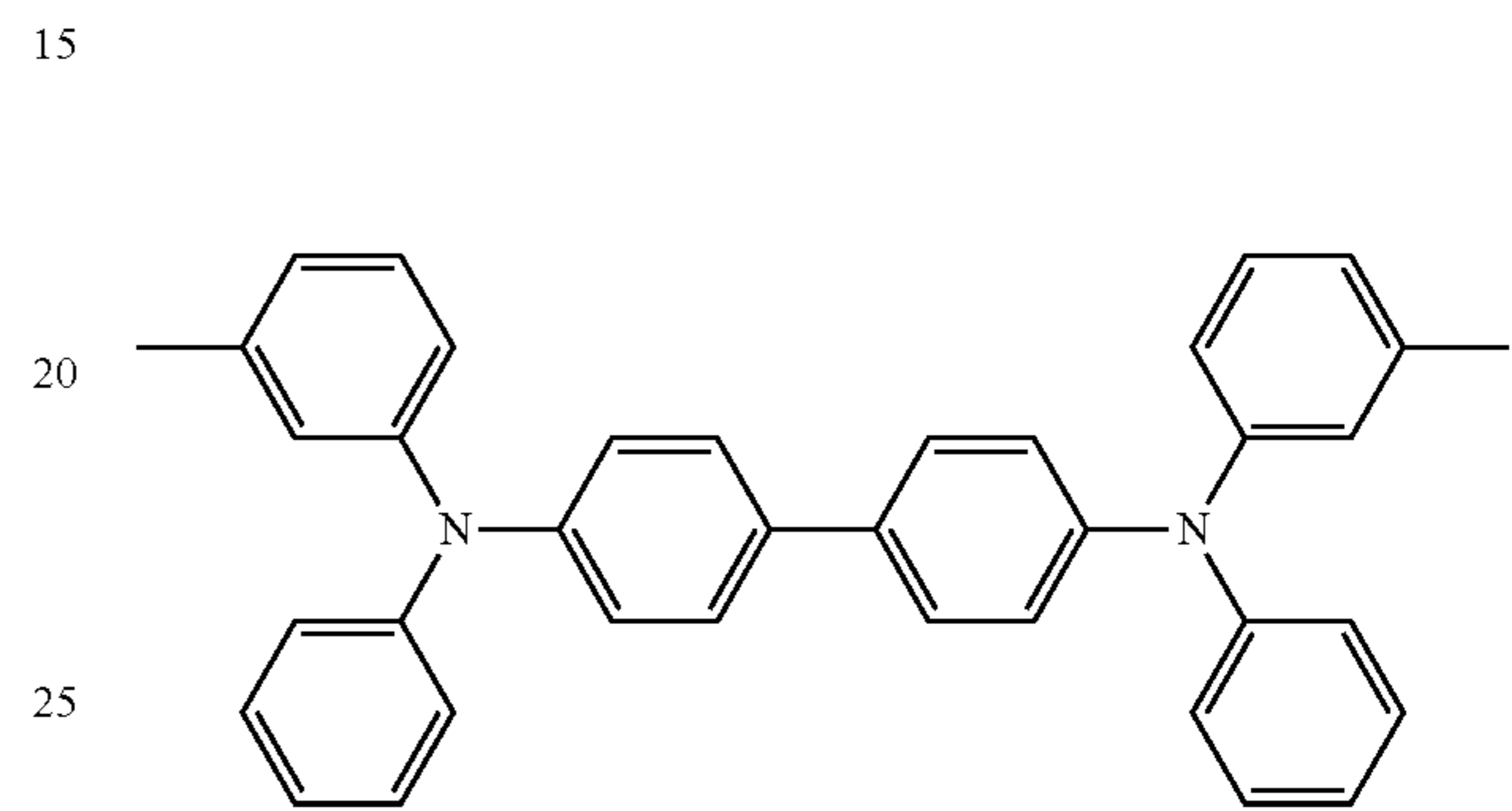
TPD
