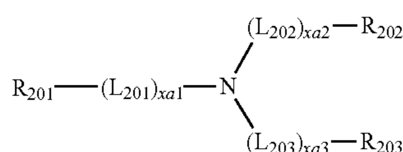
HMTPD
