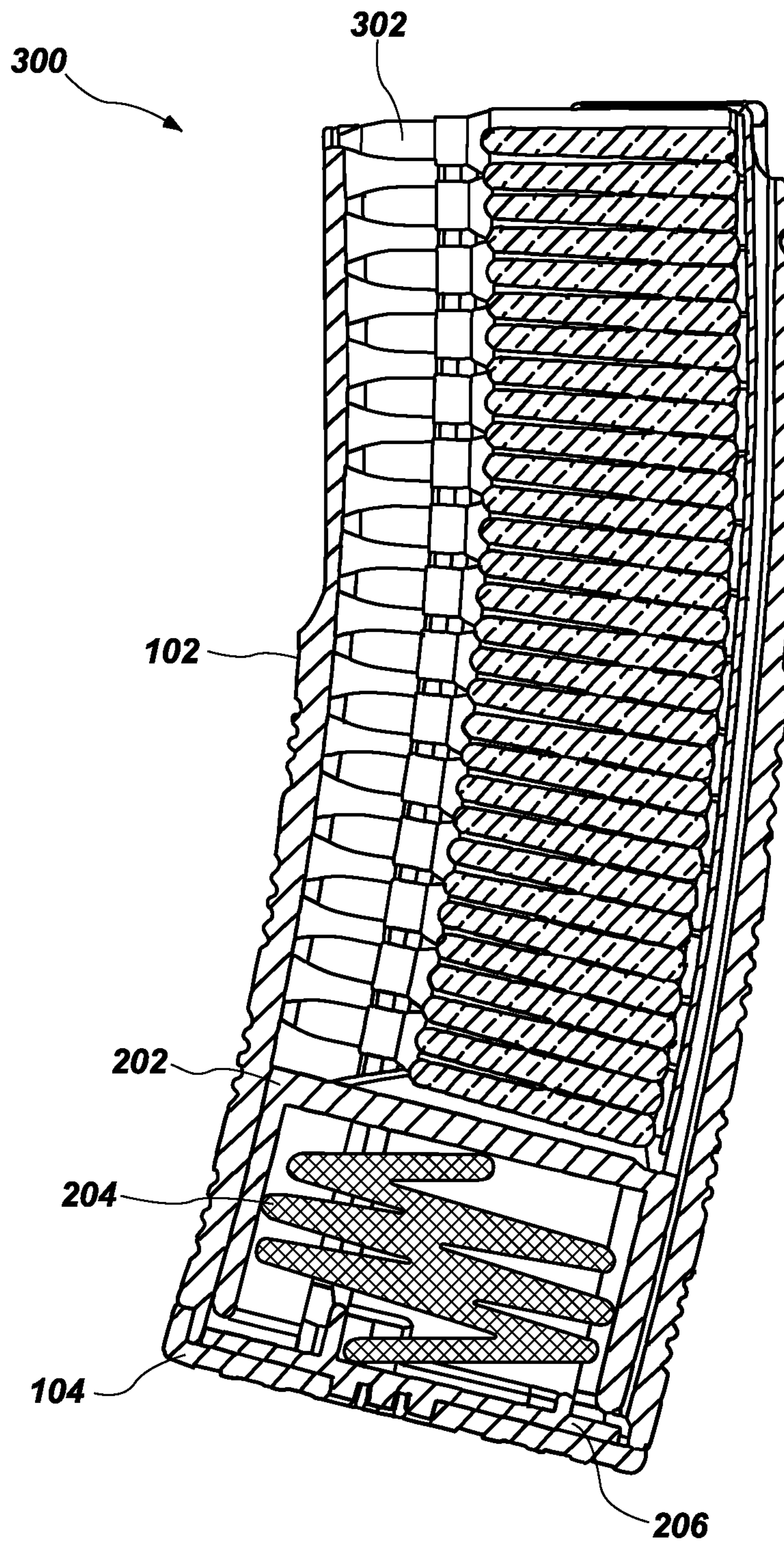
SECTION A-A
