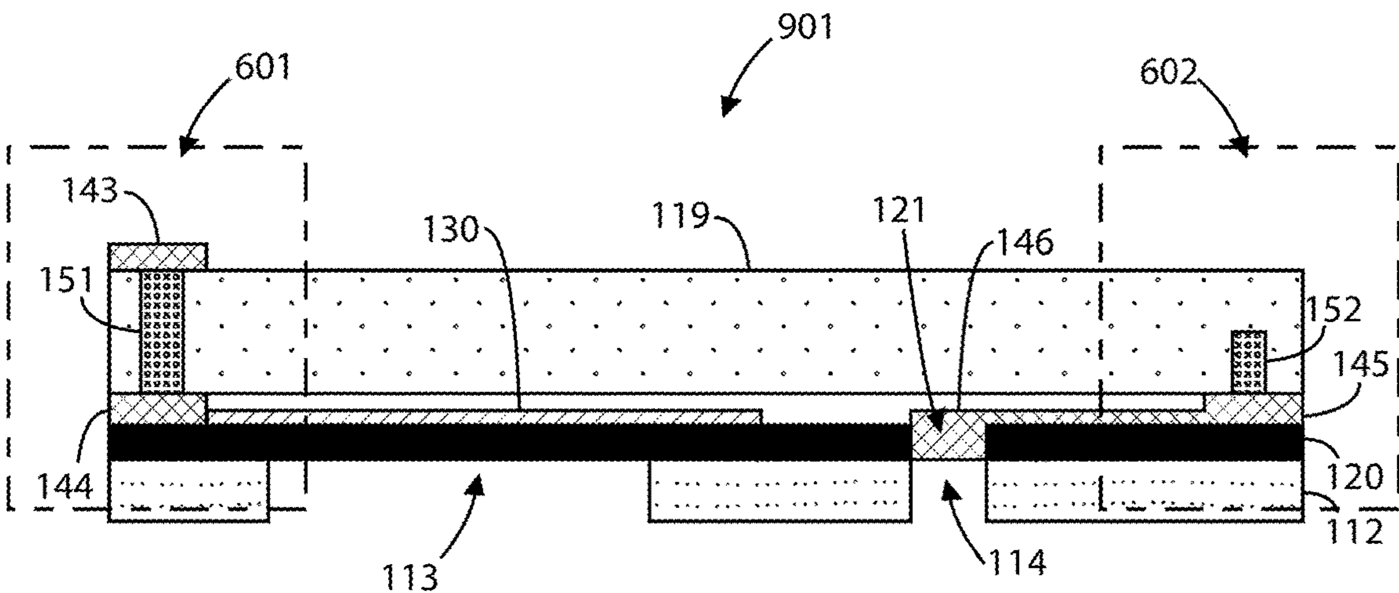
FIG. 9A
