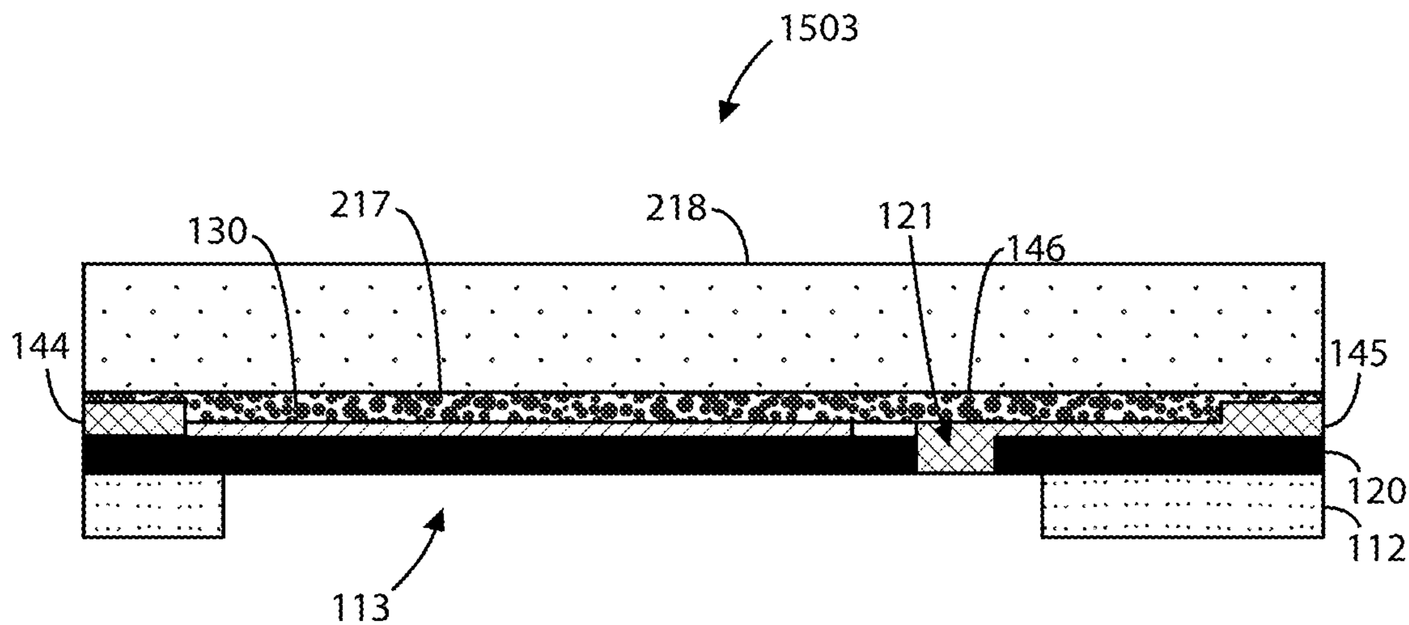
FIG. 15C
