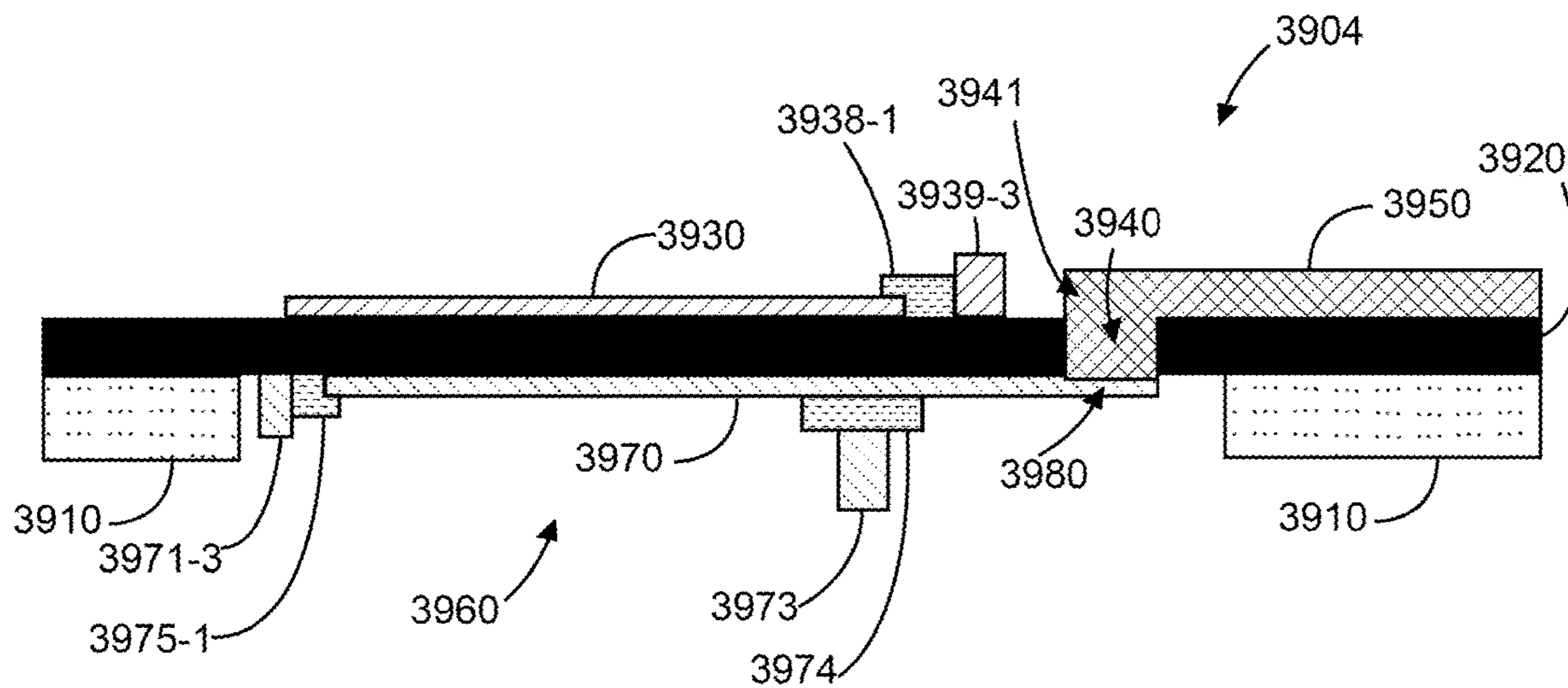
FIG. 39D
