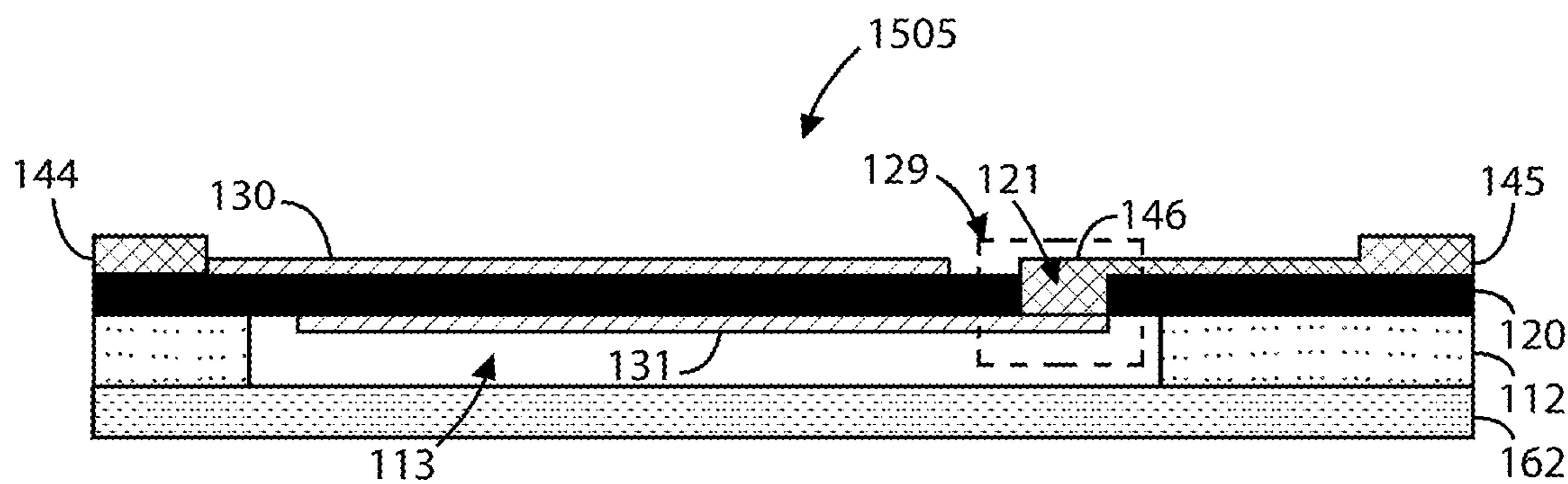
FIG. 15E
