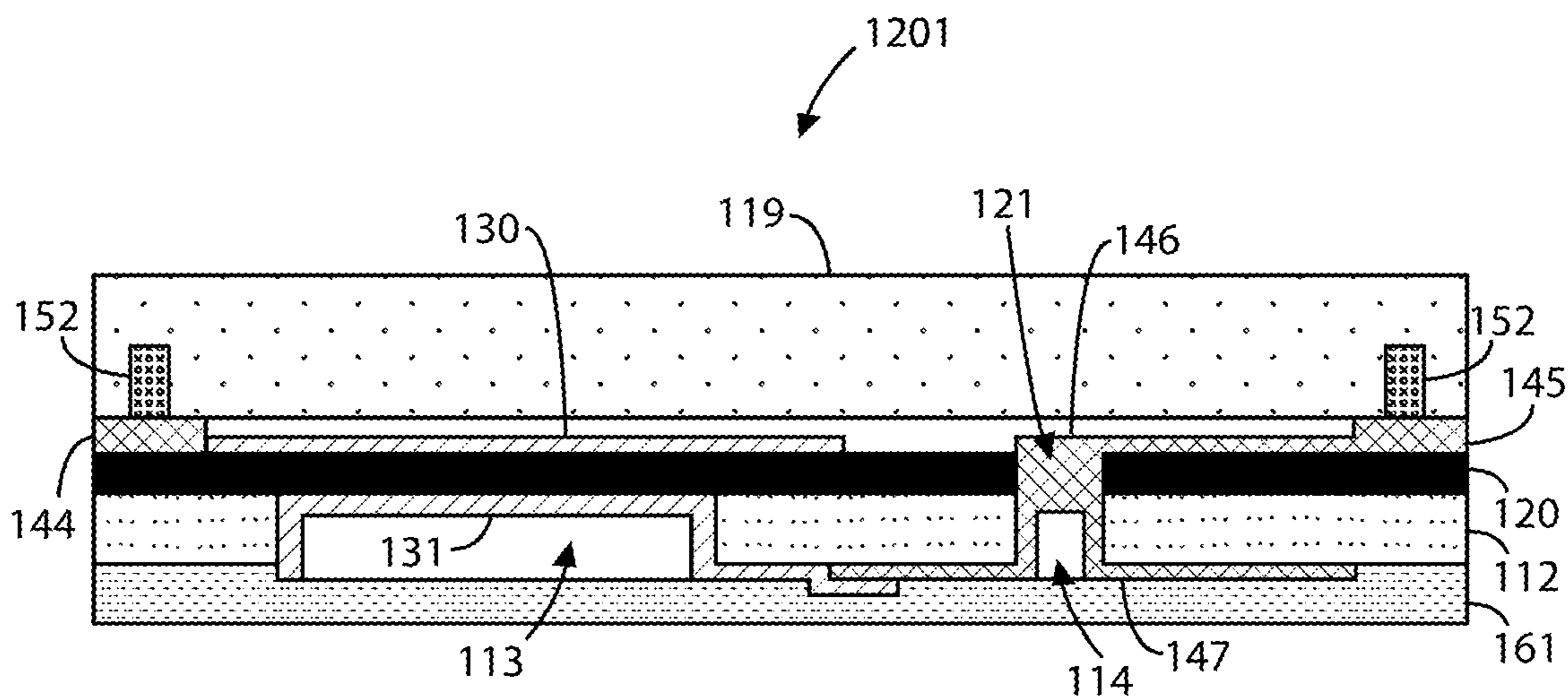
FIG.12A
