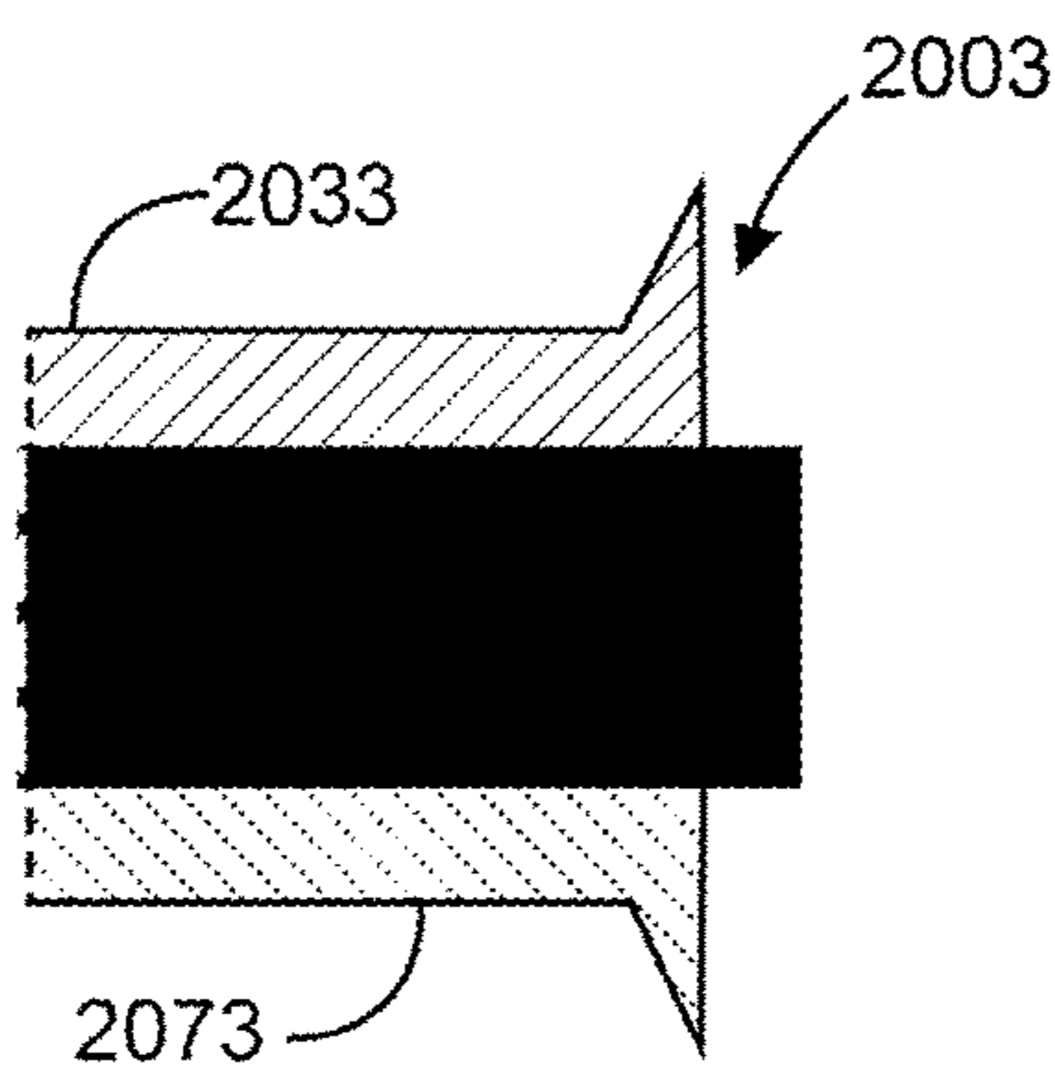
FIG. 20A
