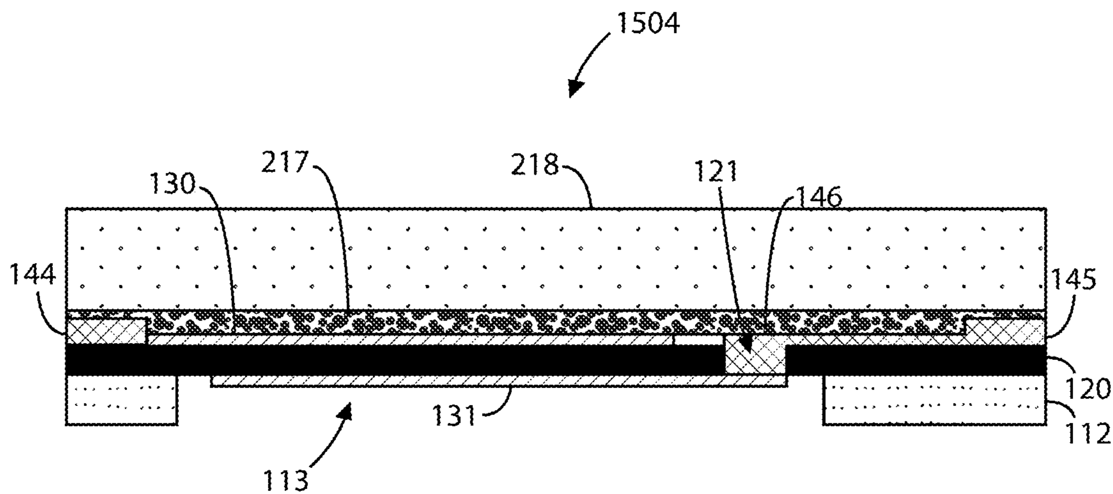
FIG. 15D
