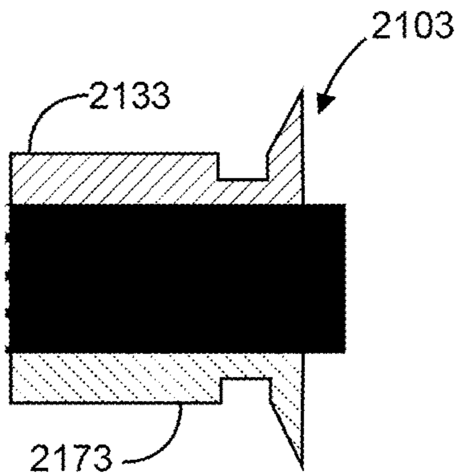
FIG. 21A
