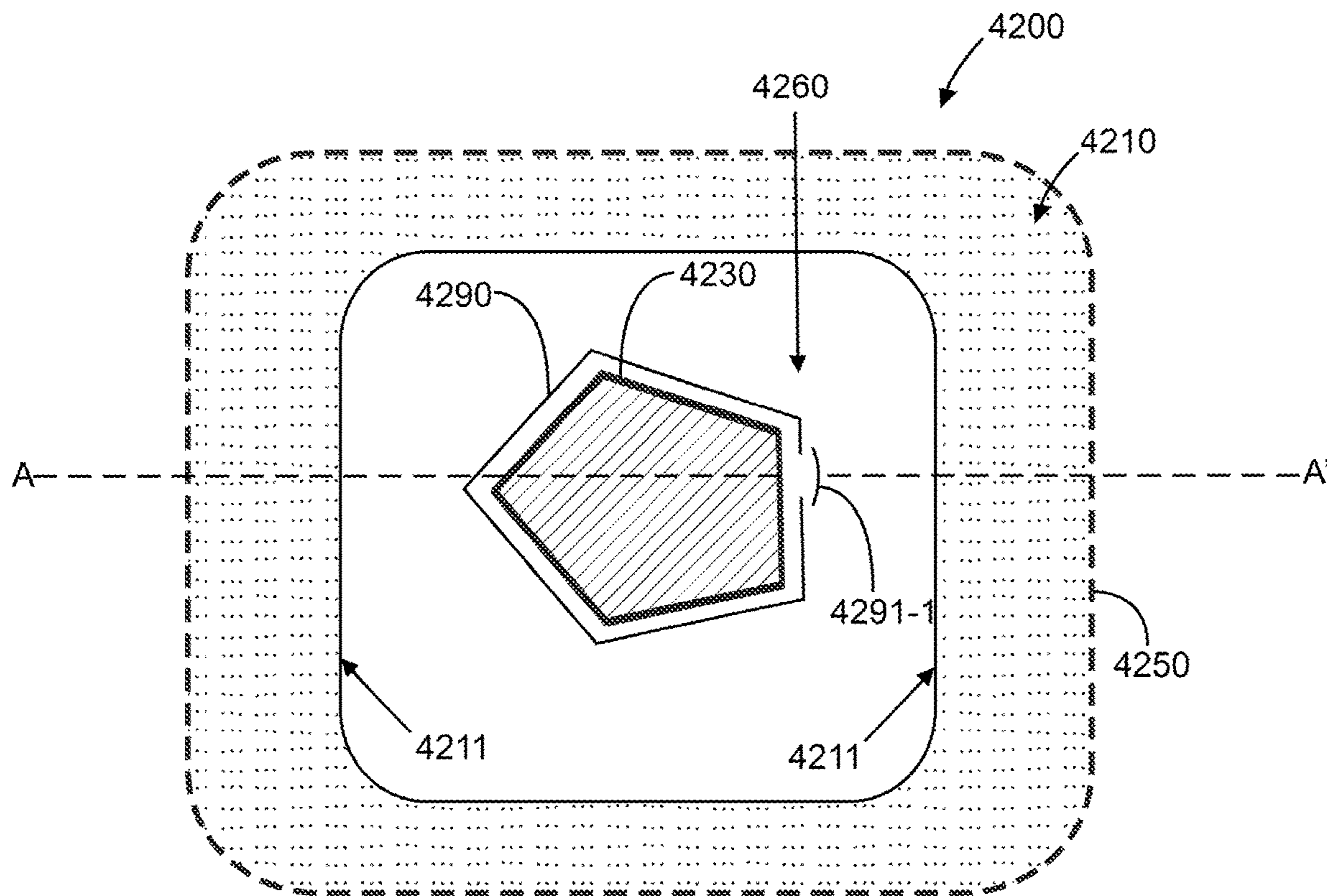
FIG. 42
