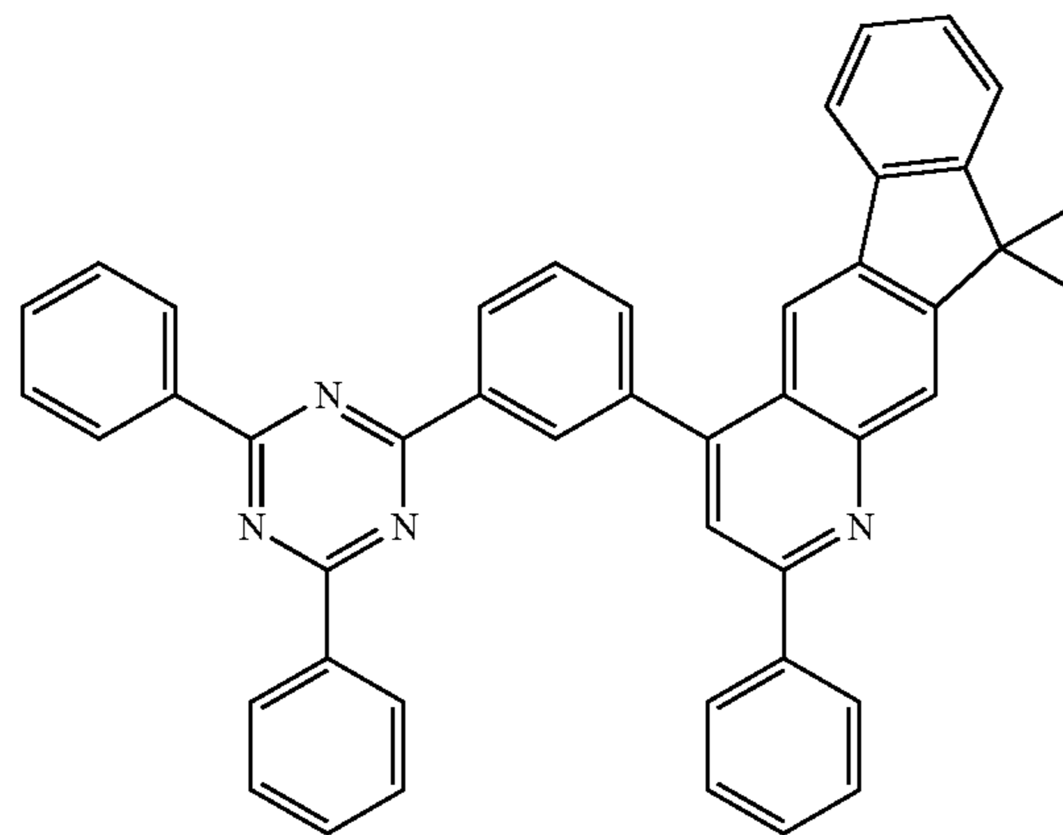
C-1
