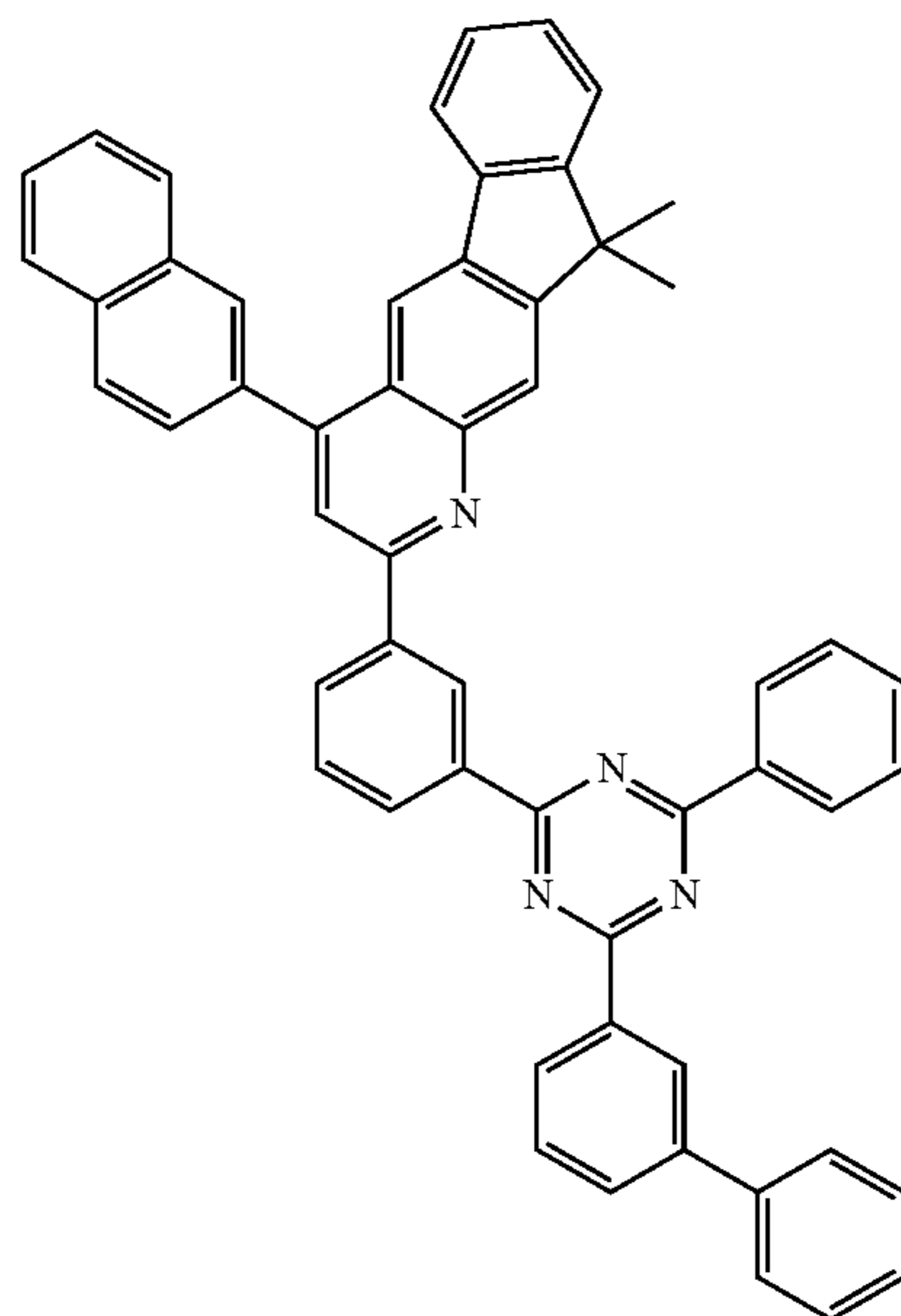
C-322
