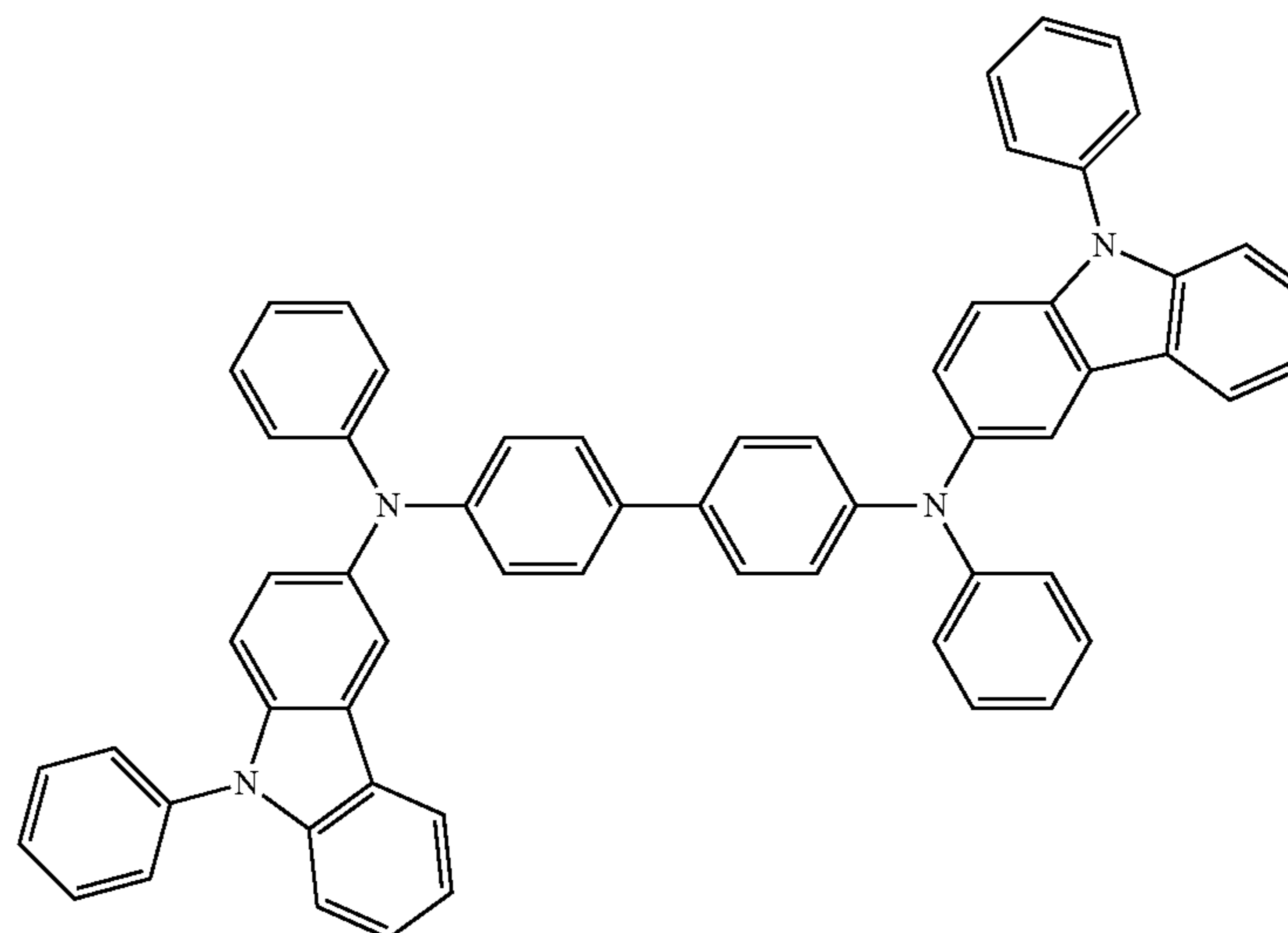
HI-1
