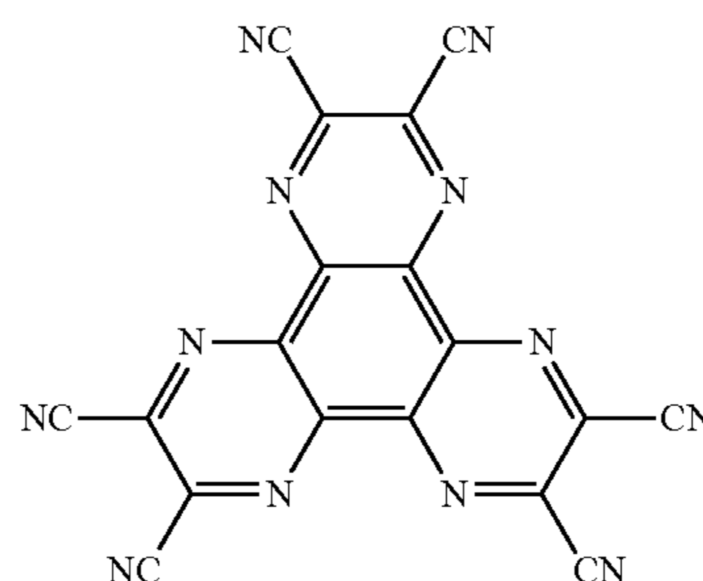
HI-2
