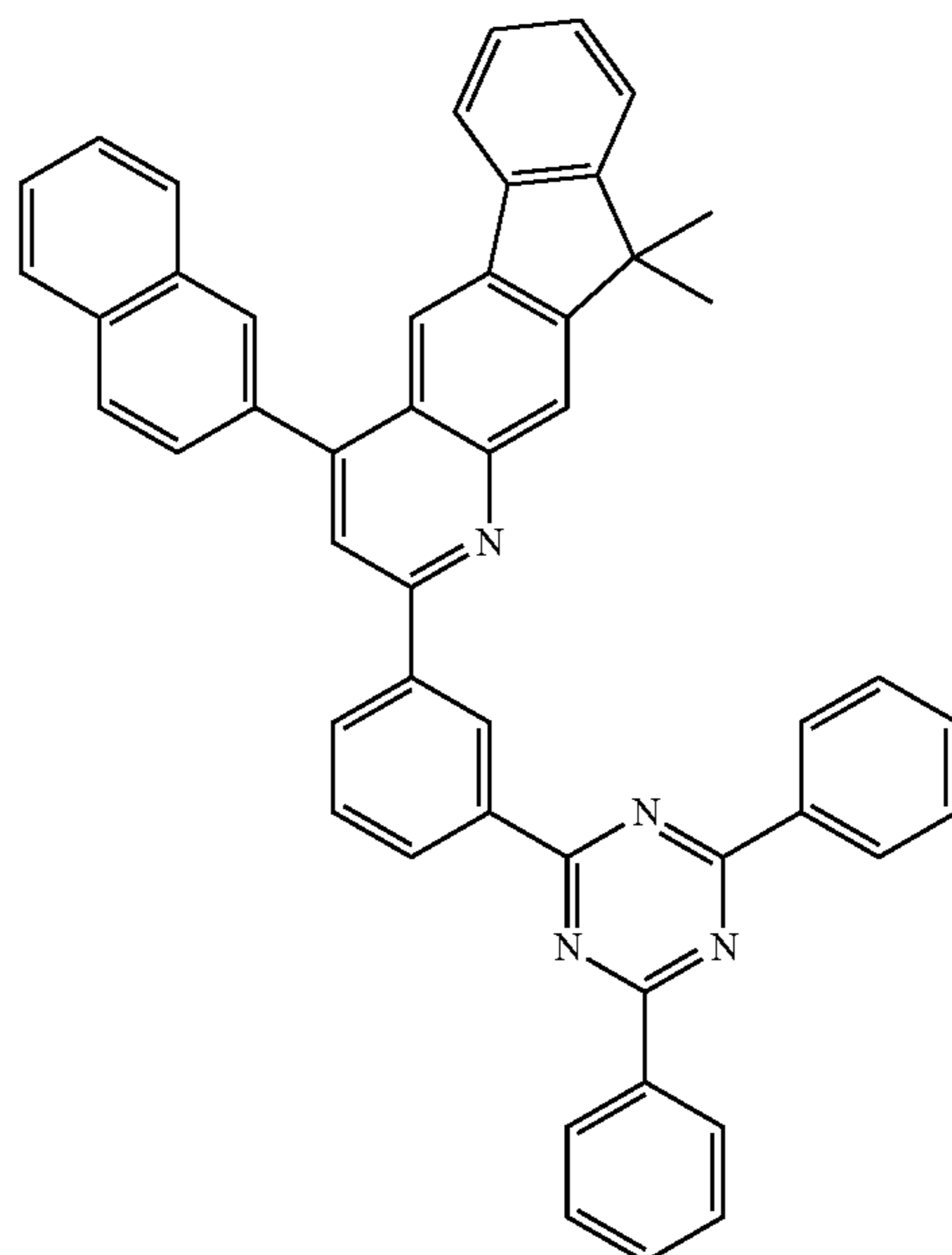
C-119
