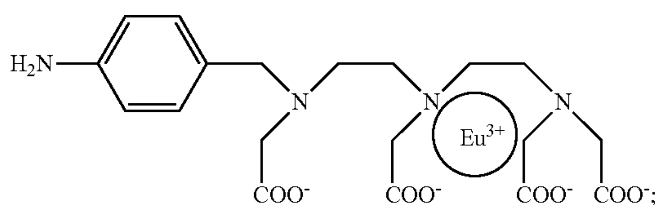
Europium-N1-amino (Eu-N1-amino)
