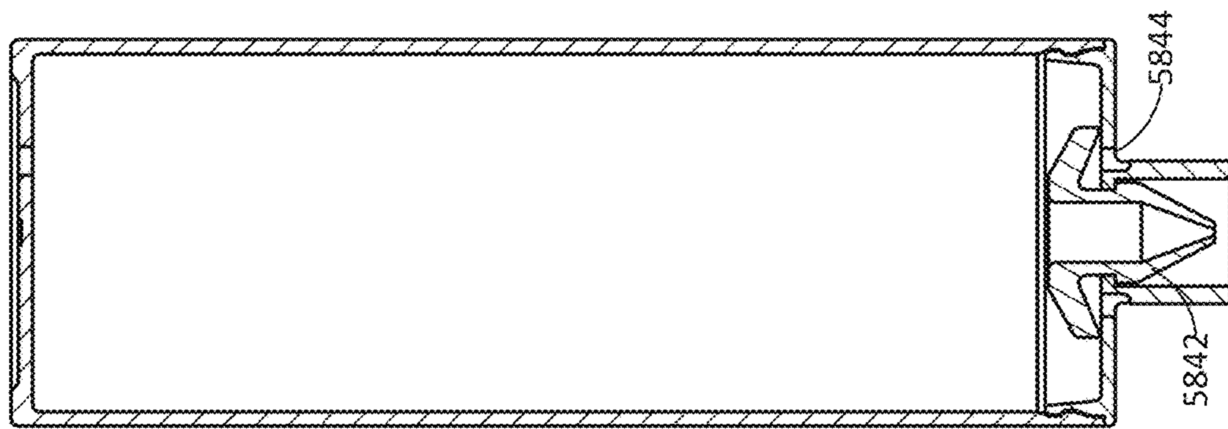
FIG. 58D
