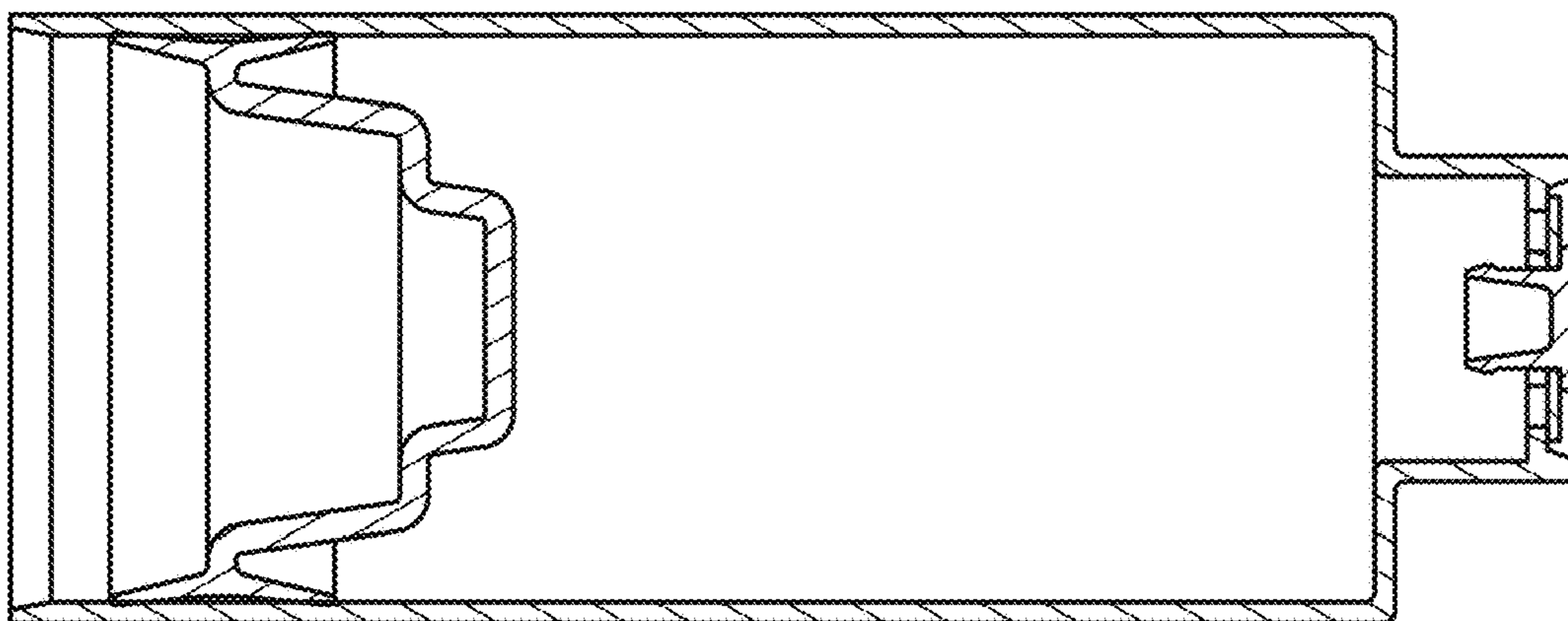
FIG. 58A
