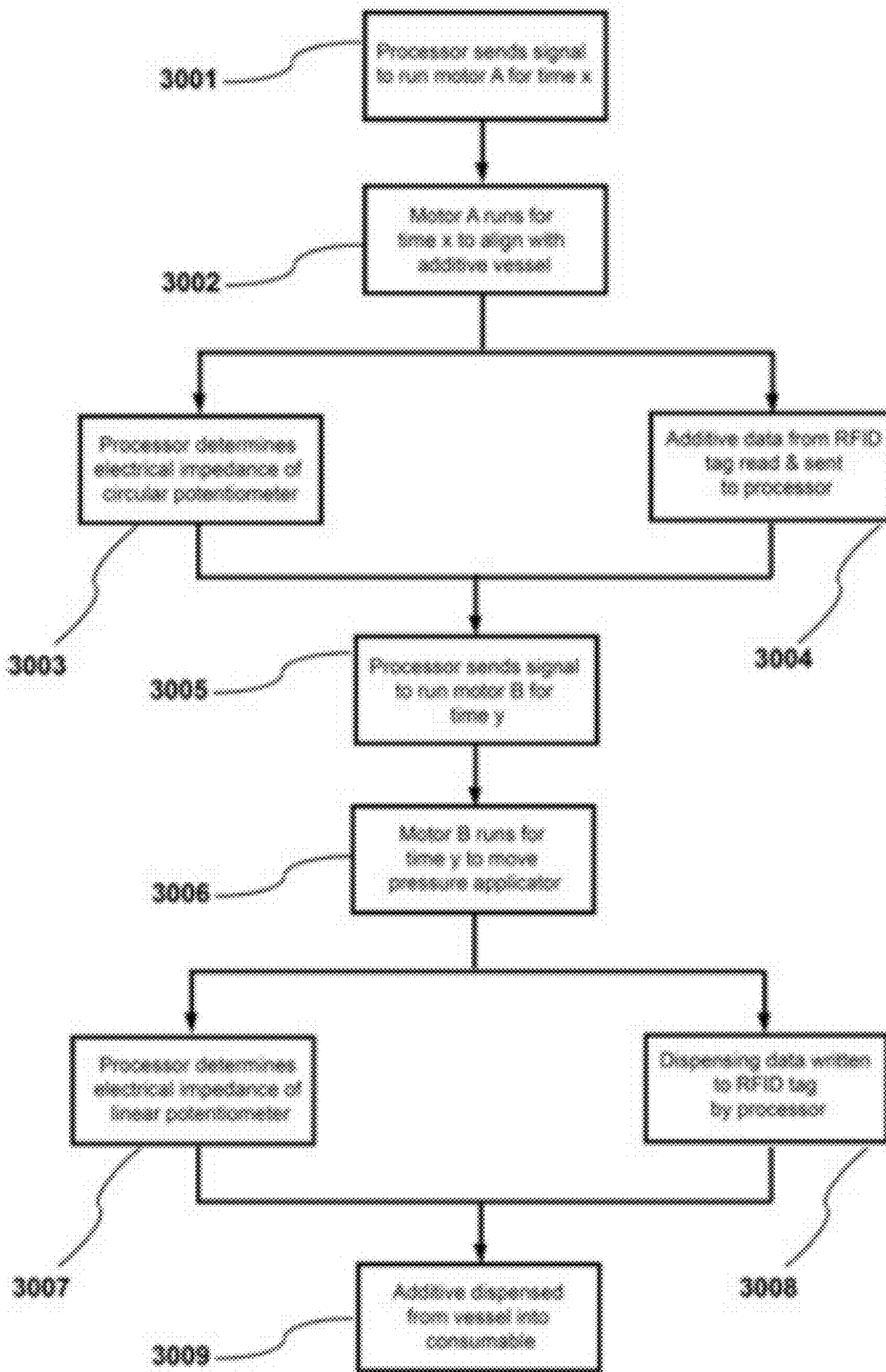
FIG. 30
