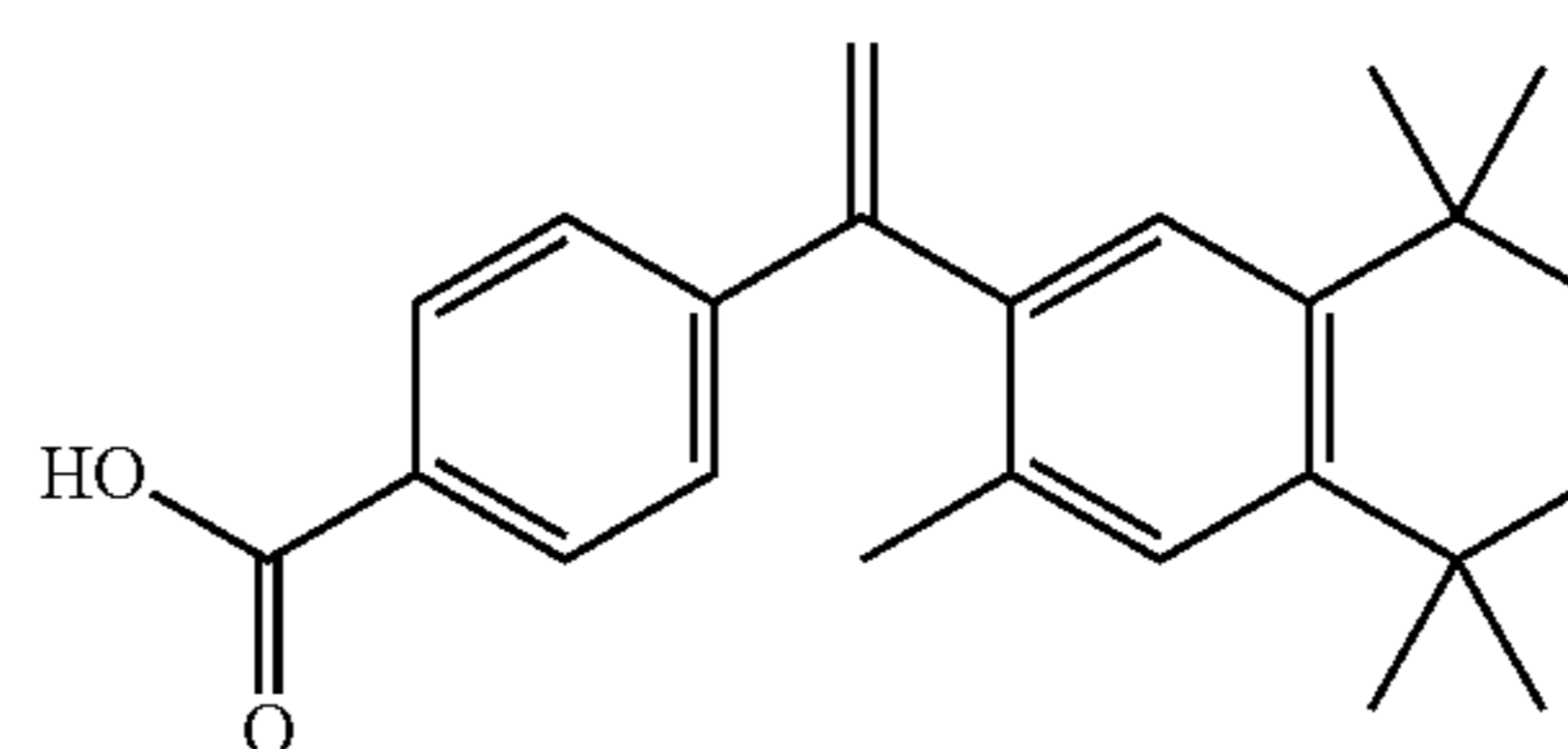
Bexarotene
