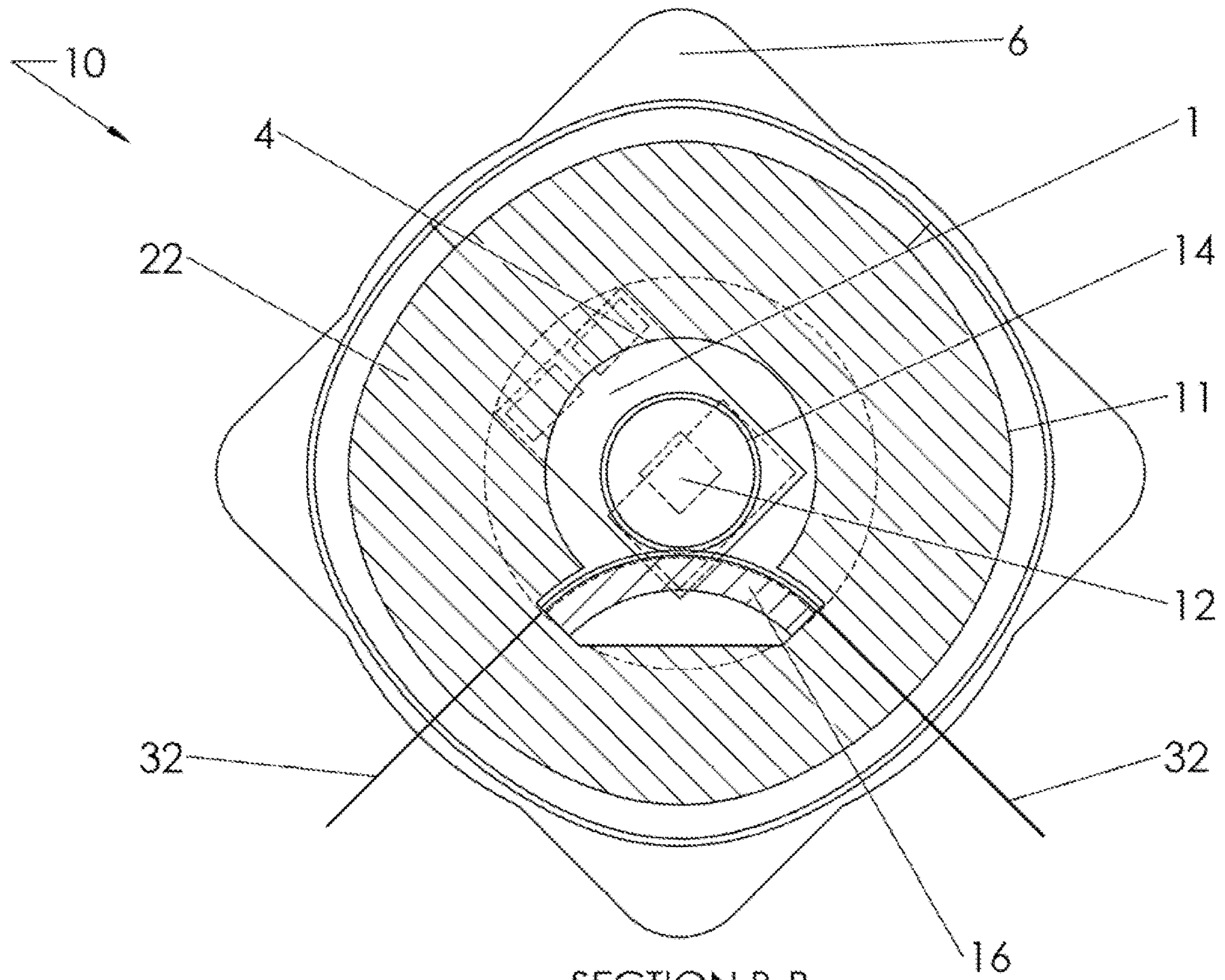
SECTION B-B FIG. 11a
