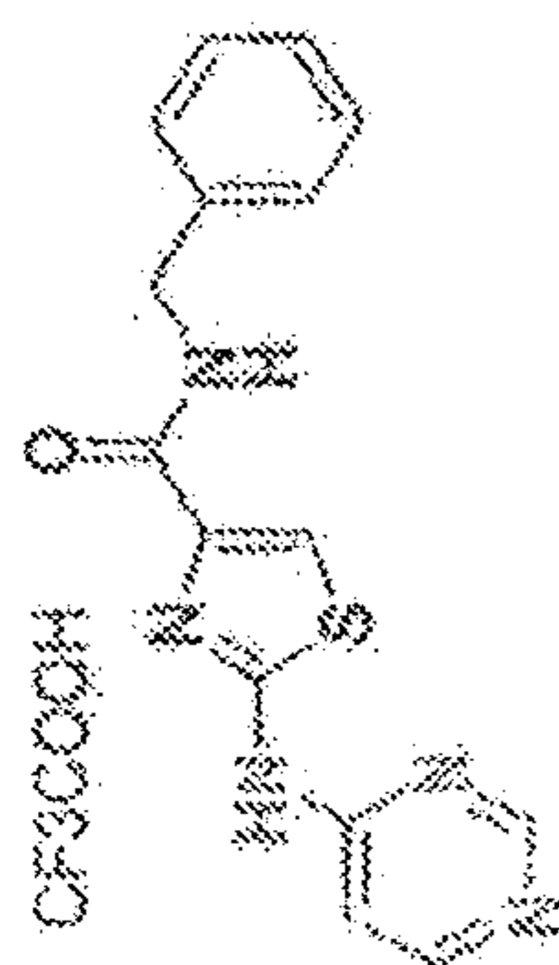
HHS-378 (Thiazovivin/Tzv)
