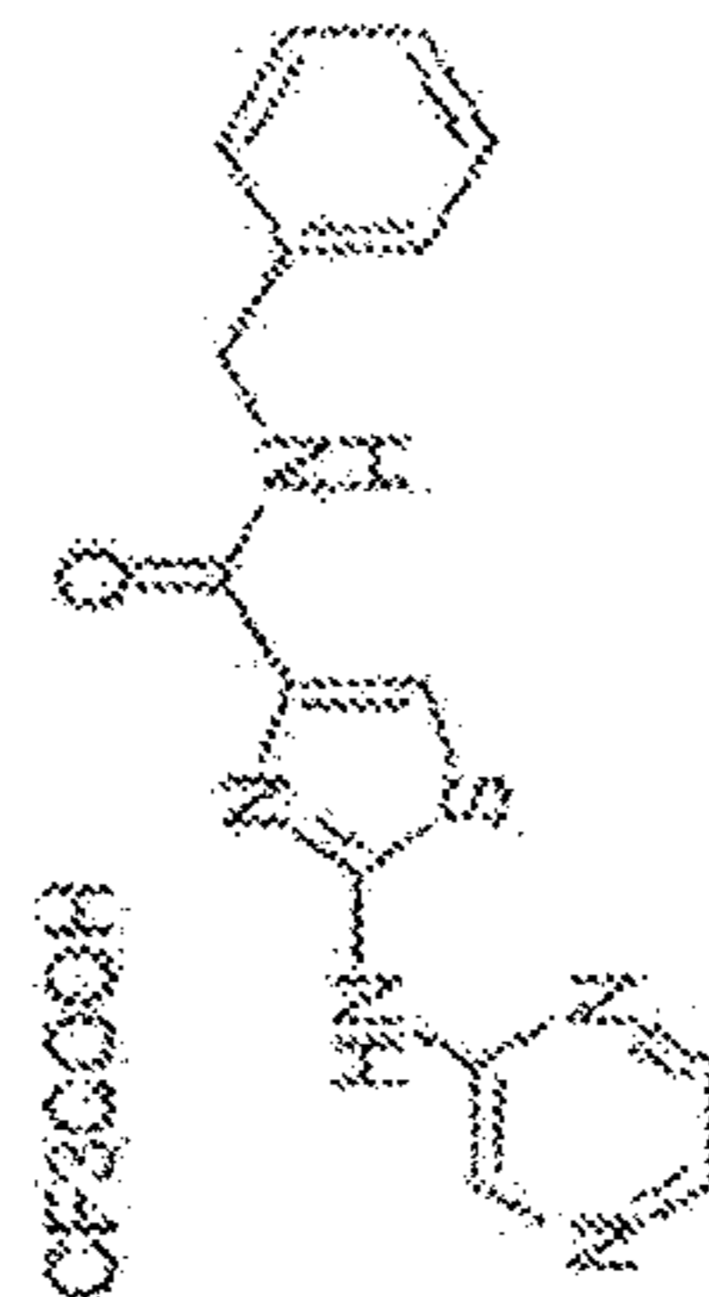
HHS-378-5
