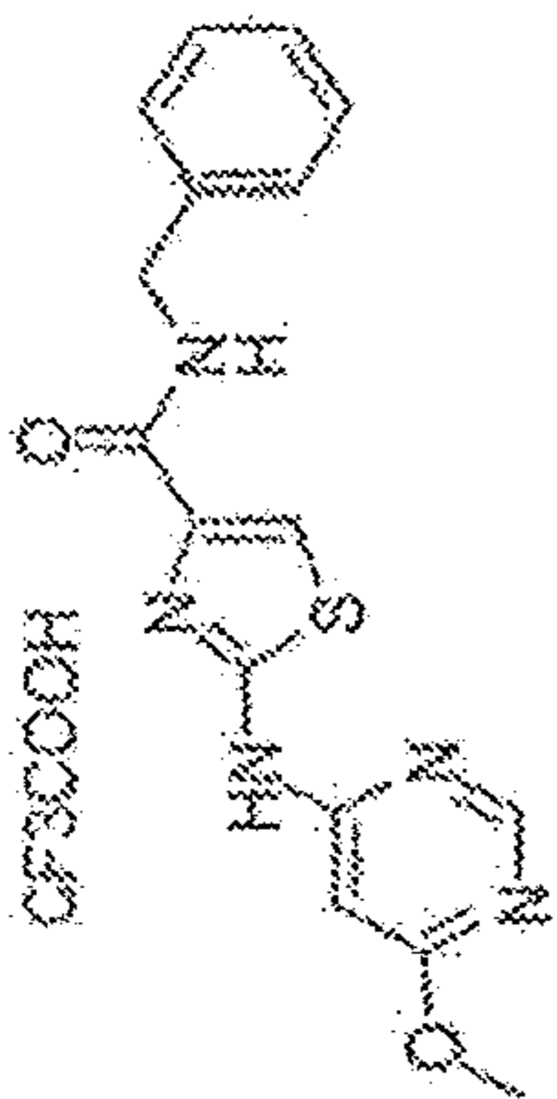
HHS-378-1
