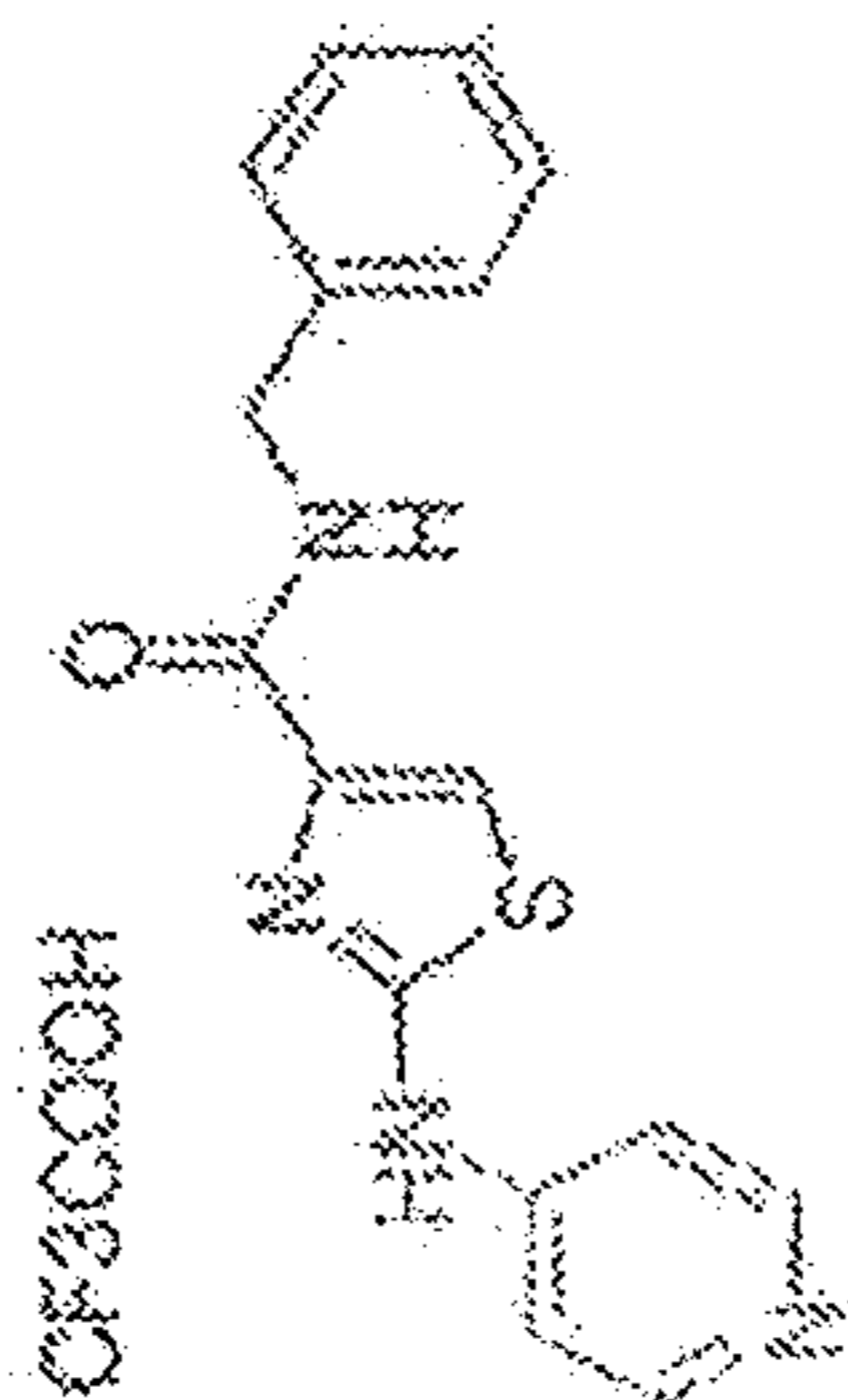
HHS-378-4
