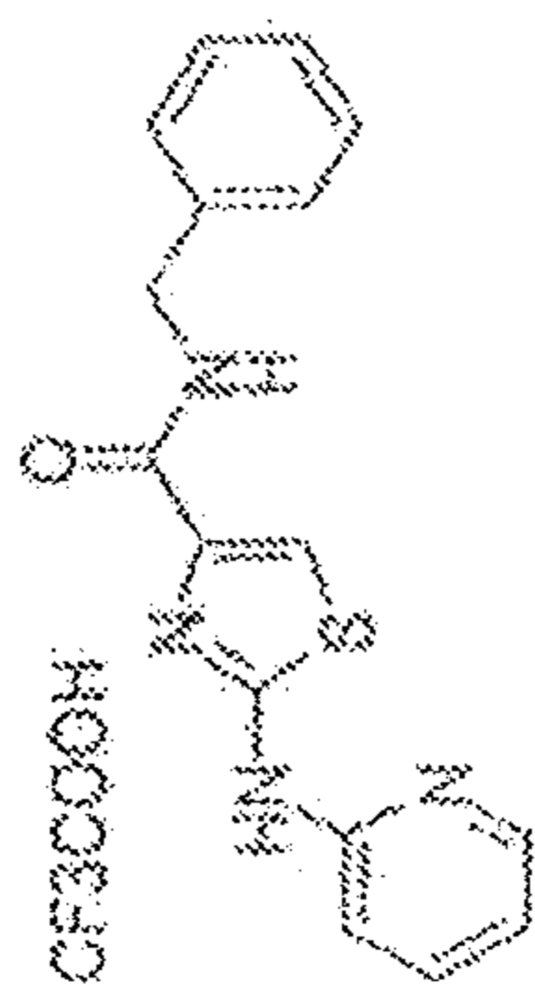
HHS-378-3
