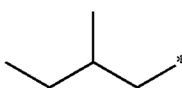
2-methylbutyl
