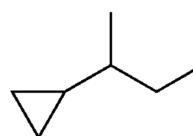
2-cyclopropylpropyl
