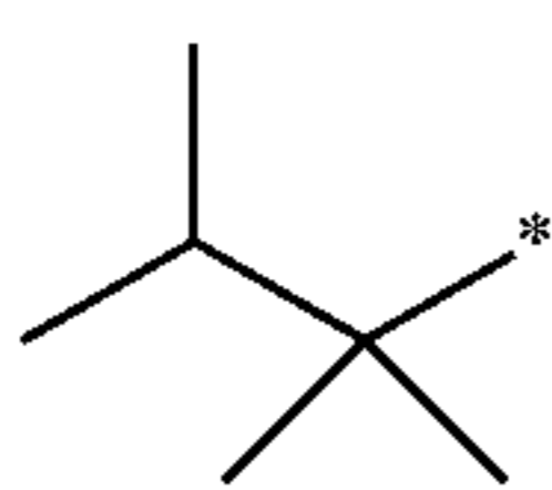
2,3-dimethylbutan-2-yl
