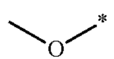
methoxy
