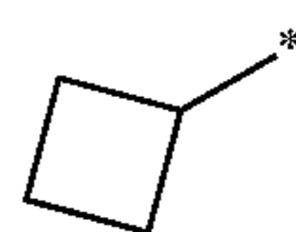
cyclobutyl
