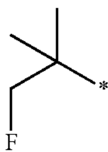
1-fluoro-2-methylpropan-2-yl
