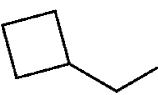
cyclobutylmethyl
