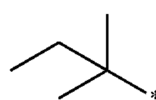
2-methylbut-2-yl
