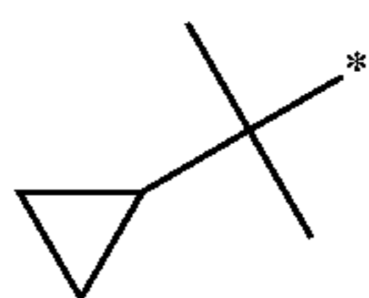
2-cyclopropylpropan-2-yl
