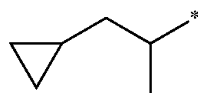
1-cyclopropylpropan-2-yl
