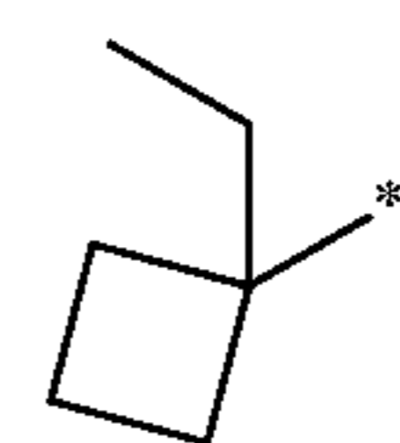
1-ethylcyclobutyl
