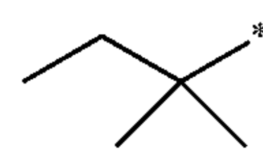
2-methylbut-2-yl
