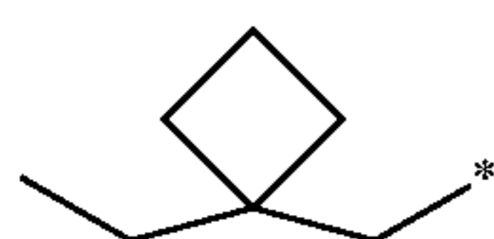
1-ethylcyclobutylmethyl
