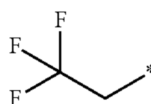
2,2,2-trifluoroethyl
