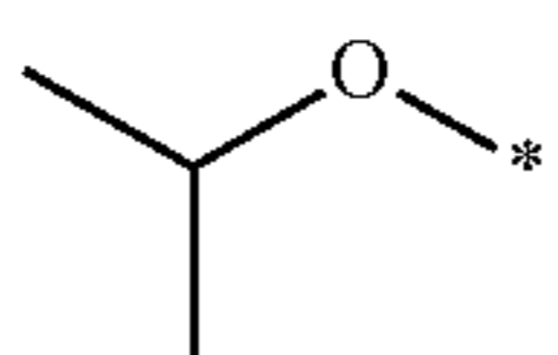
isopropoxy
