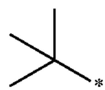
tert-butyl
