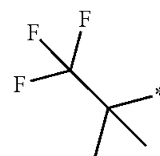
1,1,1-trifluoro-2-methylpropan-2-yl
