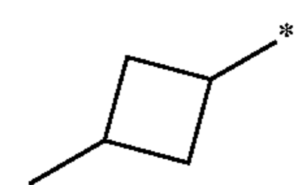
3-methylcyclobutyl
